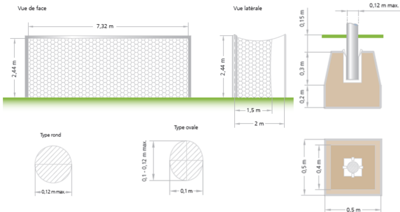
Figure 159 : détails de but
