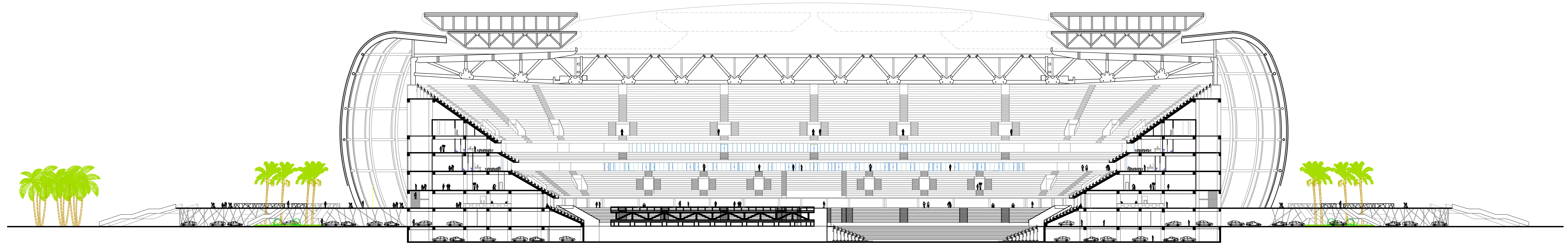
Coupe B-B
