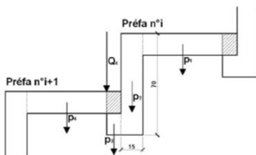
Figure 87 : Section résistante à la torsion
