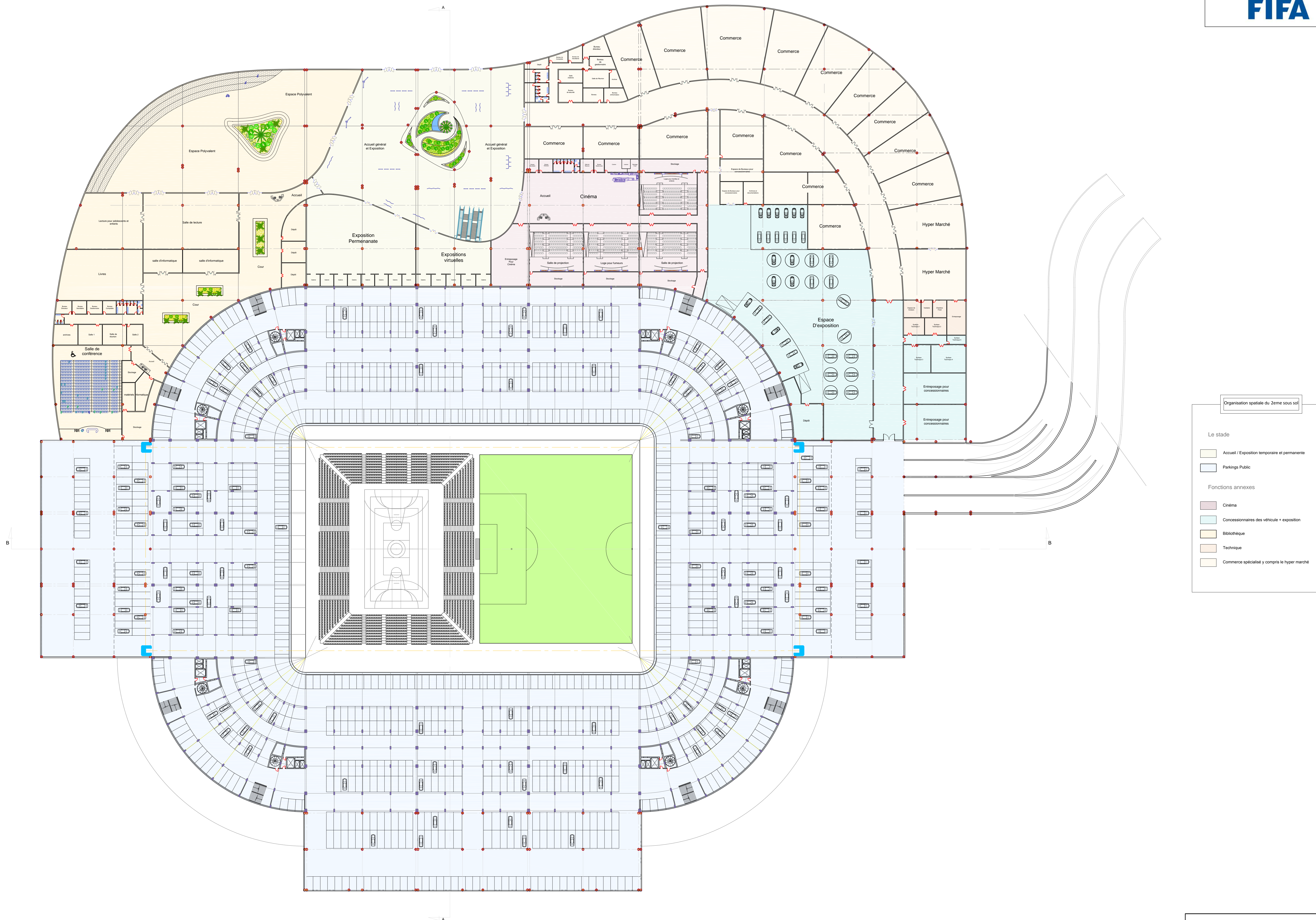
Plan du 2 eme sous-sol
