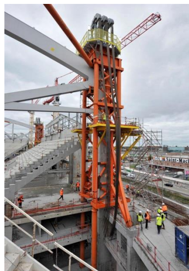
Figure 97: tour métallique temporaire Autour d'un méga poteau
