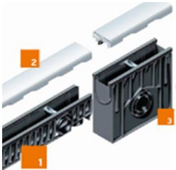
Figure 157 : les composants d'un réseau de drainage
