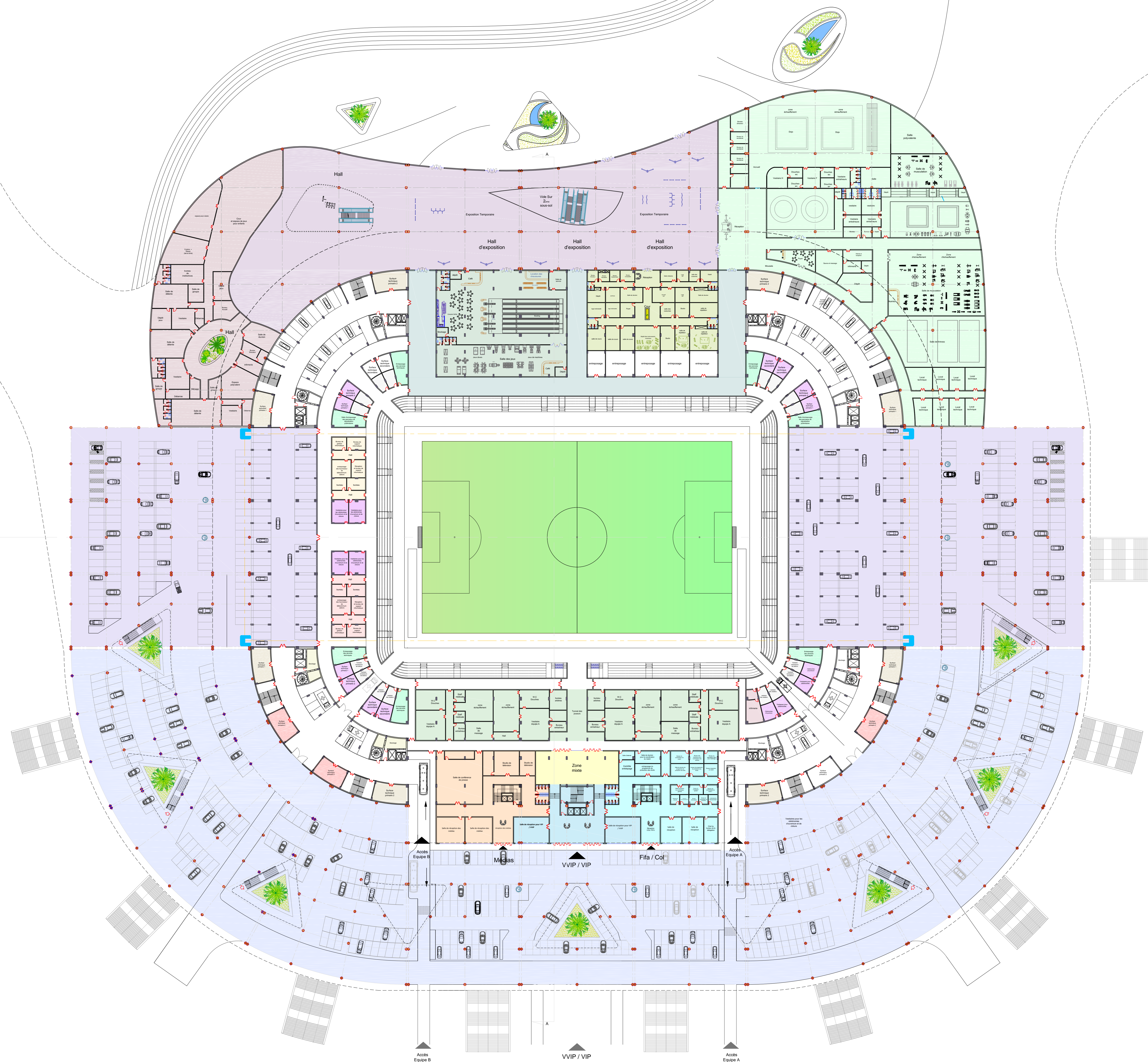
Plan du 1er sous-sol
