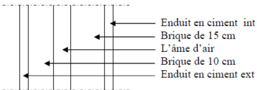
Figure II.5 Coupe transversale du mur extérieur
