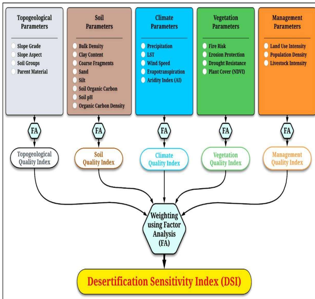
Figure 11: Desertification Sensitivity Index (Kouba, 2023) par Ahmed Alliouche et Yacine Kouba
