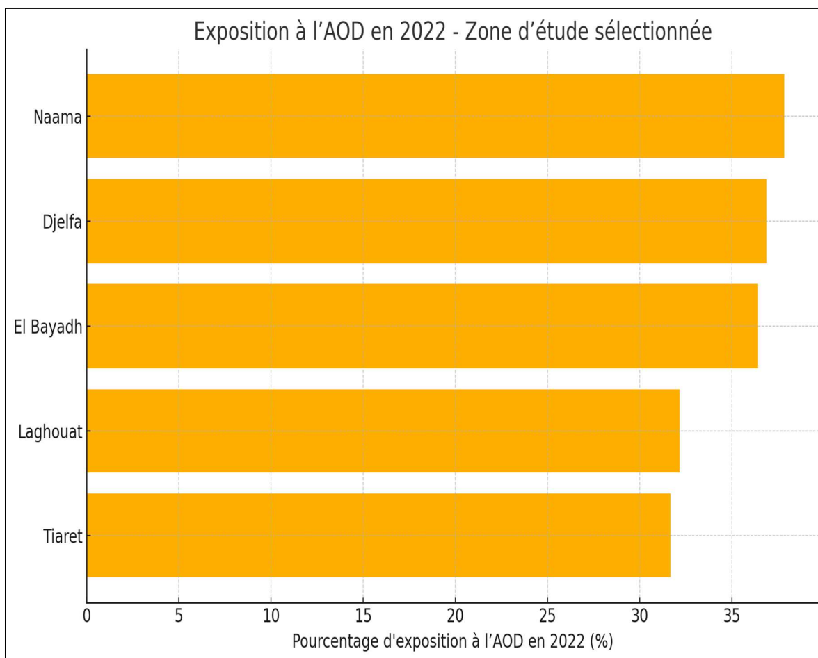
Figure 47: Classement des wilayas de votre zone d'étude selon le pourcentage d'exposition à l'AOD en 2022
