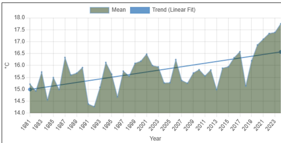
Figure 40: Analyse de la température moyenne de l'air en surface (annuelle) dans la wilaya de Tiaret (1981-2023)
