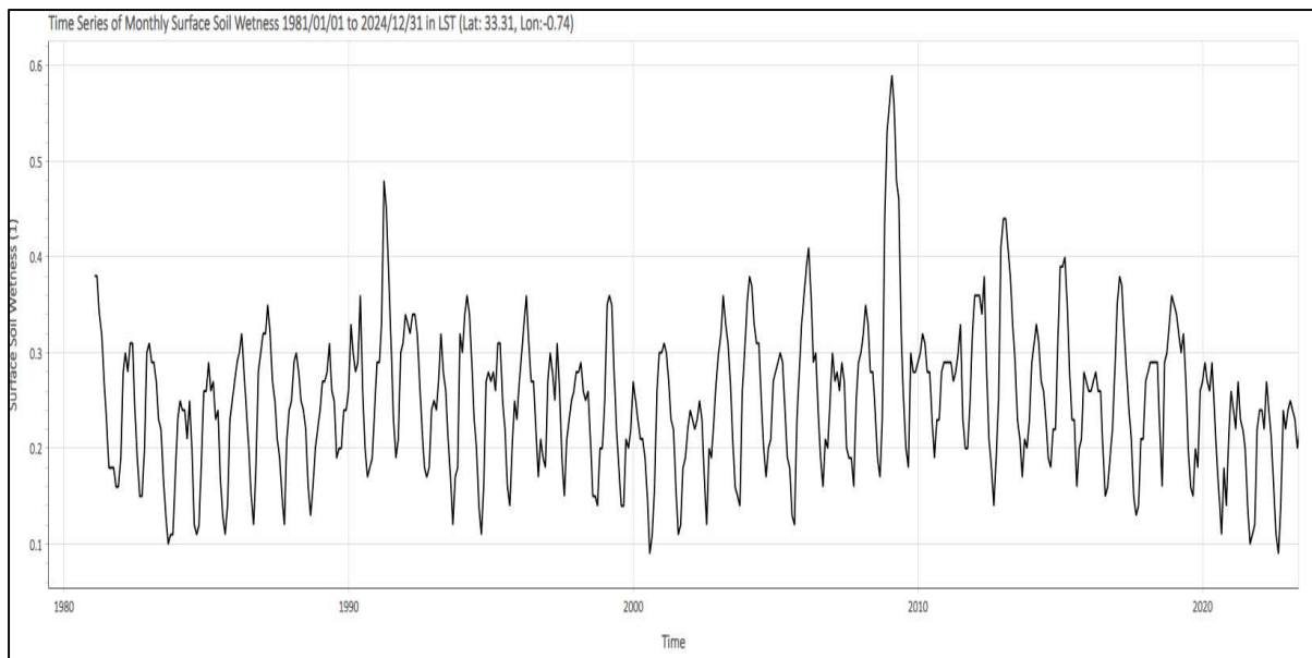
Figure 41: Humidité de surface du sol de la zone d'étude
