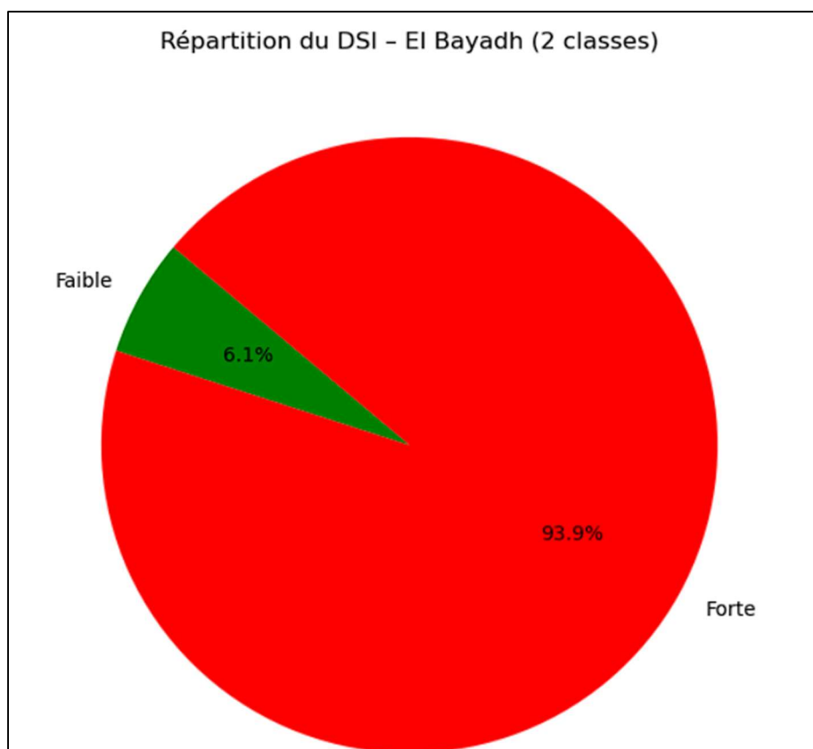
Figure 51: Répartition du DSI pie chart Elbayadh
