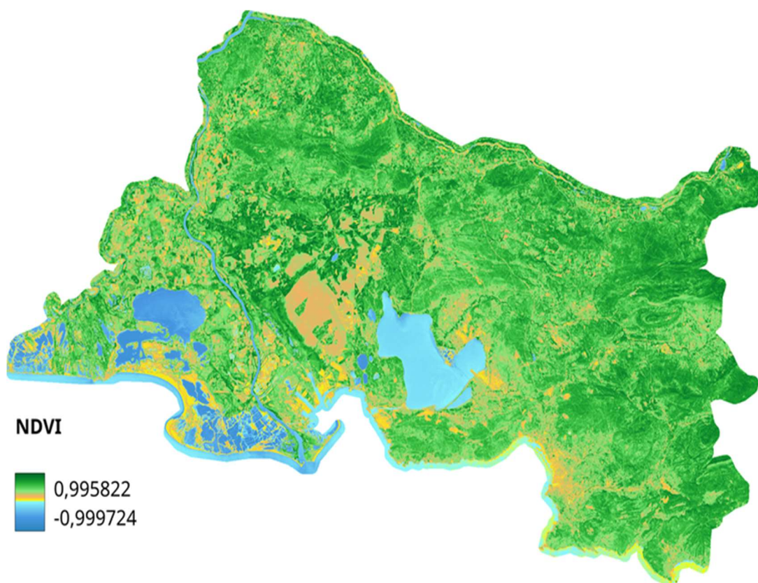
Figure 3: Exemple NDVI des Bouches-du-Rhône pour le 13 juin 2019 Image en ligne (R1)
