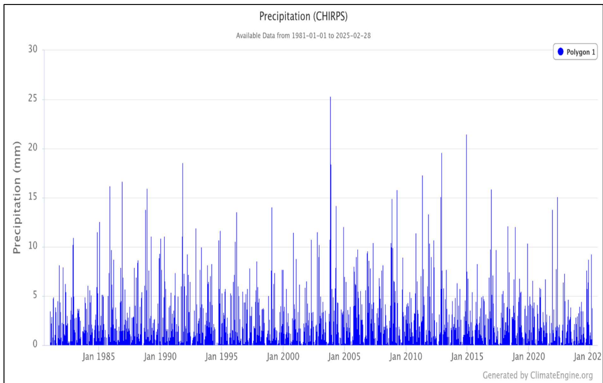
Figure 32: Analyse de la précipitation dans la wilaya El Bayedh (1981-2025)
