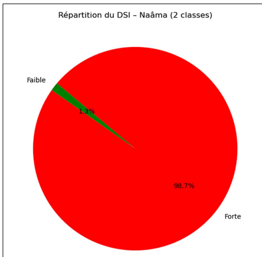
Figure 55: Répartition du DSI Pie chart Naama
