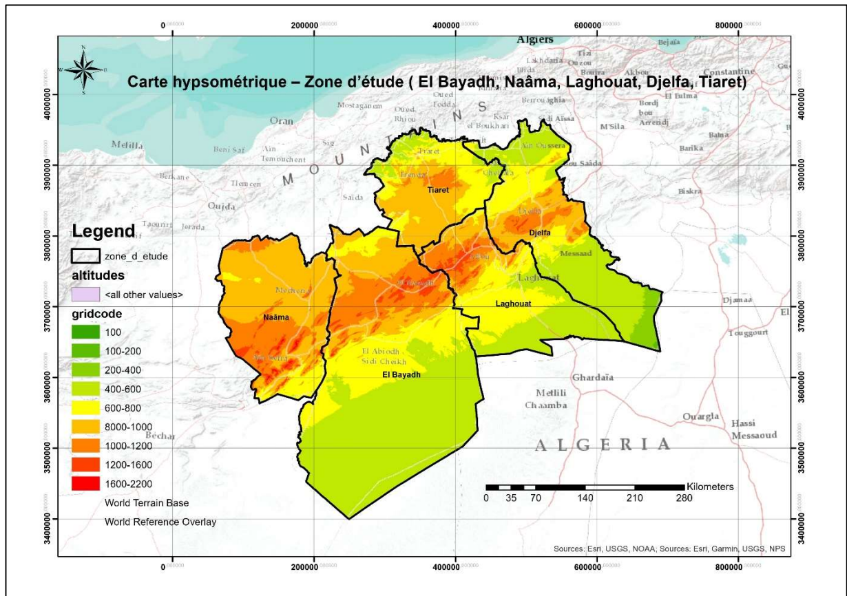
Figure 26: Carte hypsométrique de la zone d'étude
