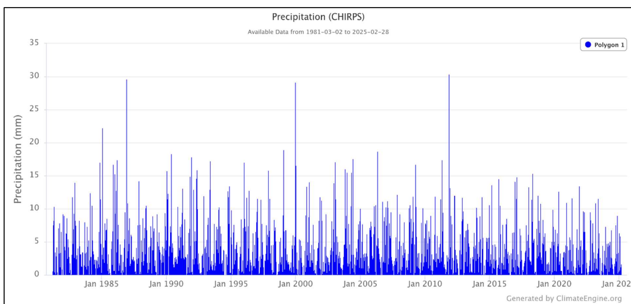
Figure 34: Analyse de la précipitation dans la wilaya de Djelfa (1981-2025)
