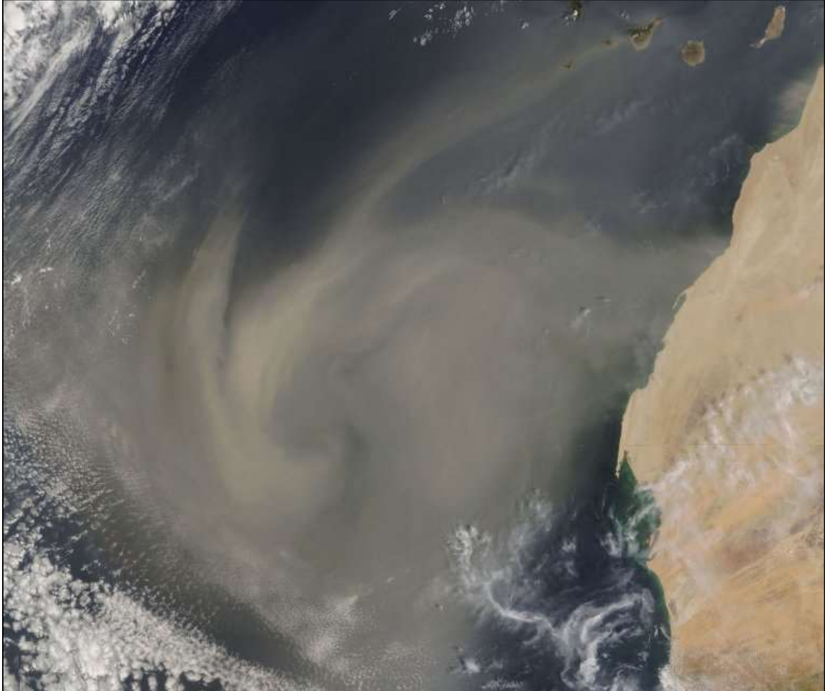
Figure 18: Tempête de sable vue de l'espace (source : NASA image).
