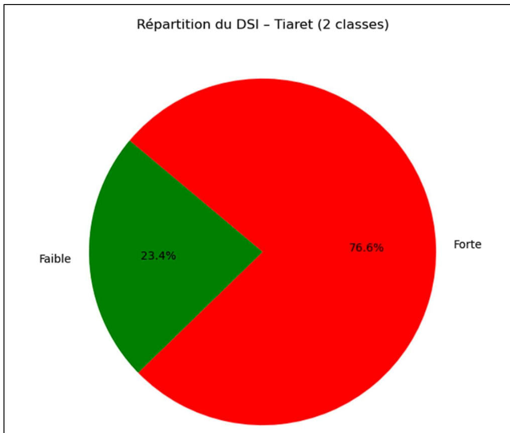
Figure 57: Répartition du DSI Pie chart Tiaret
