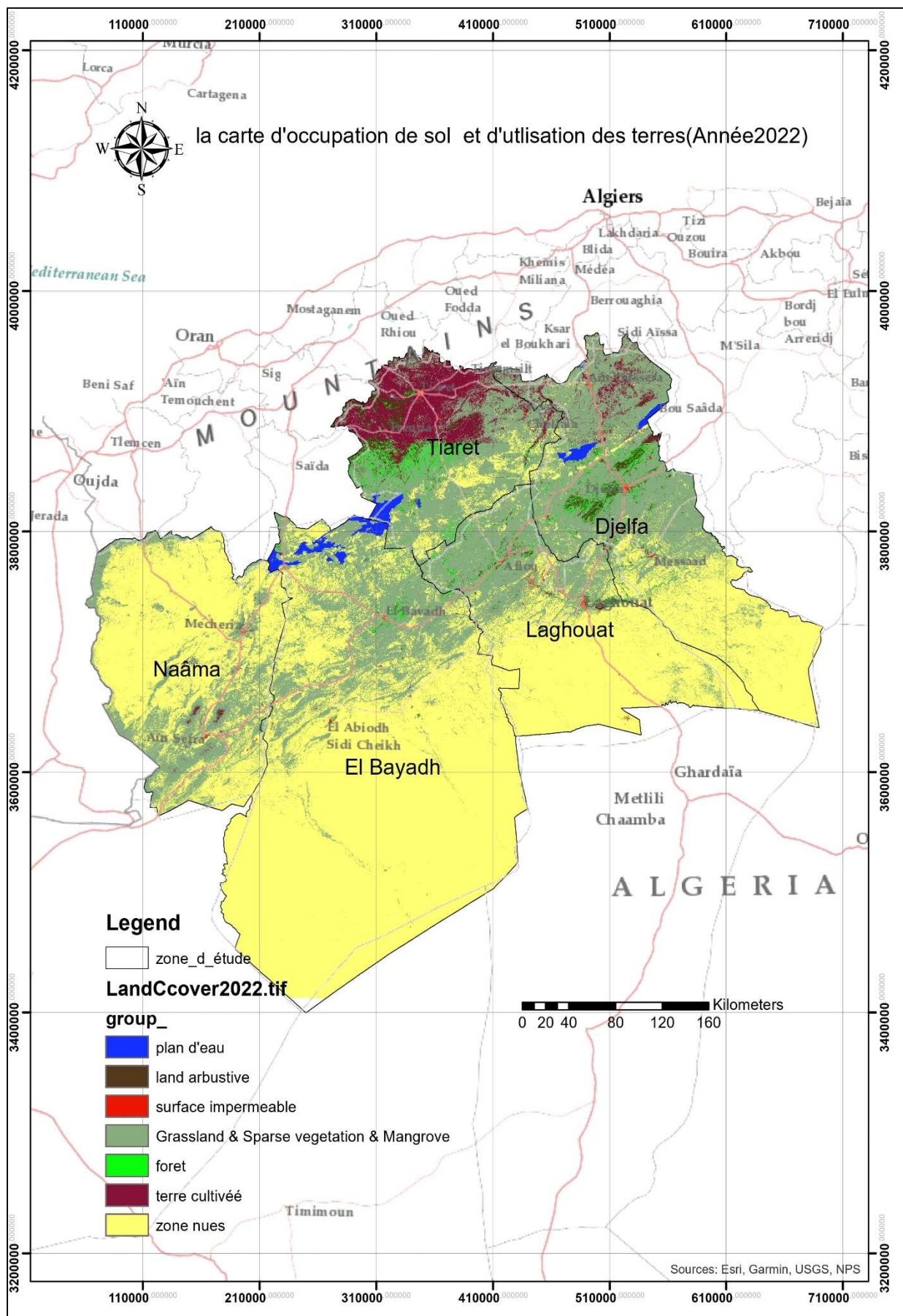
Figure 24: La carte d'occupation de sol (Année 2022)
