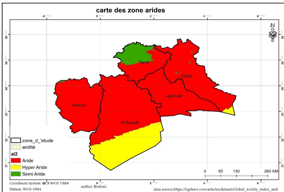
Figure 42: Carte des zones arides dans notre cas d'étude.
