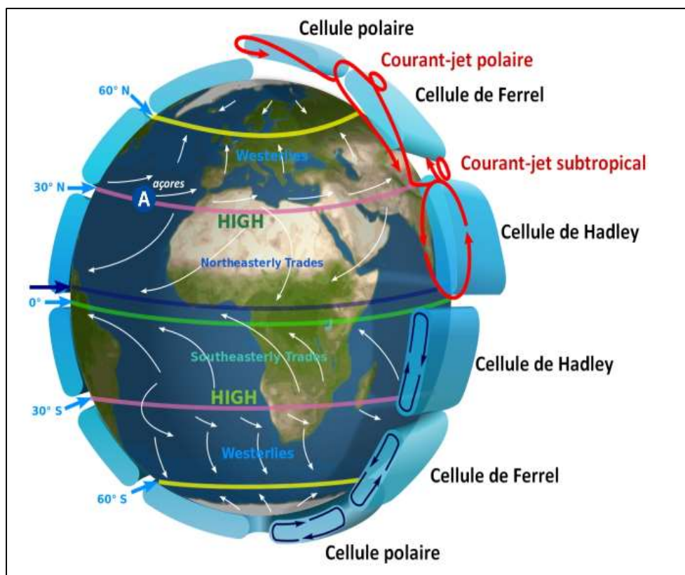
Figure 9: Schéma de la circulation atmosphérique globale sur Terre image de Kaidor via Libération
