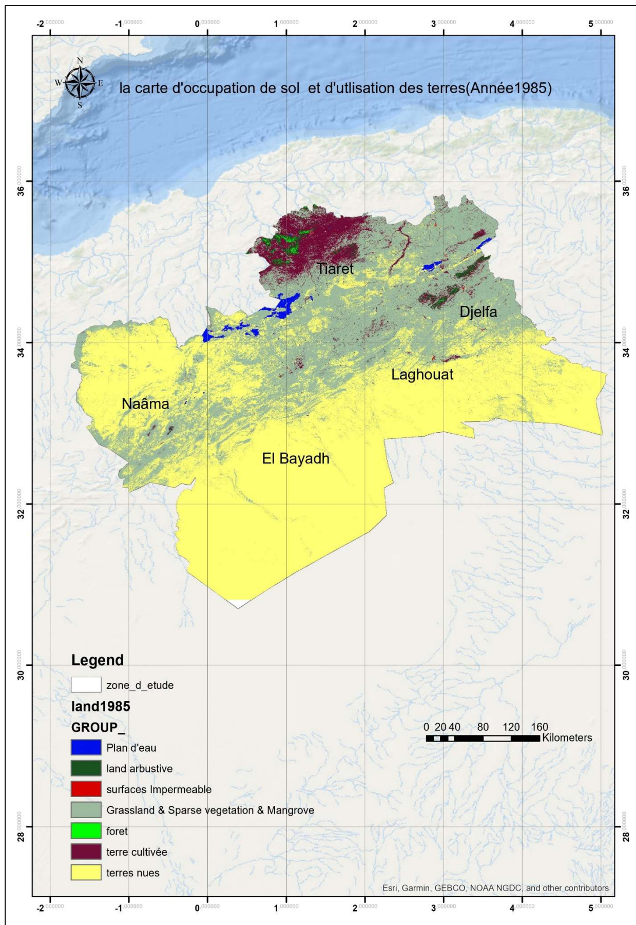
Figure 23: La carte d'occupation de sol (Année 1985)
