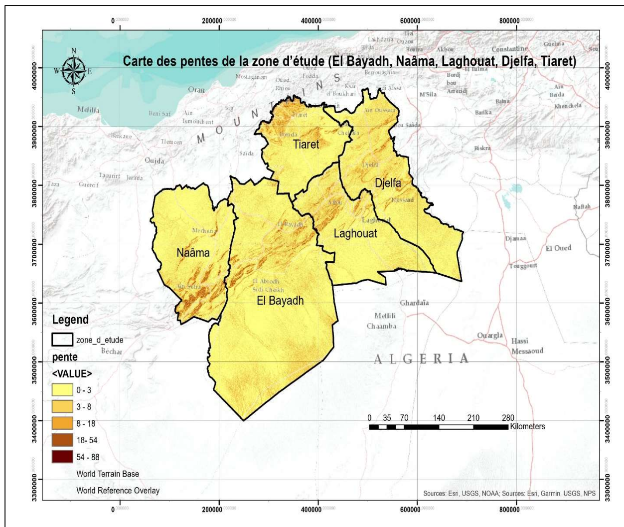
Figure 28: Carte des pentes de la zone d'étude
