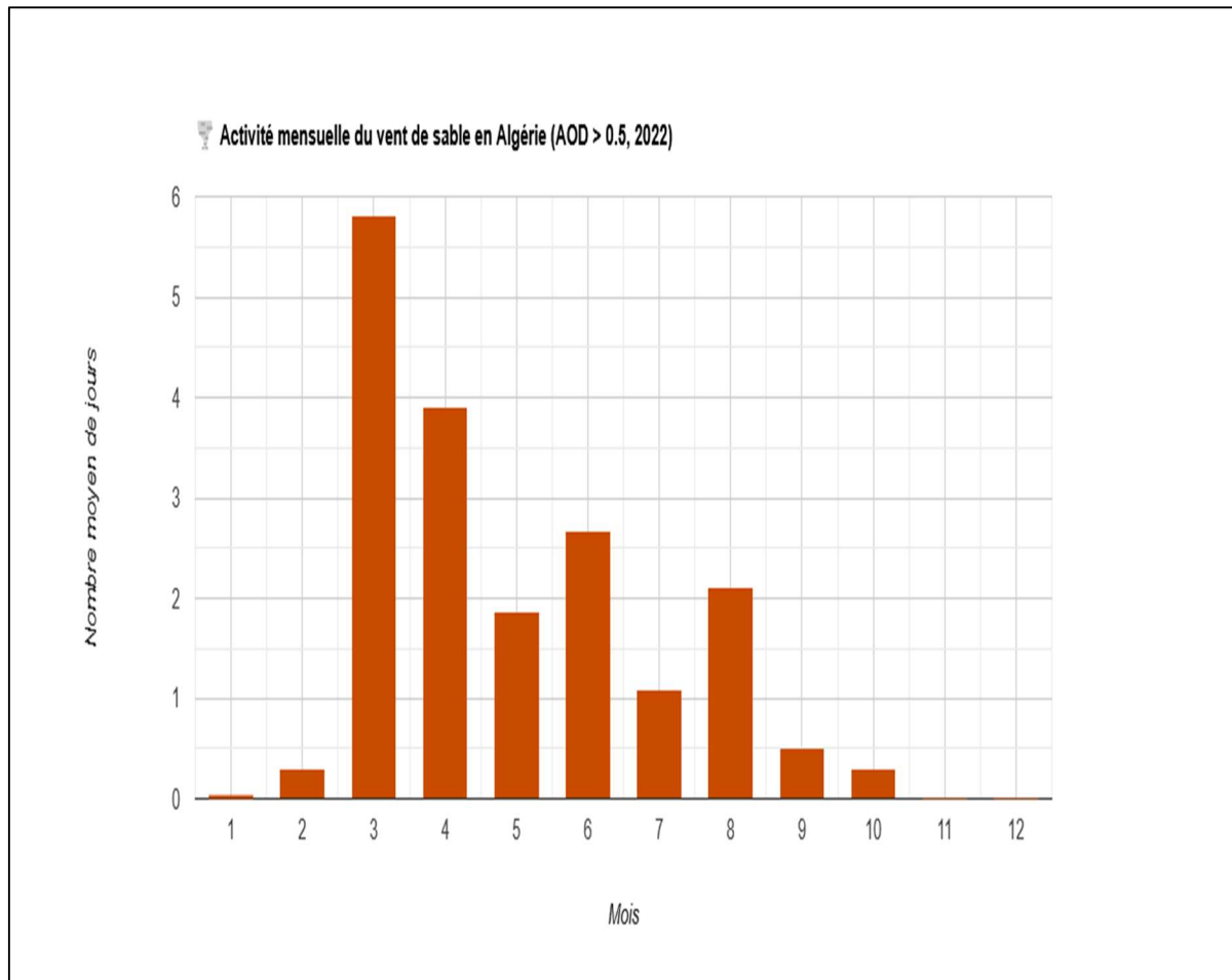
Figure 46: Le mois le plus poussiéreux en 2022
