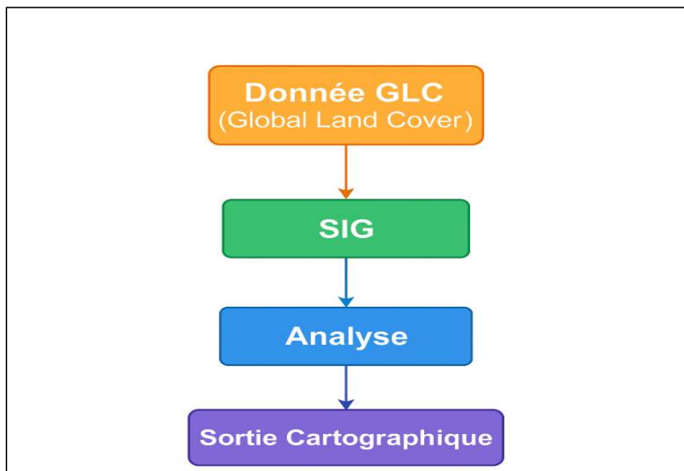
Figure 22: Méthodologie de réalisation d'une carte d'occupation de sol
