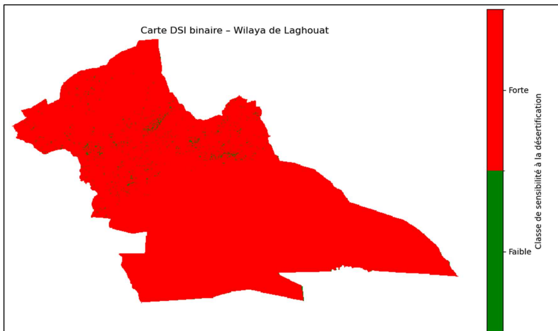
Figure 52: Carte DSI Wilaya Laghouat
