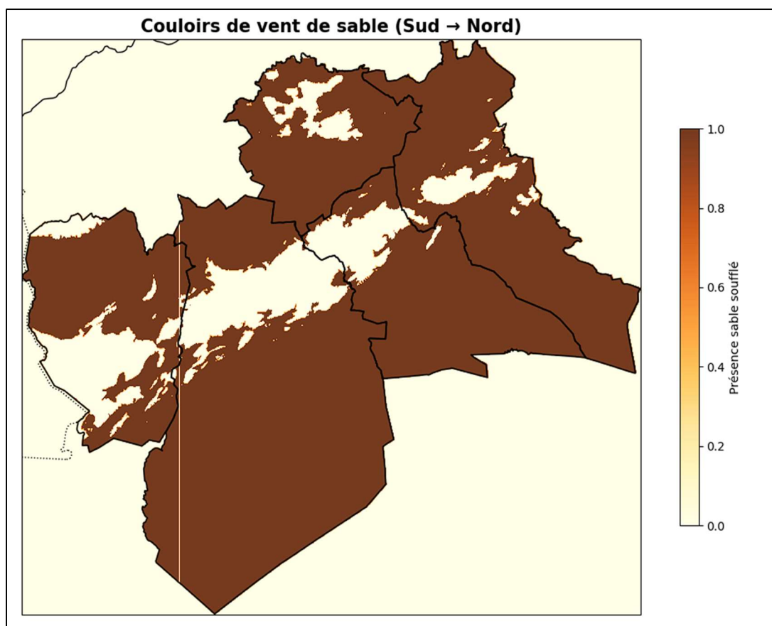
Figure 60: Couloire de vent de sable dans les Wilayas de la zone d'étude de gauche à droite Naama El-Bayadh Laghouat Tiaret et Djelfa
