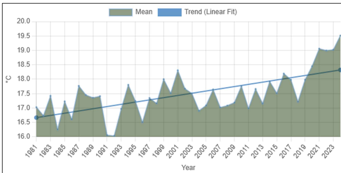
Figure 38: Analyse de la température moyenne de l'air en surface (annuelle) dans la wilaya de Djelfa (1981-2023)
