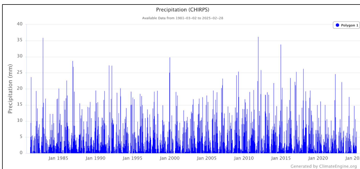
Figure 35: Analyse de la précipitation dans la wilaya de Tiaret (1981-2025)
