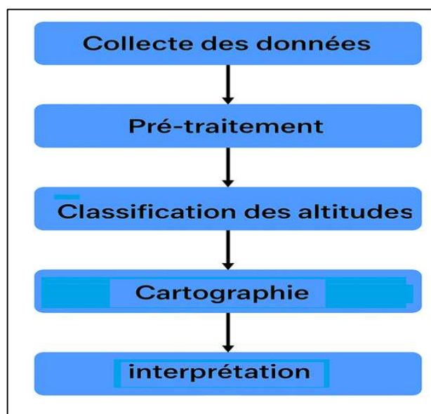
Figure 25: Méthodologie pour élaborer une carte hypsométrique
