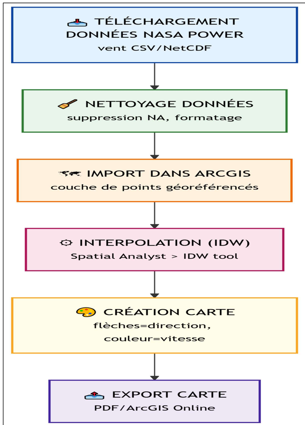
Figure 43: Méthodologie d'élaborer une carte des vents
