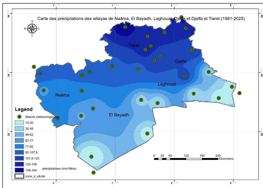
Figure 30: Carte de pluviométrie de la zone d'étude
