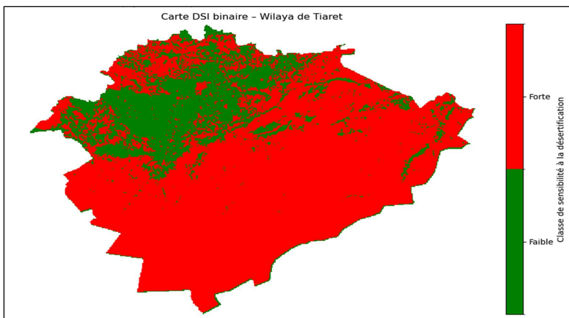
Figure 56: Carte DSI Wilaya Tiaret
