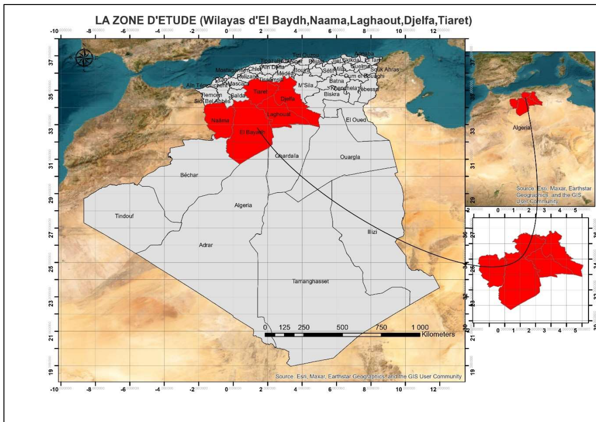
Figure 20: Carte de la zone d'étude
