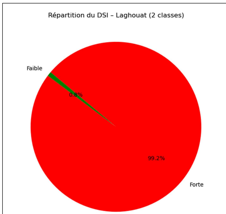
Figure 53: Répartition du DSI Pie chart Laghouat
