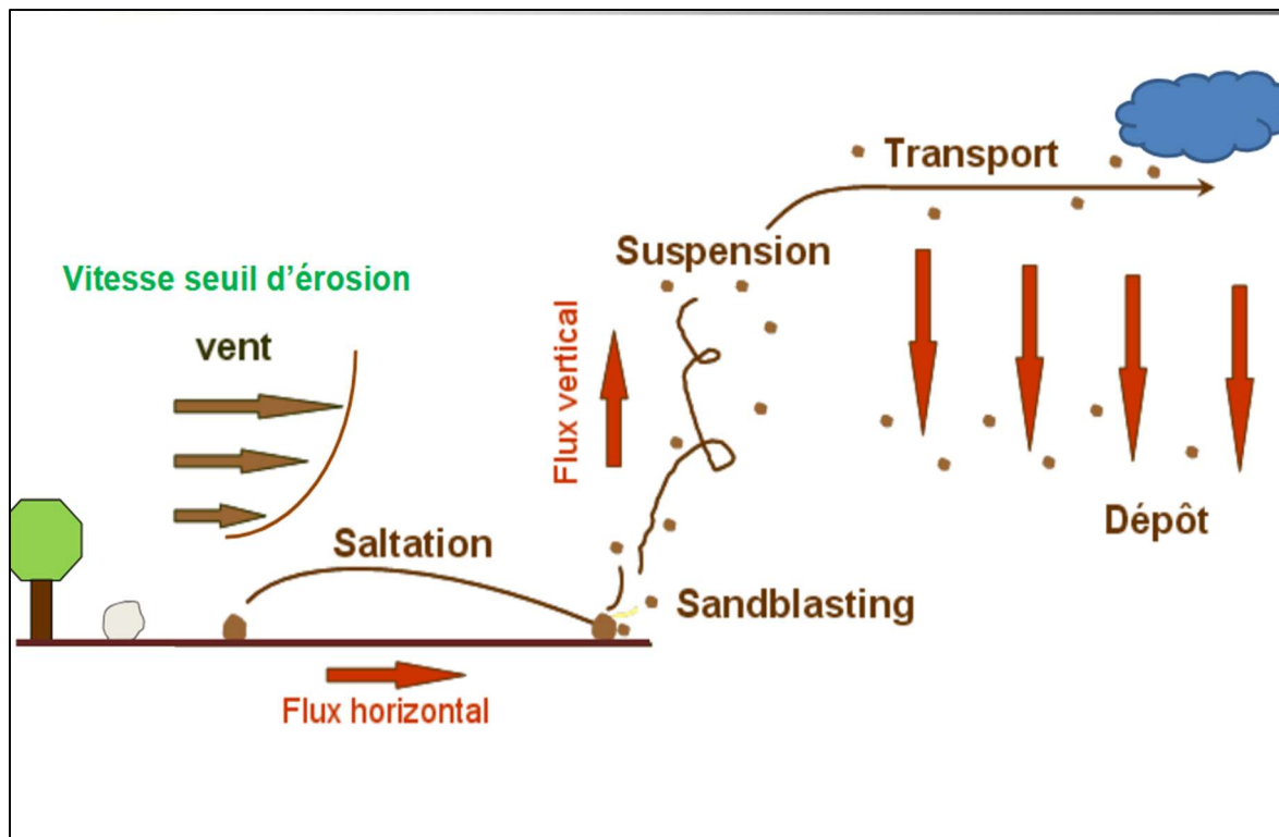
Figure 15: Erosion éolienne dans les régions arides et semi-arides image de Jean Louis RAJOT Christel BOUET
