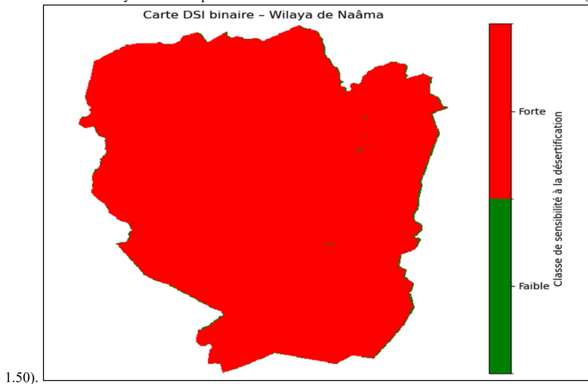
Figure 54: Carte DSI Wilaya Naama
