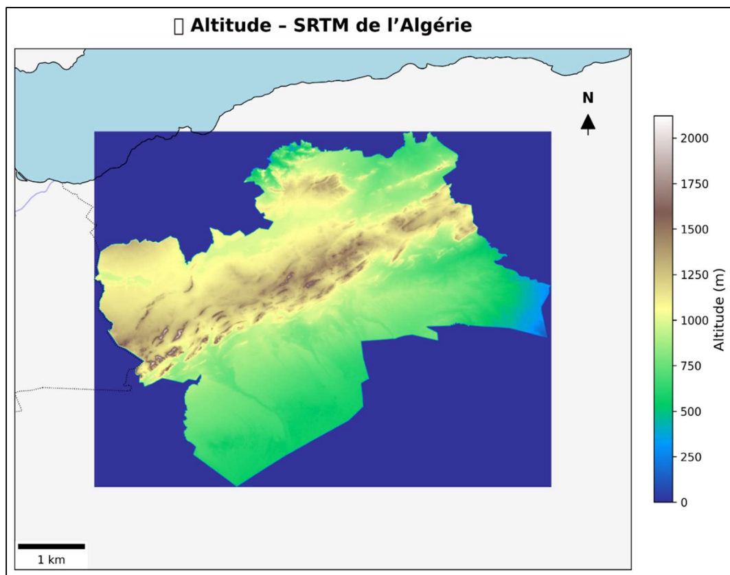
Figure 58: Topographie des Wilayas de la zone d'étude de gauche à droite Naama Elbayadh Lghouate Tiaret et Djelfa
