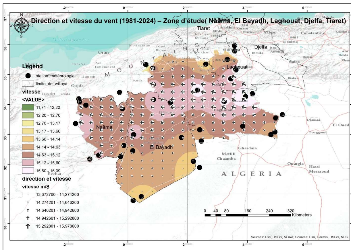
Figure 44: Carte des vents dans la zone d'étude
