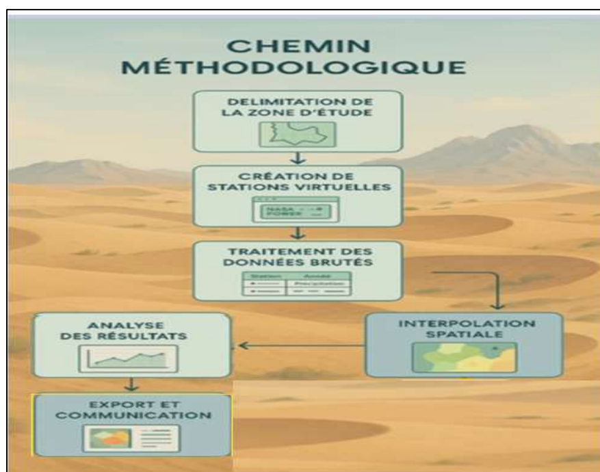
Figure 29: Méthodologie pour élaborer une carte de pluviométrie
