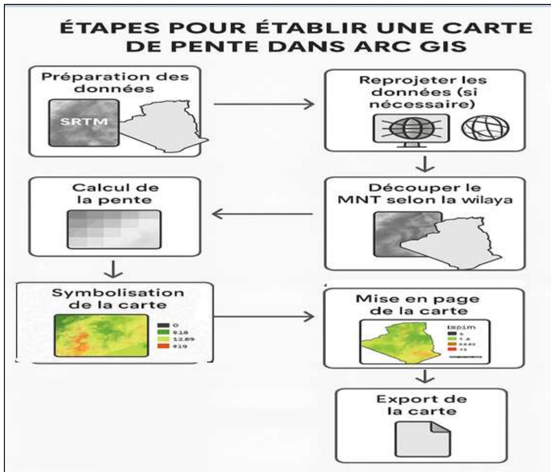
Figure 27: Méthodologie d'élaborer une carte de pente
