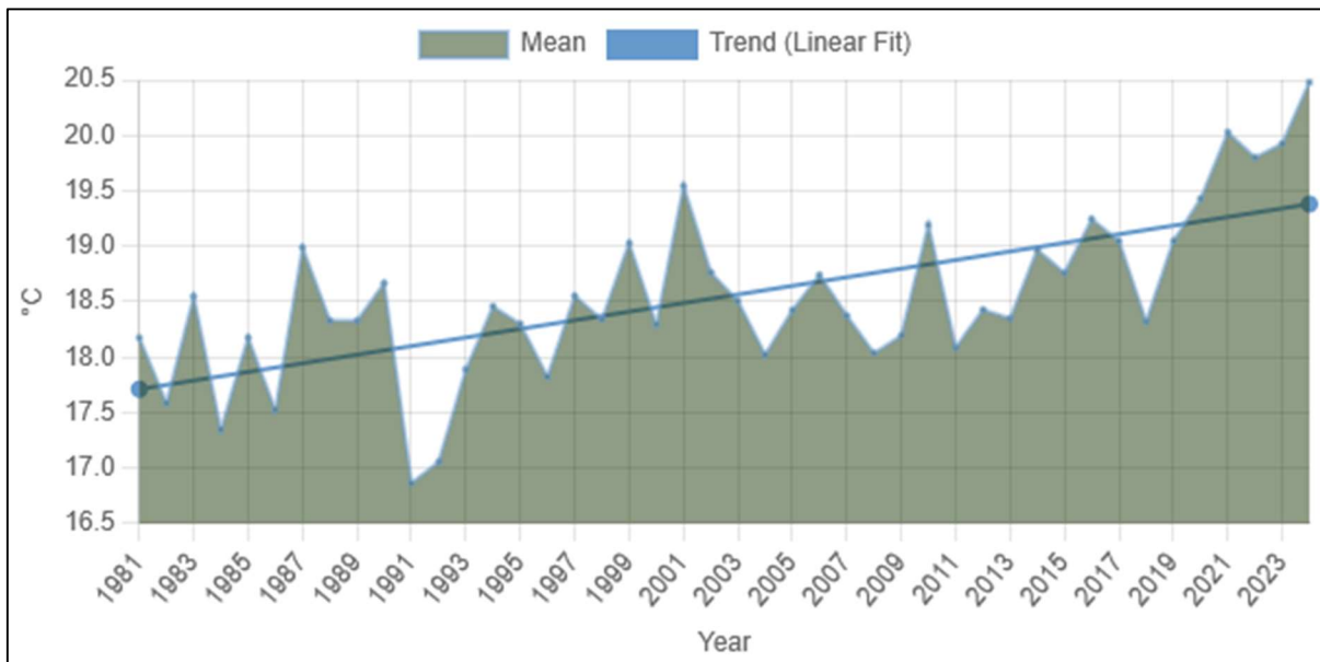
Figure 36: Analyse de la température moyenne de l'air en surface (annuelle) dans la wilaya de Laghouat (1981-2023)
