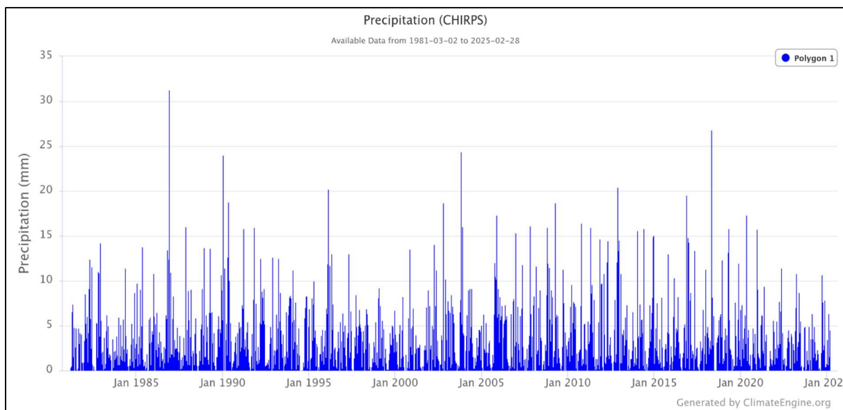
Figure 33: Analyse de la précipitation dans la wilaya de Naama (1981-2025)
