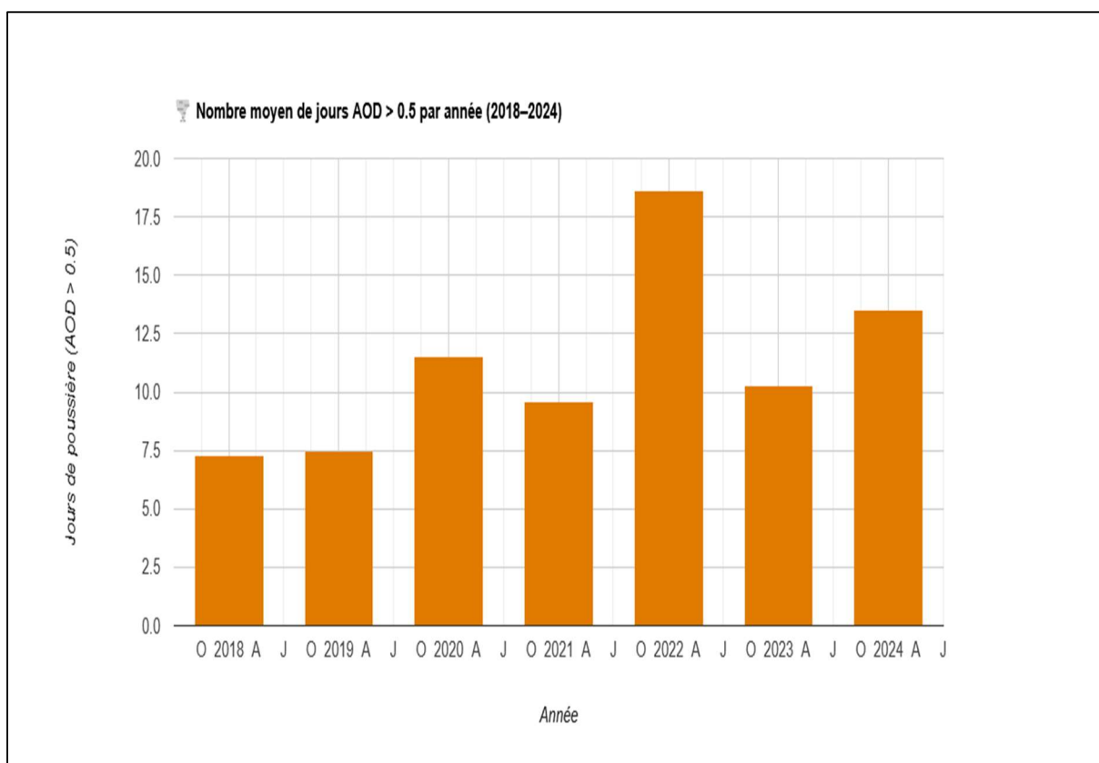
Figure 45: L'année la plus poussiéreuse dans la période du 2018 au 2024
