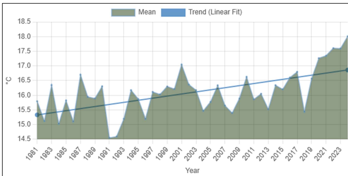
Figure 39: Analyse de la température moyenne de l'air en surface (annuelle) dans la wilaya de Naama (1981-2023)
