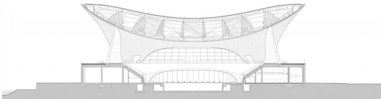
Fig54. Coupe
