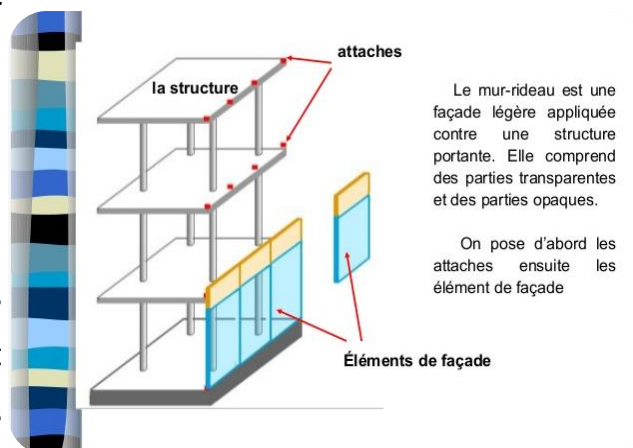
Fig241. Mur du mur rideau
