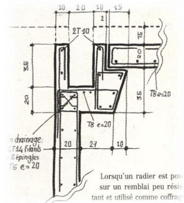
Fig125. Détail du ferrailage de l'appui d'une plage sur une chéneau de piscine à débordement
