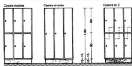
⑧ Casiers de vestiaires (exemples).
