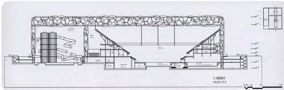
Fig88. Coupe
