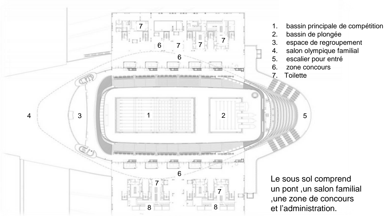
Fig47. Plan sous-sol
