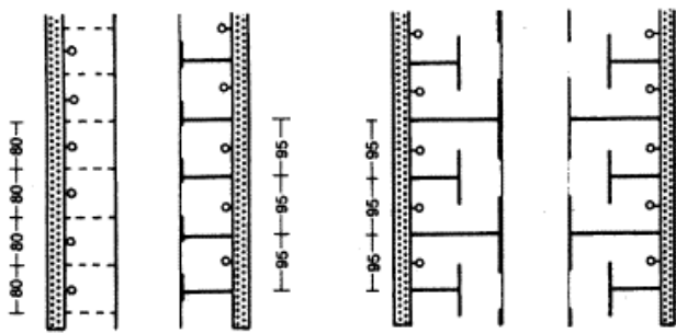
⑥ Rangée de douches ouvertes et de douches avec écran contre écia-boussures. ⑦ Rangée de douches avec écran visuel.
