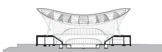
Fig57. Coupe
