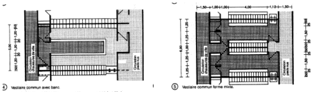
Fig156. Détail des vestiaire Neufert 8émé édition
