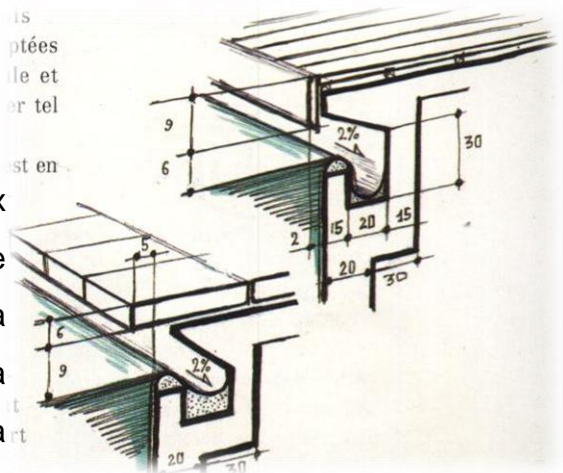
Fig128. Débordement à gorge périphérique
