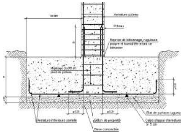
Figure 87 schéma sur semelle isolé
