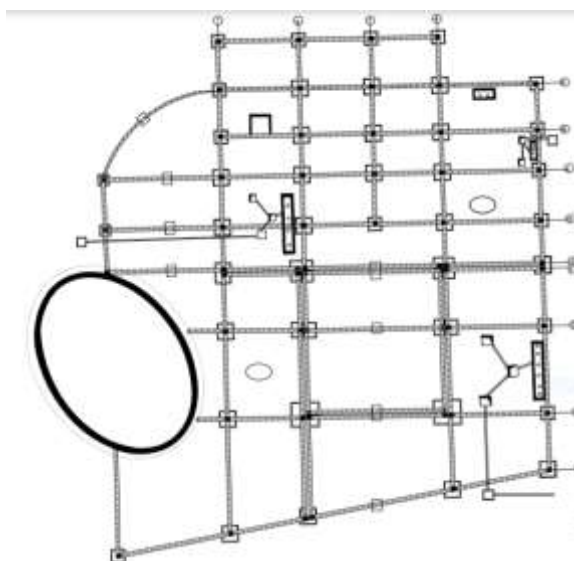
Figure 86 plan de fondation
