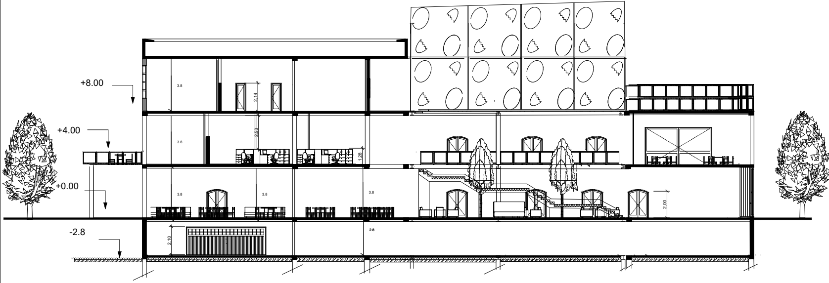
COUPE AA 1/200
