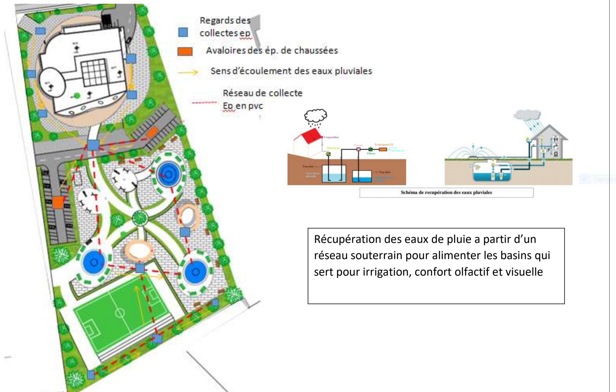
Schéma de gestion de l'eau
