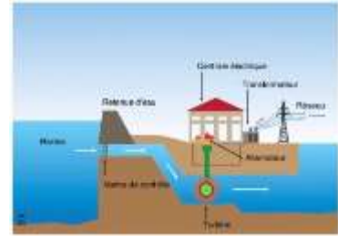
Figure 14 schéma présentant l'énergie hydraulique
