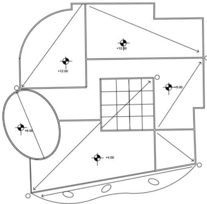
Plan de toiture 1/200
