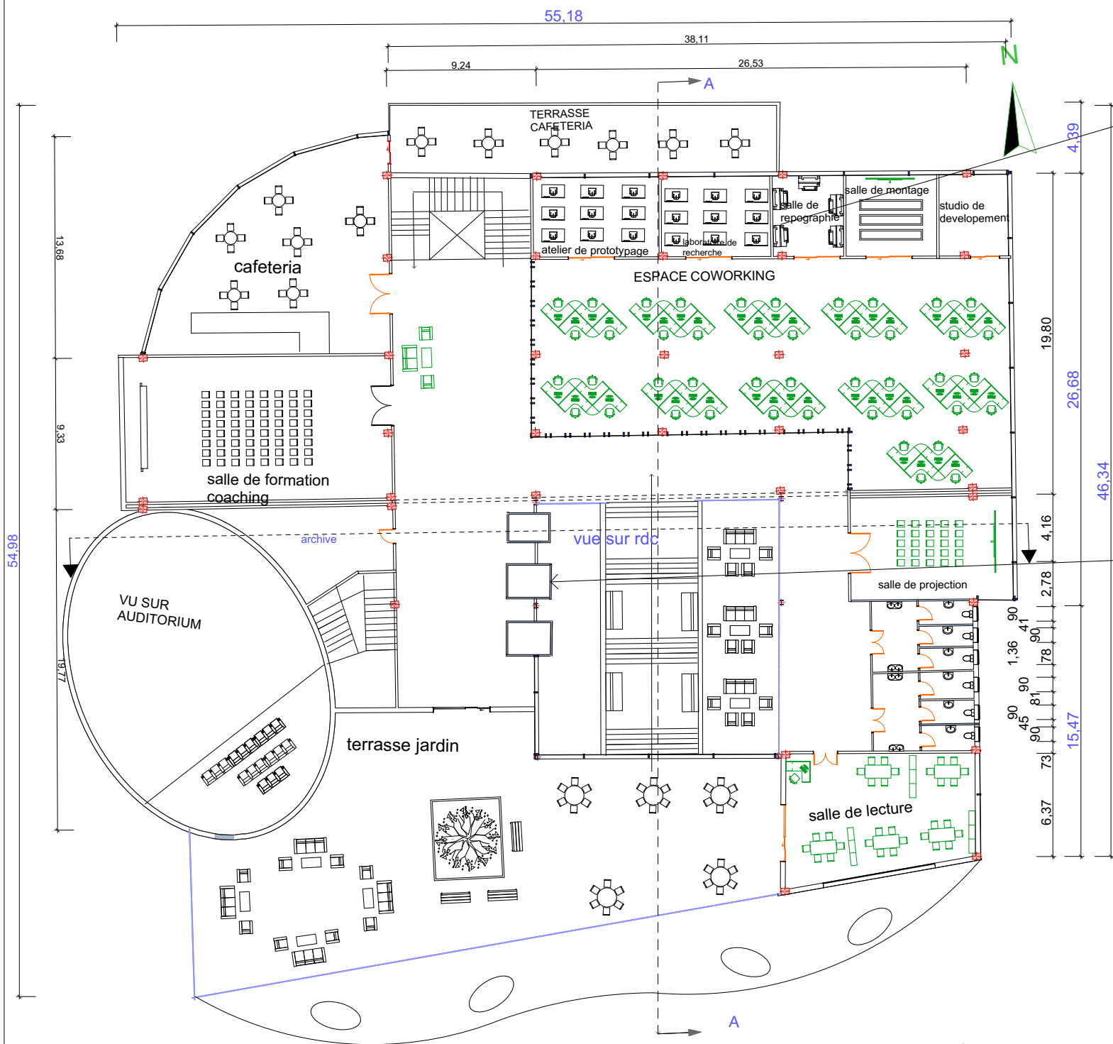
plan 1 etage 1/200
