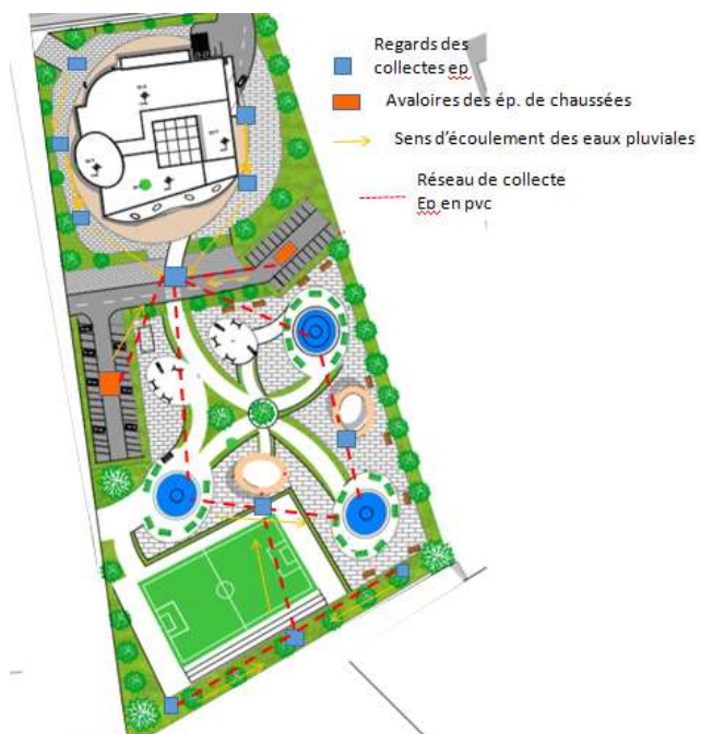
schema de recuperation des eaux pluviales
