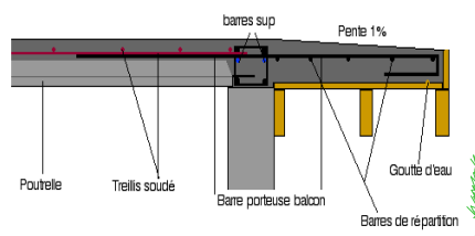
detail dalle pleine
