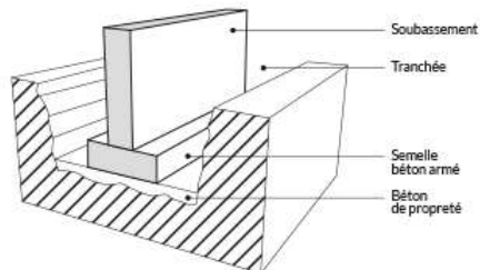
Figure 88 schéma semelle filante
