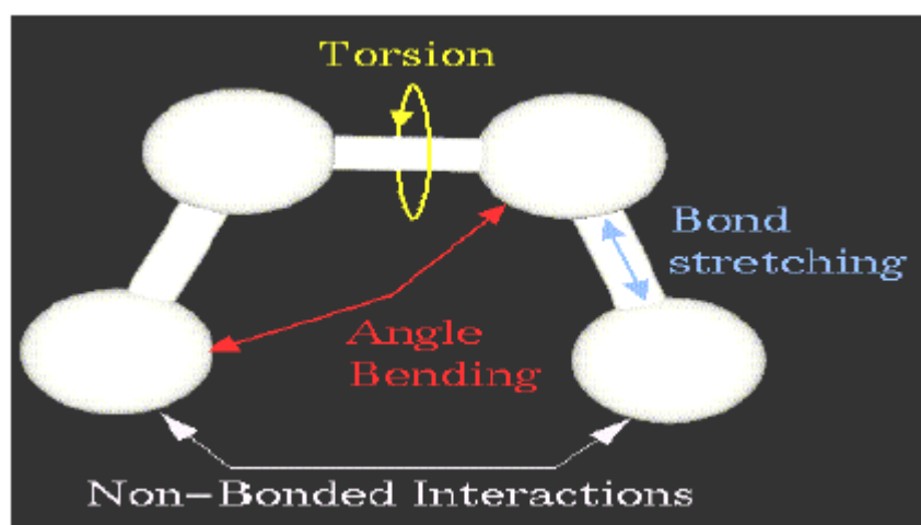
Figure8 : mécanique moléculaire
