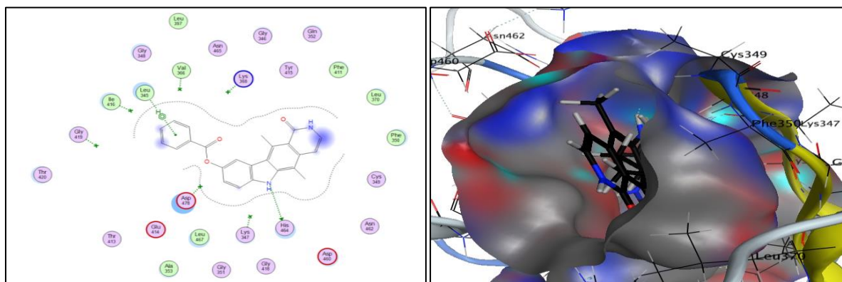
Figure14 : Interaction entre 5NXC et L1
