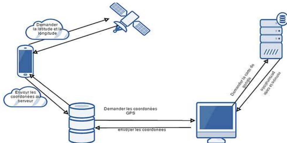
Figure III.20 Schéma du système de géolocalisation
