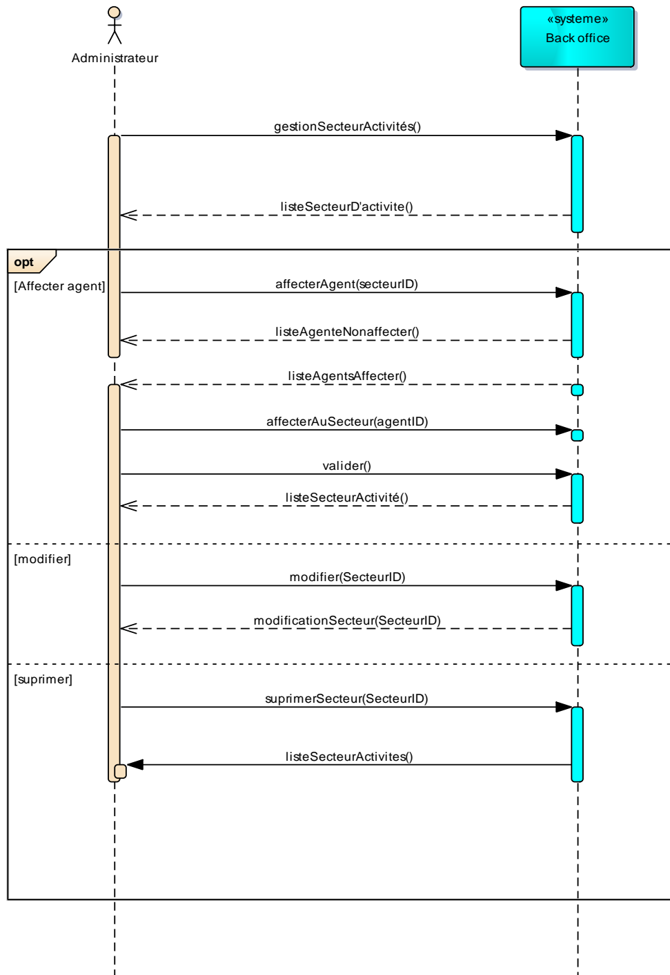
Figure II.15 Diagramme de Séquence « gérer les secteurs d'activité »
