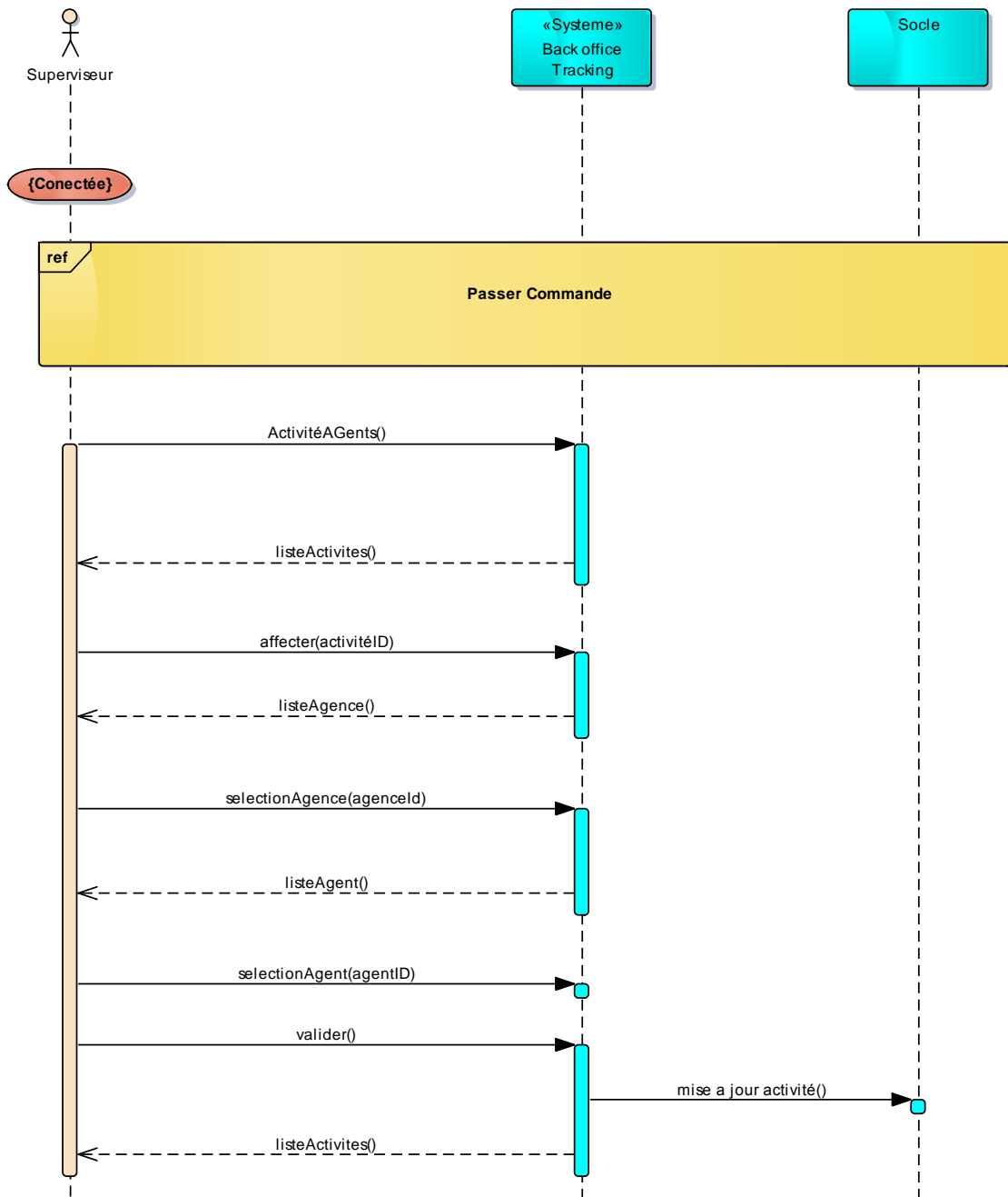
Figure II.4 Diagramme de Séquence « Affecter une activité »
