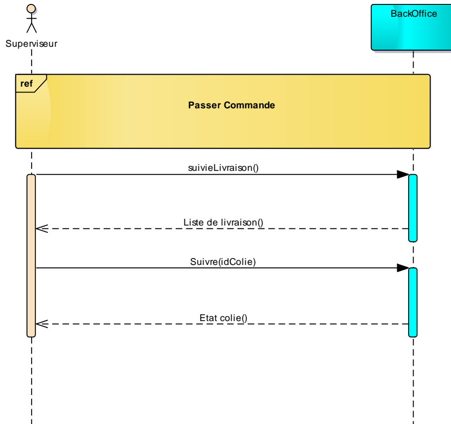
Figure II.11 Diagramme de Séquence « Traquer colis Superviseur »
