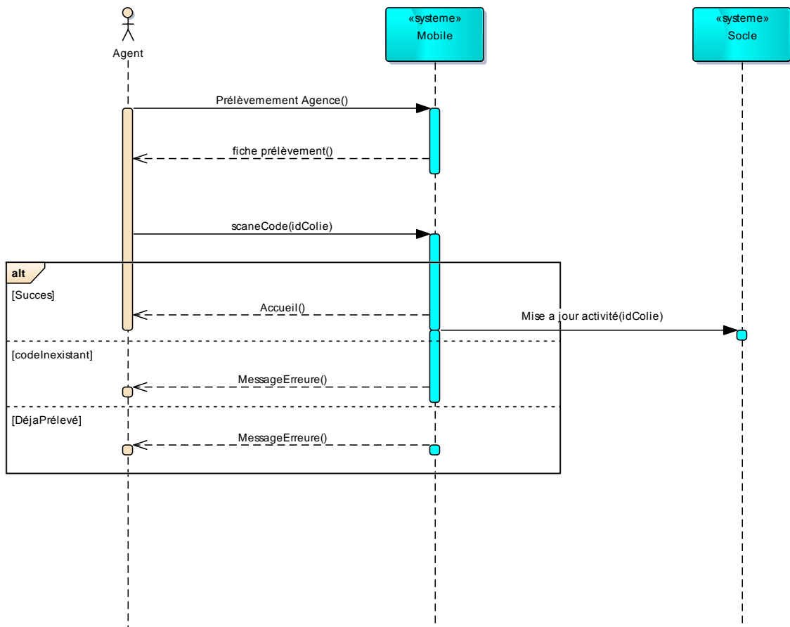
Figure II.8 Diagramme de Séquence « Prélèvement Agence »
