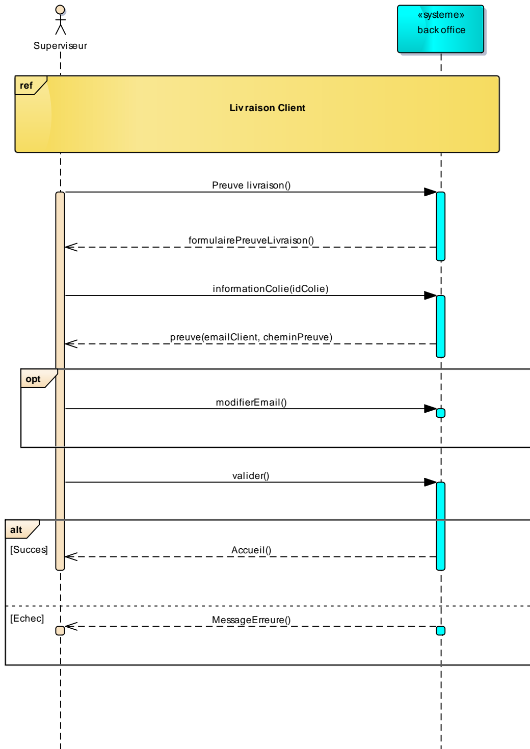
Figure II.16 Diagramme de Séquence « Fournir la preuve de livraison »
