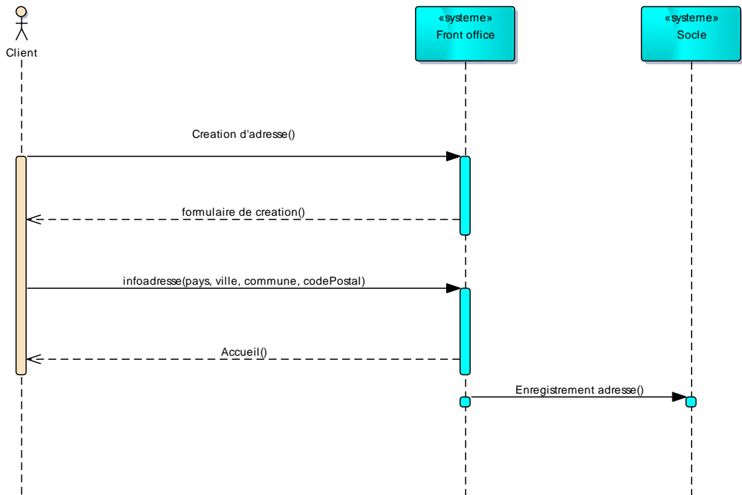
Figure II.2 Diagramme de séquence « créer adresse »
