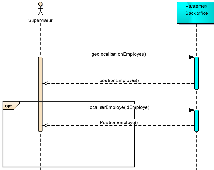
Figure II.12 Diagramme de Séquence « géo localiser un employé »
