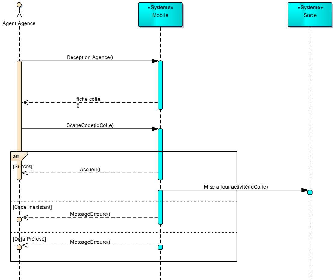
Figure II.7 Diagramme de Séquence « Réception Agence »
