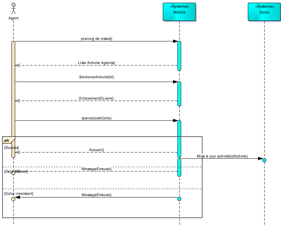
Figure II.6 Diagramme de Séquence « Prélèvement client »
