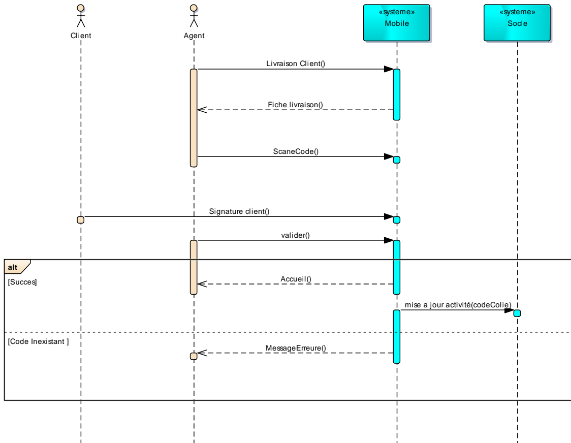
Figure II.9 Diagramme de Séquence « Livraison Client »
