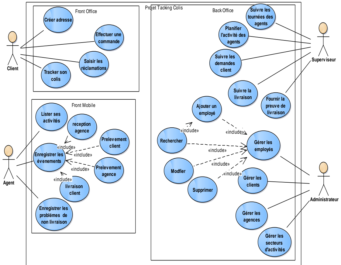
Figure II.1 Diagramme de cas d'utilisation
