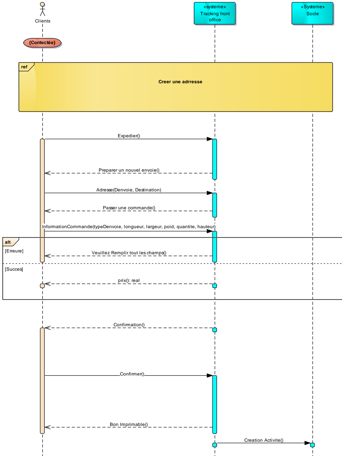
Figure II.3 Diagramme de séquence « passer commande »
