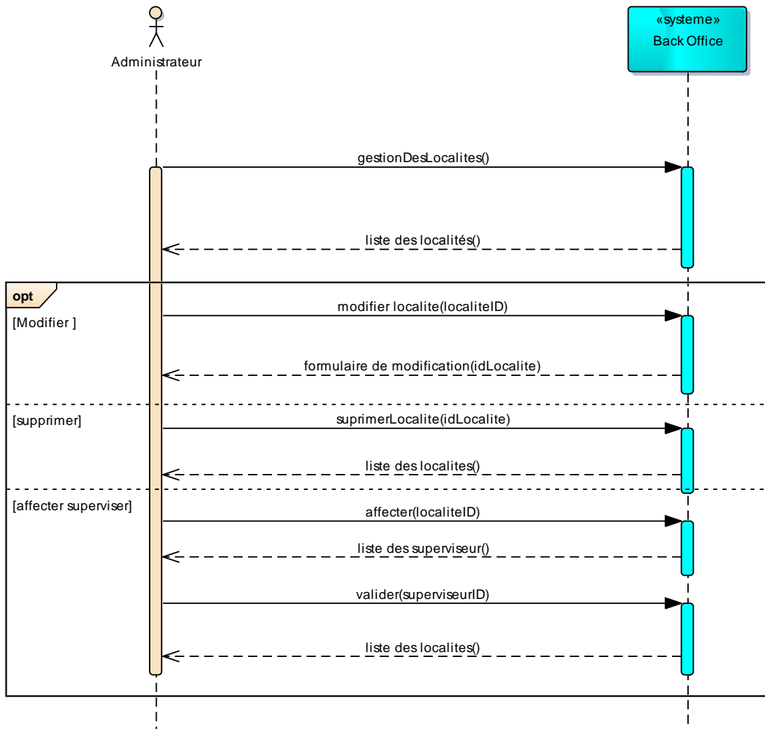
Figure II.14 Diagramme de Séquence « gérer les localités »
