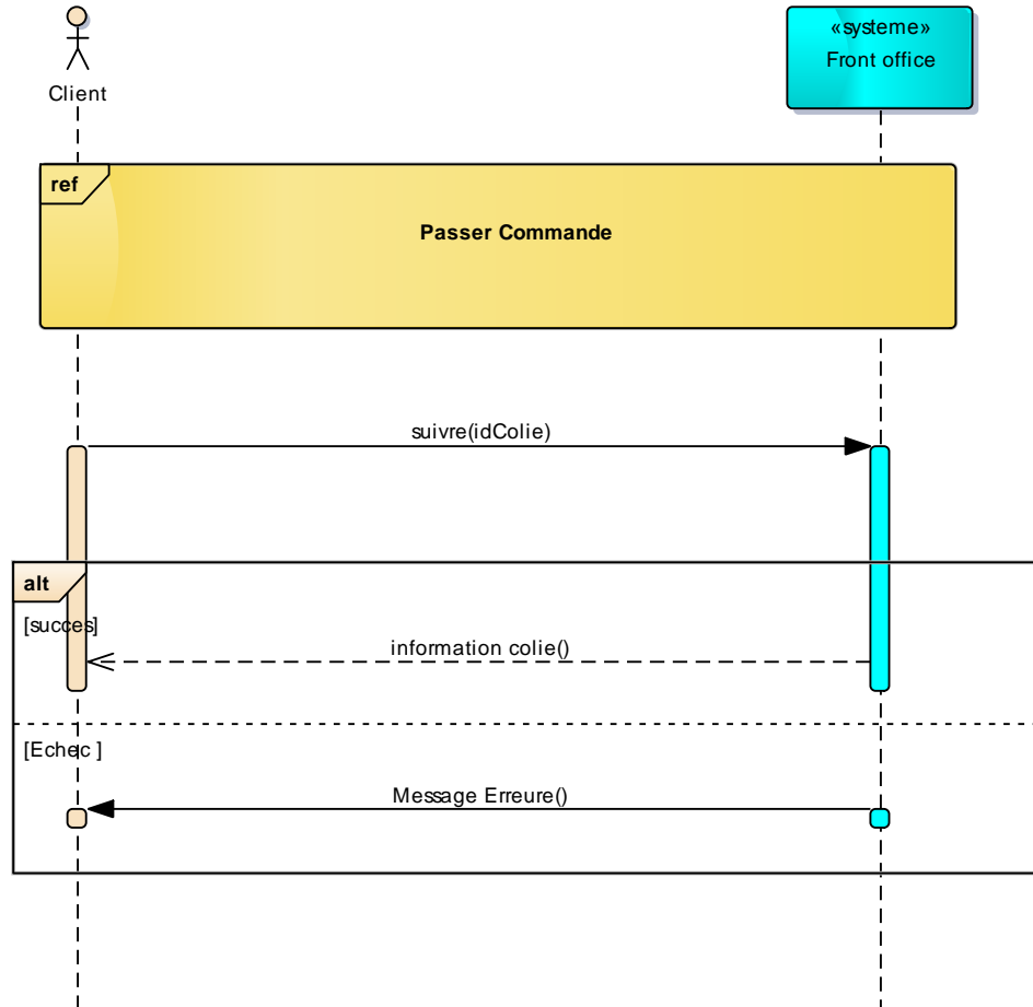
Figure II.10 Diagramme de Séquence « Traquer colis client »
