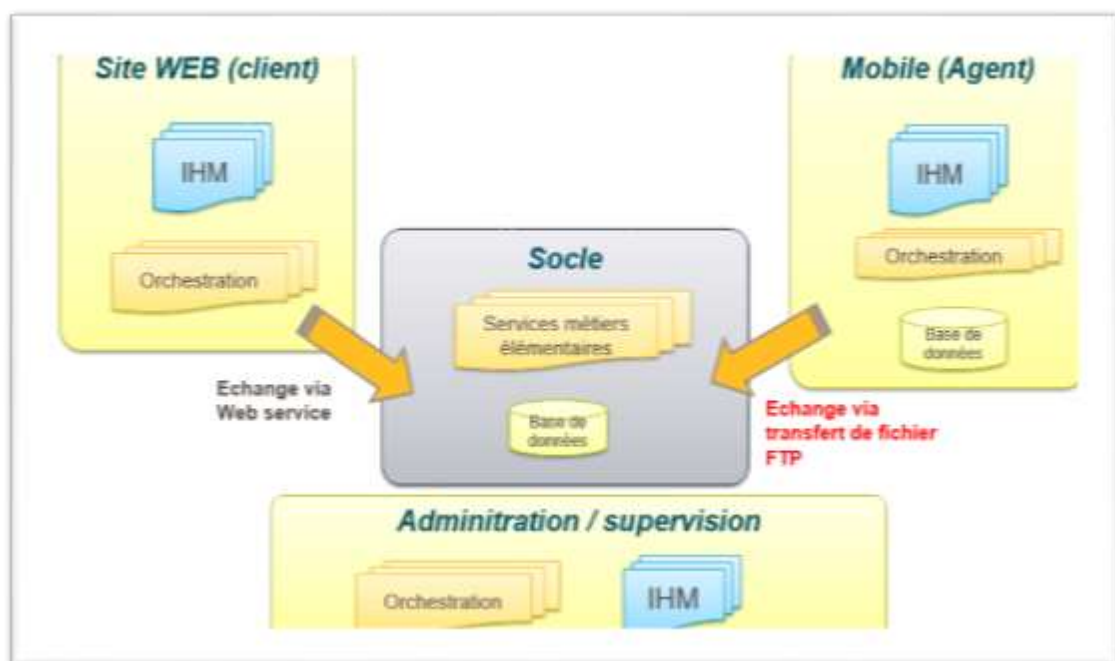
Figure I.1 Architecture globale du projet Tracking Colis
