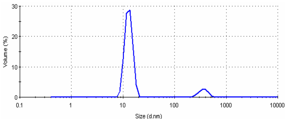
Figure 14. Répartition de la taille du volume obtenue pour un échantillon d'or colloïdal [25].
