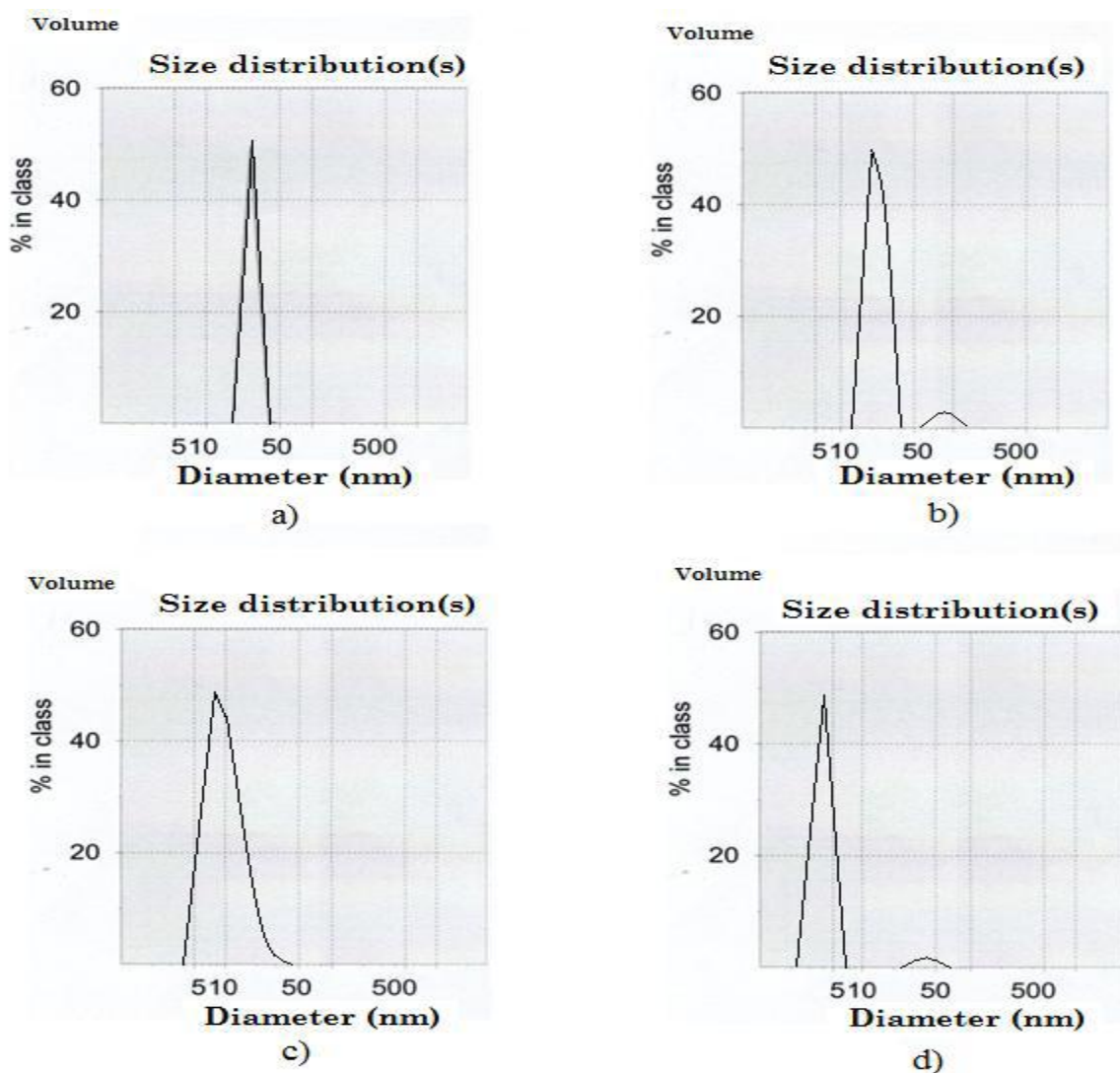
Figure 18. Analyse granulométrique de la solution colloïdale des nanoparticules de taille moyenne en volume: a) 26,6 nm ; b) 21,1 nm ; c) 7,8 nm et d) 4,2 nm.
