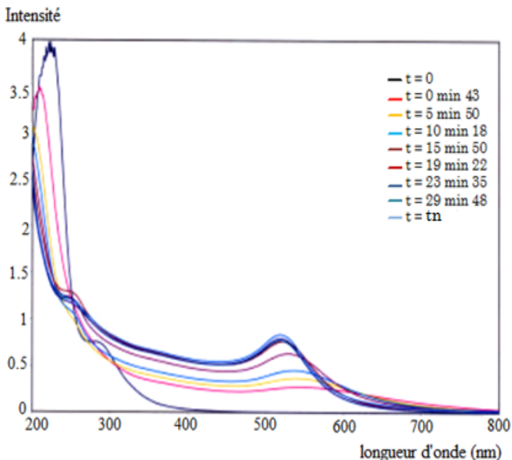
Figure 20. Étude cinétique de la croissance des particules par la méthode utilisant le mélange citrate de sodium/acide tannique (suivie par spectrophotométrie UV-visible).
