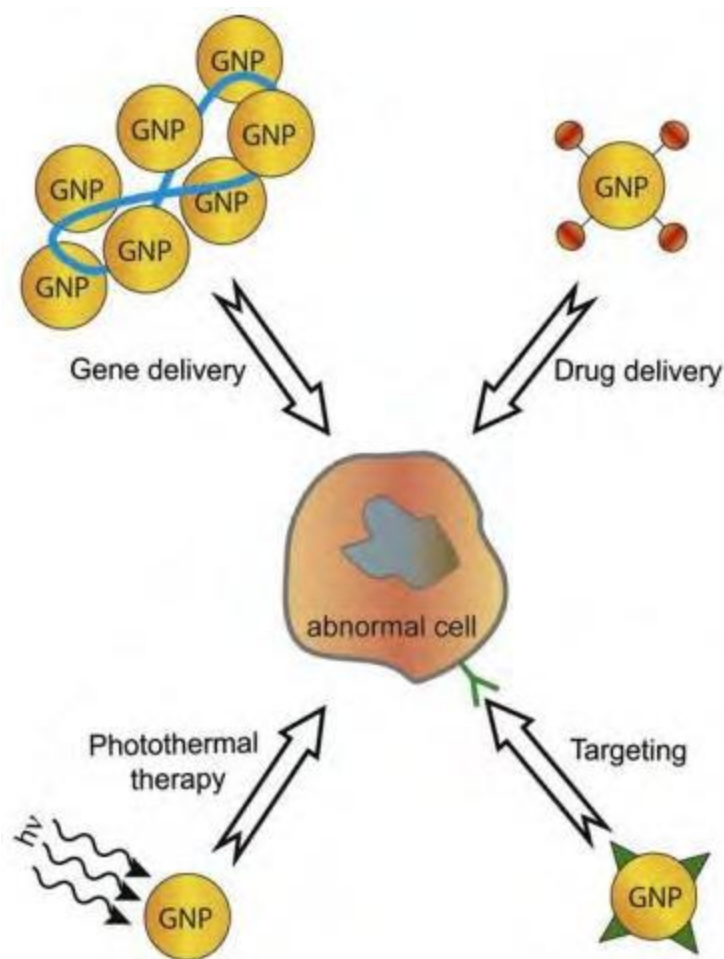
Figure 3. Schéma représentant les différentes applications médicales des nanoparticules d'or.
