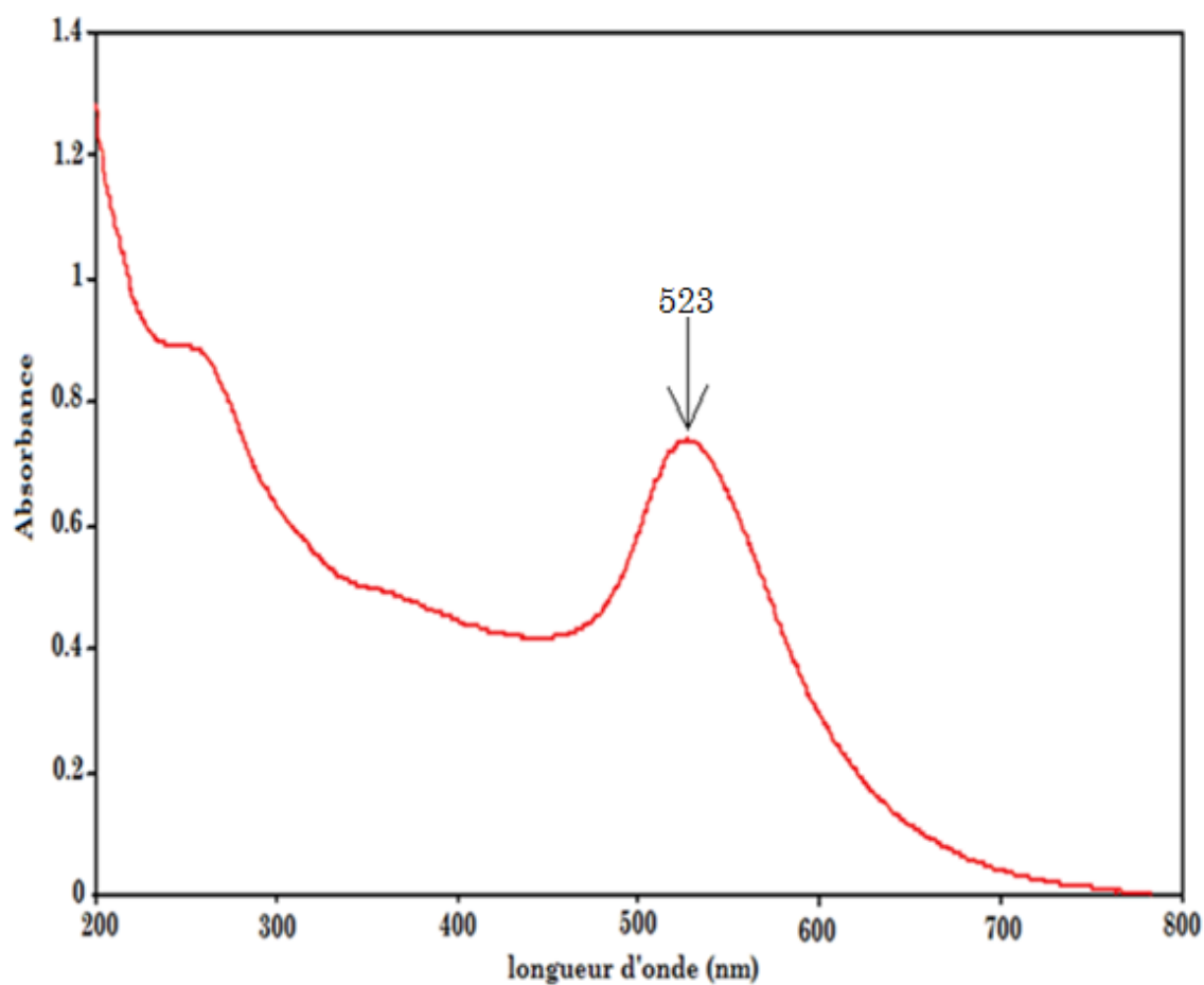
Figure 16: spectre UV-visible de la solution colloïdale de nanoparticules d'or.
