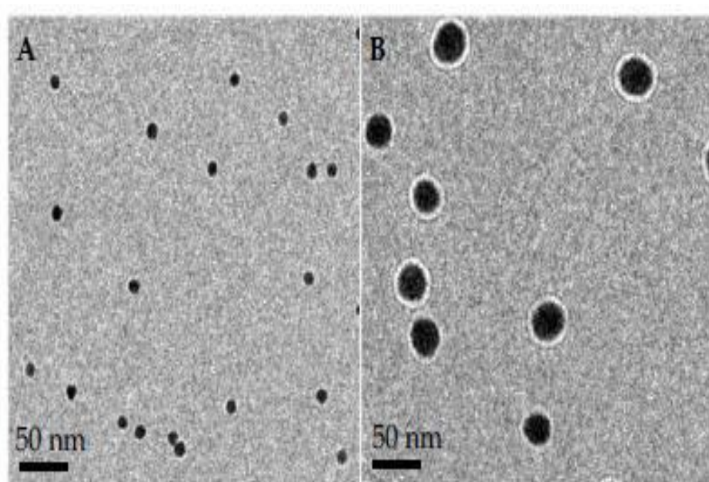
Figure 5. Images TEM de nanoparticules d'or d'un diamètre moyen de A 15 nm, B 40 nm [24]
