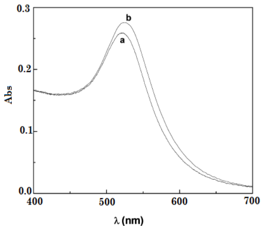
Figure 15: Spectre d'absorption UV-vis de GNPs (0,05 mM) en l'absence (courbe a) et en présence de micelles de caséine (5.0 mg/ml) (courbe b) [27].
