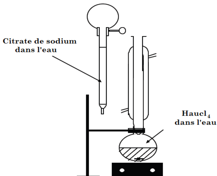
Figure 4. Schema du montages pour la synthèse à l'aide de sodium ( \text{C}_6\text{H}_5\text{O}_7\text{Na}_3 \cdot 2\text{H}_2\text{O} ).
