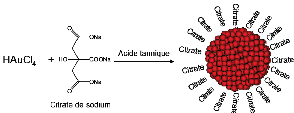
Figure 2. Synthèse des nanoparticules par la voie citrate/ acide tannique.
