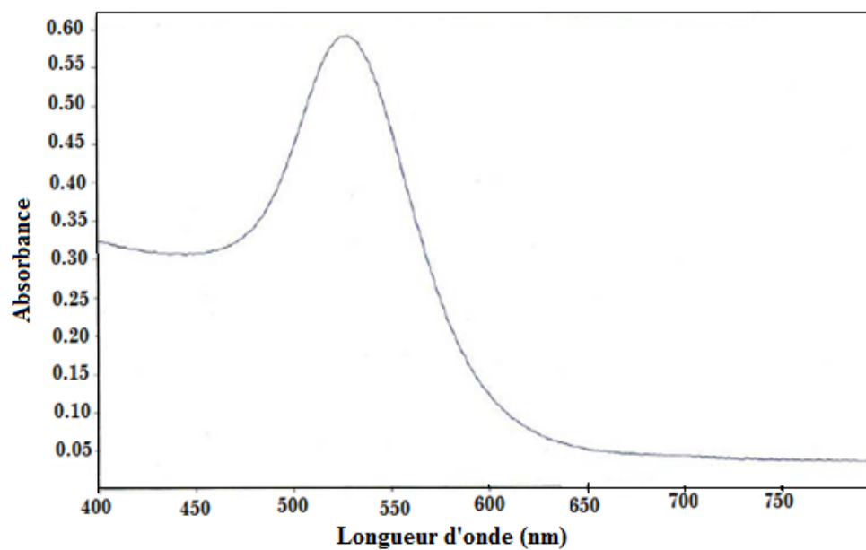
Figure 7. Spectre d'absorption UV-vis des nanoparticules d'or [24].
