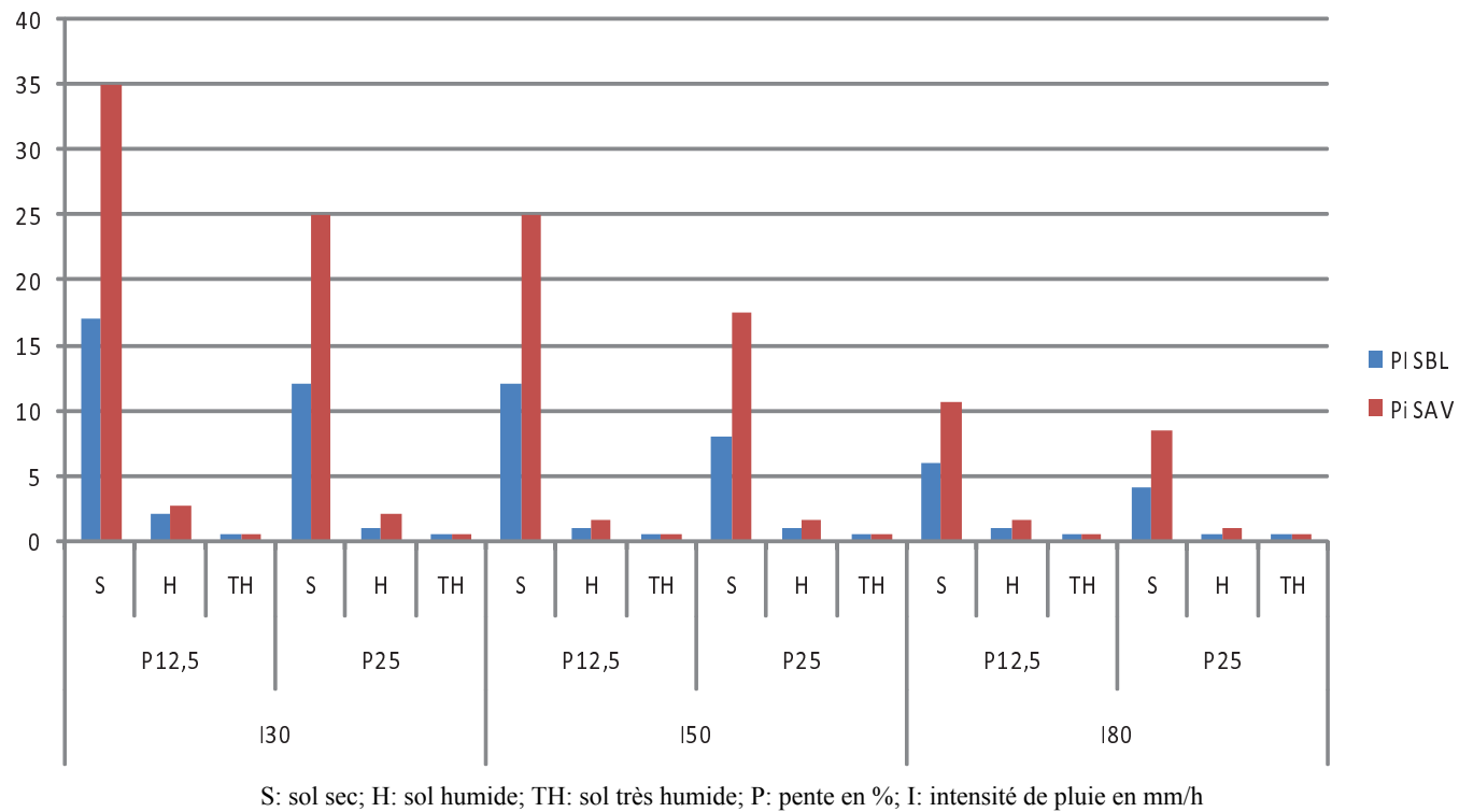
Fig. 3. Effet des états de surface et de l'intensité de pluie sur la pluie d'imbibition
