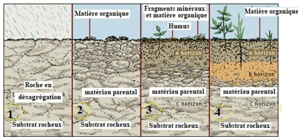
Figure 1. Processus de la formation d'un sol (source : Microsoft® Encarta® 99).
