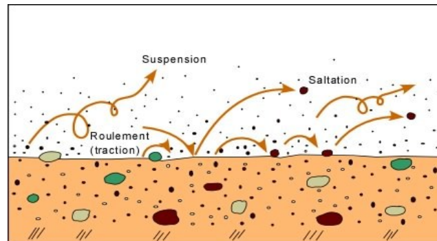
Figure 8. Schéma de l'effet de l'érosion éolienne. 8
