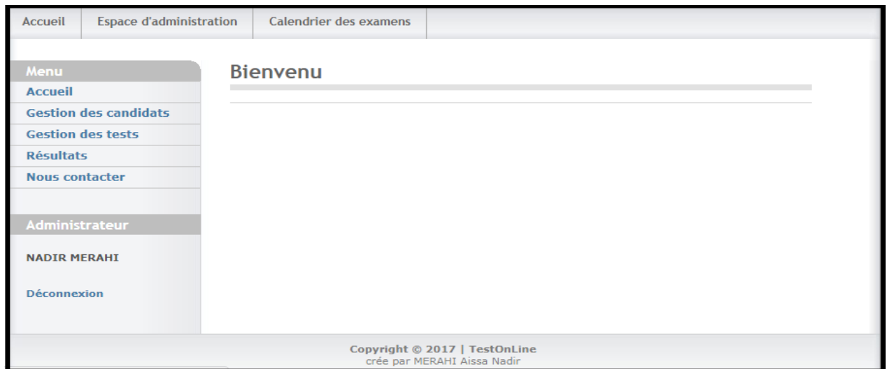
Figure 17: Espace administrateur
