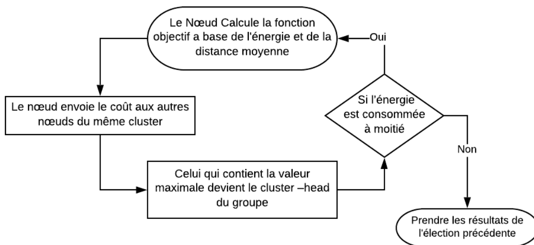
Figure III.5 Processus d'élection des cluster-heads
