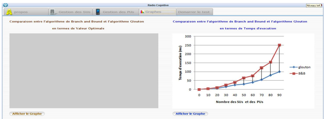
Figure III.14: Comparaison entre l'algorithme de B&B et l'algorithme Glouton
