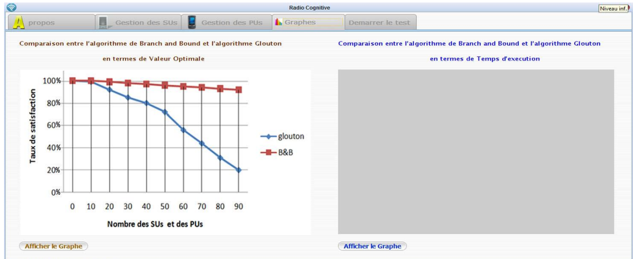
Figure III.13: Comparaison entre l'algorithme de B&B et l'algorithme Glouton
