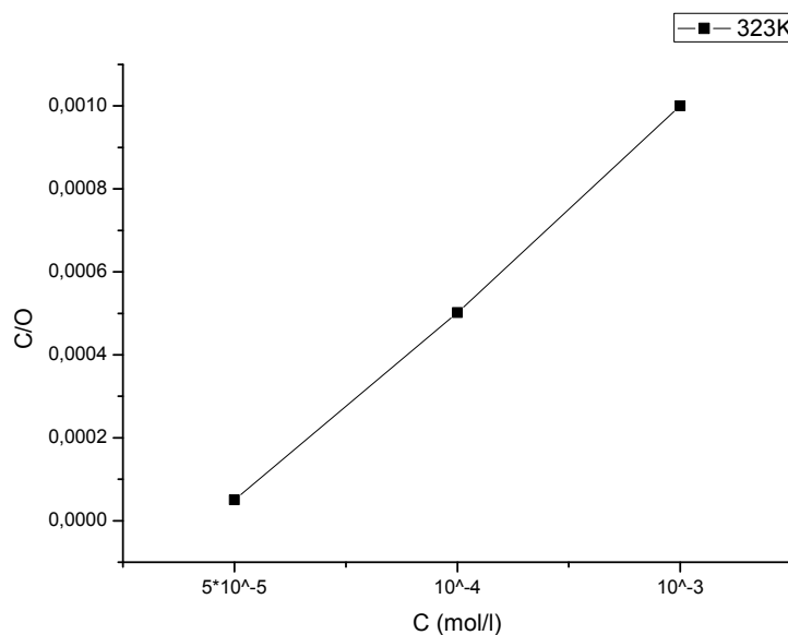
Fig. II-10 : Isotherme de LANGMUIR du l'acier dans HCl 1M en présence de différentes concentrations d'Amide à 323K
