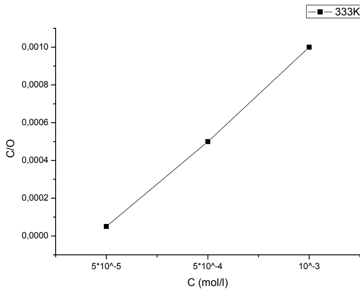
Fig. II-10 : Isotherme de LANGMUIR du l'acier dans HCl 1M en présence de différentes concentrations d'Amide à 333K
