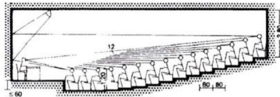
④ Forme normale d'amphithéâtre
