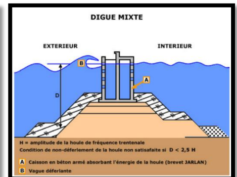
Figure 214 : digue mixte
