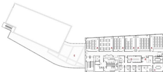
Figure 56: plan 2 eme étage
