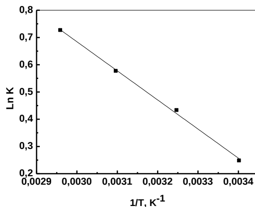
Figure 134: Evolution de \ln K_d en fonction de 1/T pour l'extraction de Pb(II) par la résine Lewatit TP 214, [Pb(II)]_i = 1,0 \cdot 10^{-3} mol/L, m = 0,050 g, V = 5 mL, pH_i = 4,5 , \emptyset = 250 tpm.
