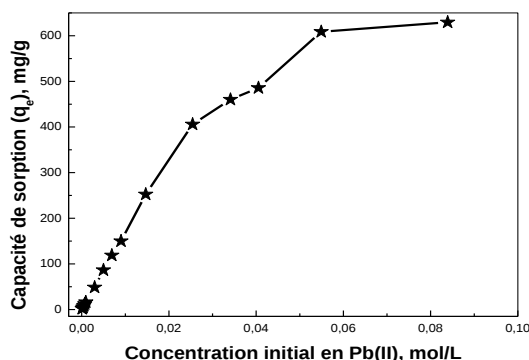
Figure 57 : Effet de la concentration initiale du Pb(II) sur la capacité de son sorption sur la Lewatit TP 207, m \approx 0.0600 g, t_{\text{agitation}} = 15 mn, \varnothing = 250 tpm.
