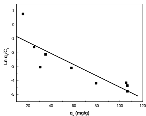
Figure 41 : Modèle de Elovich appliqué à l'extraction de La(III) par la résine Lewatit TP 260, m = 0,1000 g, V_{sol} = 5 mL, t_{agitation} = 30 mn, \varnothing = 250 tpm
