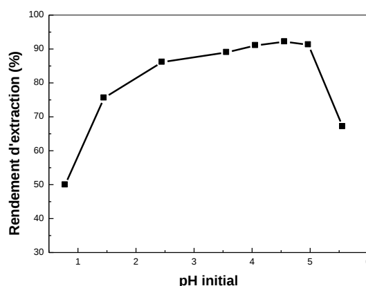
Figure 74: Effet du pH initial sur le rendement d'extraction de Pb(II) par la Lewatit TP 260, [Pb(II)]_0 = 5.10^{-4} mol/L, V_{sol} = 5 mL, m = 0,060 g, t_{agitation} = 60 min, \varnothing = 250 tpm
