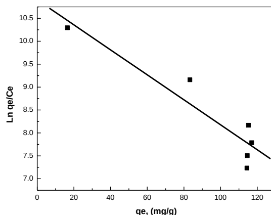
Figure 18: Application du modèle d'Elovich à l'isotherme d'extraction de La(III) par la résine Lewatit TP 207, m = 0.1000 g, V_{\text{sol}} = 5 mL, t_{\text{agitation}} = 20 mn, \varnothing = 250 tpm
