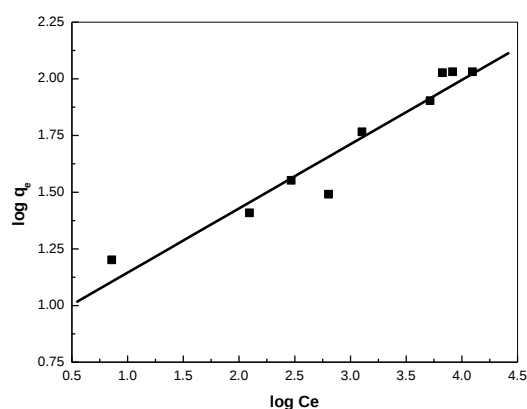
Figure 40 : Modèle de Freundlich appliqué à l'extraction de La(III) par la résine Lewatit TP 260, m = 0,1000 g, V_{sol} = 5 mL, t_{agitation} = 30 mn, \varnothing = 250 tpm
