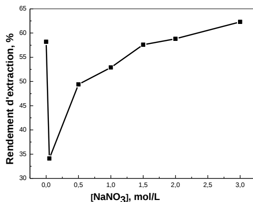
Figure 112: Effet de la concentration en \text{NaNO}_3 sur le rendement d'extraction de \text{Cd(II)} par la Lewatit TP 214, m = 0,0500 g, V = 5,0 mL, \text{pH}_i = 5,0 , [\text{Cd}^{2+}]_i = 1,0 \cdot 10^{-3} mol/L, t = 60 mn, \varnothing = 250 tpm.
