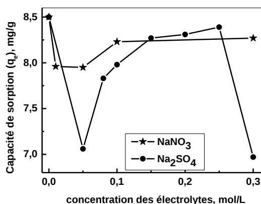
Figure 59 : Effet de l'ajout d'un sel sur la capacité de sorption de Pb(II) par la Lewatit TP 207, [\text{Pb(II)}]_0 = 5,0 \cdot 10^{-4} \text{ M} , V = 5 \text{ mL} , m = 0.0600 \text{ g} , t_{\text{agitation}} = 15 \text{ mn} , \varnothing = 250 \text{ tpm} .
