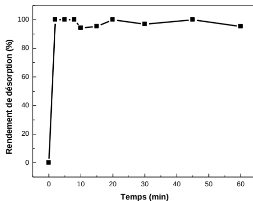
Figure 49: Effet du temps de contact sur le rendement de la désorption du \text{La(III)} retenu par la résine Lewatit TP 260, V_{\text{acide sulfurique}} = 5,0 \text{ mL} , [\text{H}_2\text{SO}_4] = 2,5 \text{ M} , m = 0,100 \text{ g} , \varnothing = 250 \text{ tpm}
