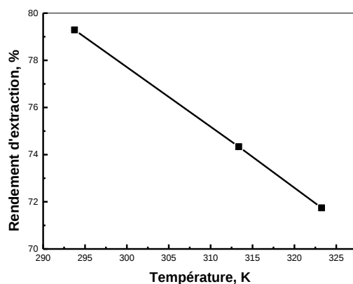
Figure 81 : Effet de la température sur le rendement de l'extraction de Pb(II) par la Lewatit TP 260, [\text{Pb(II)}]_i = 5.10^{-4} mol/L, m = 0,0600 g, V = 5 mL, \text{pHi} \approx 1,15 , \varnothing = 250 tpm
