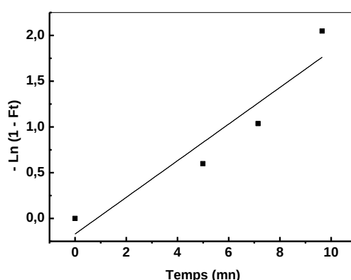
Figure 123: Modèle de diffusion externe appliqué à la cinétique de sorption des ions \text{Pb}^{2+} sur la résine Lewatit TP214, [\text{Pb(II)}]_0 = 1,0 \cdot 10^{-3} \text{ M} , m = 0.050 \text{ g} , V = 5 \text{ mL} , \text{pHi} = 4,5 , \emptyset = 250 \text{ tpm} .
