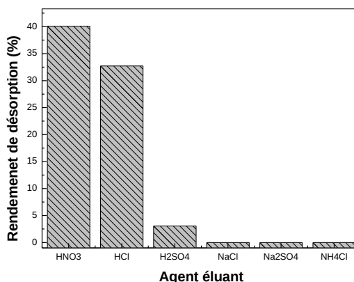
Figure 92: Effet de la nature de l'éluant sur le rendement de désorption des ions Pb^{2+} à partir de la Lewatit TP 260 chargée en métal, V_{Eluant} = 5,0 mL, m_{résine\ saturée\ en\ Pb(II)} = 0,060 g, \varnothing = 250 tpm
