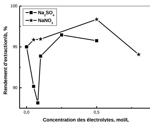
Figure 79 : Effet de l'ajout d'un sel sur le rendement de sorption de Pb(II) par la Lewatit TP 260, [\text{Pb(II)}]_0 = 5,0 \cdot 10^{-4} \text{ M} , V = 5 \text{ mL} , m = 0,0600 \text{ g} , t_{\text{agitation}} = 15 \text{ mn} , \varnothing = 250 \text{ tpm}
