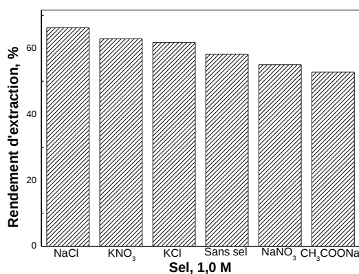
Figure 110 : Effet de la nature du sel ajouté sur le rendement d'extraction de Cd(II) par la Lewatit TP 214, m = 0,050 g, V = 5,0 mL, pH i = 5,0, [Cd 2+ ] = 1,0 10 -3 mol/L, t = 60 mn, Ø = 250 tpm
