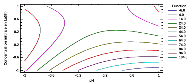
Figure 135 : La surface de réponse et la courbe iso-réponse montrant l'effet de pH et de la concentration en métal et leur effet mutuel sur le rendement d'extraction avec X_1 = 0
