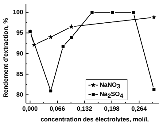
Figure 58 : Effet de l'ajout d'un sel sur le rendement de sorption de Pb(II) par la Lewatit TP 207, [\text{Pb(II)}]_0 = 5,0 \cdot 10^{-4} \text{ M} , V = 5 \text{ mL} , m = 0.0600 \text{ g} , t_{\text{agitation}} = 15 \text{ mn} , \varnothing = 250 \text{ tpm} .
