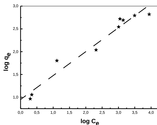
Figure 90: Modèle de Freundlich appliqué à l'extraction de Pb(II) par la résine Lewatit TP 260, m = 0.0600 \text{ g} , V_{\text{sol}} = 5 \text{ mL} , t = 15 \text{ mn} , \varnothing = 250 \text{ tpm}
