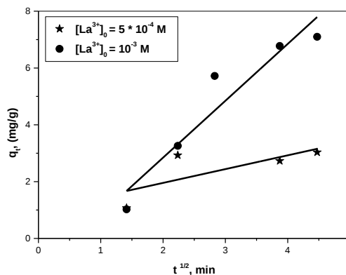
Figure 34: Application du modèle de Morris-Webber à la cinétique de sorption des ions \text{La}^{3+} par la résine Lewatit TP 260, m = 0,1000 \text{ g} , V_{\text{sol}} = 5 \text{ mL} , \text{pH}_{\text{initial}} \approx 5.19 , \varnothing = 250 \text{ tpm}
