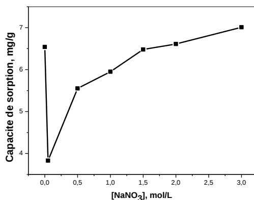
Figure 113: Effet de la concentration en \text{NaNO}_3 sur la capacité d'extraction de \text{Cd(II)} par la Lewatit TP 214, m = 0,0500 g, V = 5\text{mL} , \text{pH}_i = 5,0 , [\text{Cd(II)}]_i = 1,0 \cdot 10^{-3} mol/L, t = 60 mn, \varnothing = 250 tpm.
