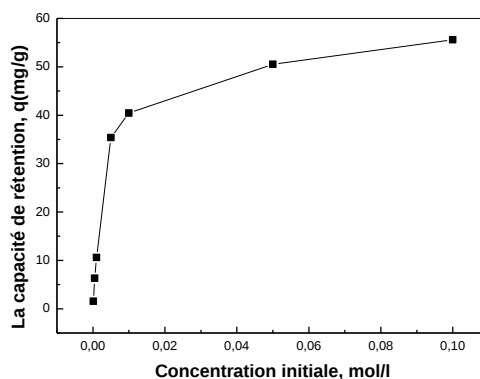
Figure 127: Influence de la concentration initiale en Pb(II) sur la capacité de rétention des ions de \text{Pb}^{2+} par la résine Lewatit TP 214, \text{pH}_i = 4,5 , m = 0,050 g, V = 5 mL, t = 30 mn, \varnothing = 250 tpm.
