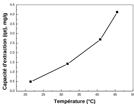
Figure 22 : Effet de la température sur la capacité d'extraction de \text{La}^{3+} par la Lewatit TP 207, [\text{La}^{3+}]_i = 5.10^{-4} mol/L, m = 0,100 g, V = 5 mL, \text{pHi} \approx 3,46 , \varnothing = 250 tpm
