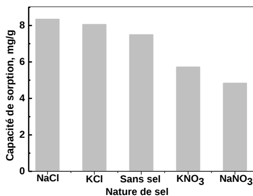
Figure 131: Effet de la nature du sel ajouté sur la capacité de rétention des ions Pb(II) par la résine Lewatit 214, pH \approx 4,0-5,0, m_{\text{résine}} = 0,050 g, V_{\text{aq}} = 5 mL, [\text{Pb(II)}] = 10^{-3} M, \varnothing = 250 tpm.
