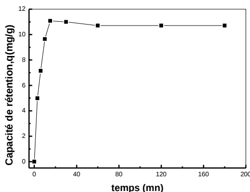
Figure 120: Effet du temps de contact sur la capacité de rétention des ions \text{Pb}^{2+} par la résine Lewatit TP 214, [\text{Pb(II)}]_0 = 1,0 \cdot 10^{-3} \text{ M} , m = 0.050 \text{ g} , V = 5 \text{ mL} , \text{pHi} = 4,5 , \emptyset = 250 \text{ tpm} .
