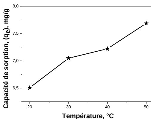
Figure 61 : Effet de la température sur la capacité de sorption de Pb(II) par la Lewatit TP 207, [Pb(II)]_i = 5.10^{-4} mol/L, m = 0,0600 g, V = 5 mL, pHi \approx 1,3 , \emptyset = 250 tpm
