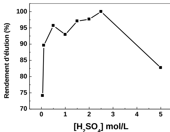
Figure 48: Effet de la concentration de l'éluant sur le rendement de la désorption du \text{La(III)} retenu par la résine Lewatit TP 260, V_{\text{acide sulfurique}} = 5 \text{ ml} , m_{\text{résine chargée}} = 0,100 \text{ g} , t = 60 \text{ min} , \varnothing = 250 \text{ tpm}
