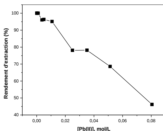
Figure 77 : Effet de la concentration initiale du Pb(II) sur le rendement de sa sorption par la résine Lewatit TP 260, m = 0.0600 g, V_{\text{sol}} = 5 mL, t_{\text{agitation}} = 15 mn, \varnothing = 250 tpm
