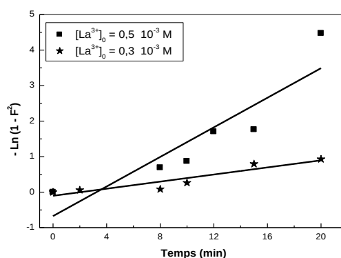
Figure 13: Application du modèle de diffusion intra-particulaire à la cinétique de sorption des ions La^{3+} sur la Lewatit TP 207, m = 0.1000 g, V = 5 ml, pH = 3,46 , \varnothing = 250 tpm
