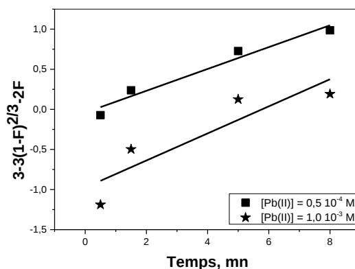
Figure 88: Modèle de diffusion par réaction chimique appliqué à la cinétique de sorption des ions Pb(II) sur la Lewatit TP 260, m = 0,0600 g, V = 5 ml, \text{pH} = 5 , \varnothing = 250 tpm
