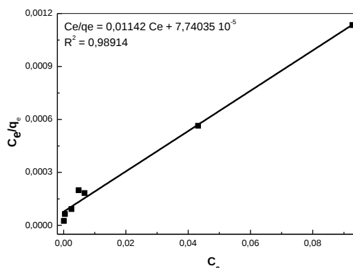
Figure 108 : Application du modèle de Langmuir pour l'extraction de Cd(II) par la Lewatit TP 214, V = 5,0 mL, m = 0.0300 g, pH_i = 5,0 , \emptyset = 250 tpm.
