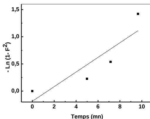
Figure 124: Modèle de diffusion intra-particulaire appliqué à la cinétique de sorption des ions \text{Pb}^{2+} sur la résine Lewatit TP214, [\text{Pb(II)}]_0 = 1,0 \cdot 10^{-3} \text{ M} , m = 0.050 \text{ g} , V = 5 \text{ mL} , \text{pHi} = 4,5 , \emptyset = 250 \text{ tpm} .
