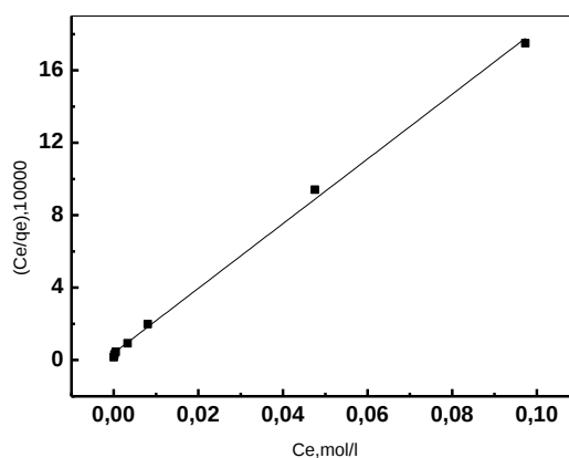
Figure 128: Modèle de Langmuir appliqué à l'extraction des ions Pb(II) par la Lewatit TP 214, \text{pH}_i = 4,5 , m = 0,0500 g, V = 5 mL, t = 30 mn, \varnothing = 250 tpm.
