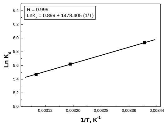
Figure 83: Evolution de \ln K_d en fonction de 1/T pour l'extraction de Pb(II) par la Lewatit TP 260, [Pb(II)]_i = 5.10^{-4} mol/L, m = 0,0600 g, V = 5 mL, pH_i \approx 1,15 , \emptyset = 250 tpm
