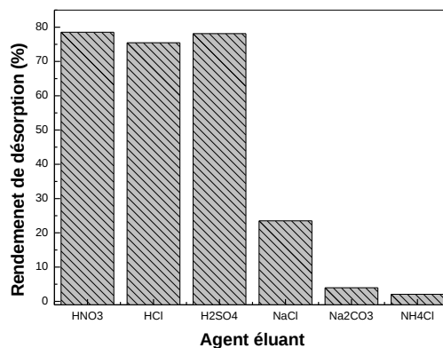
Figure 24: Effet de la nature de l'éluant sur le rendement de l'élution de La(III) à partir de la Lewatit TP 207 chargée en métal, V_{\text{Eluant}} = 5,0 \text{ mL} , m_{\text{(résine saturée en La(III))}} = 0,100 \text{ g} , \emptyset = 250 \text{ tpm}
