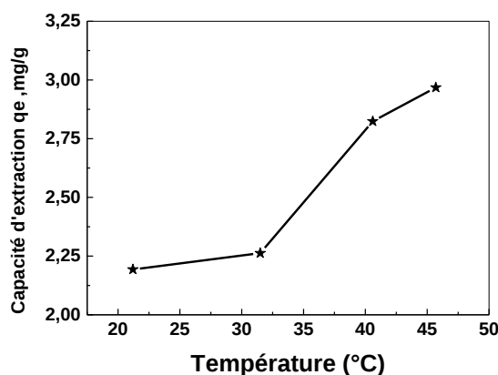
Figure 45 : Effet de la température sur la capacité d'extraction de \text{La}^{3+} par la Lewatit TP 260, [\text{La}^{3+}]_i = 5.10^{-4} mol/L, m = 0,1000 g, V = 5 mL, \text{pH}_i \approx 5,19 , \varnothing = 250 tpm
