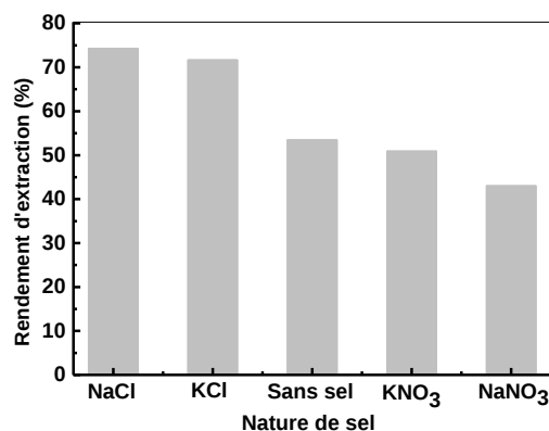
Figure 130: Effet de la nature du sel ajouté sur le rendement d'extraction des ions Pb(II) par la résine Lewatit 214, pH \approx 4,0-5,0, m_{\text{résine}} = 0,050 g, V_{\text{aq}} = 5 mL, [\text{Pb(II)}] = 10^{-3} M, \varnothing = 250 tpm.
