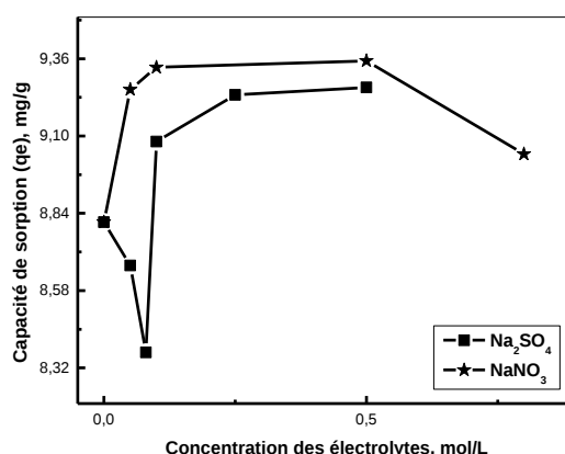
Figure 80 : Effet de l'ajout d'un sel sur la capacité de sorption de Pb(II) par la Lewatit TP 260, [Pb(II)]_0 = 5,0 \cdot 10^{-4} M, V = 5 mL, m = 0,0600 g, t_{agitation} = 15 mn, \varnothing = 250 tpm
