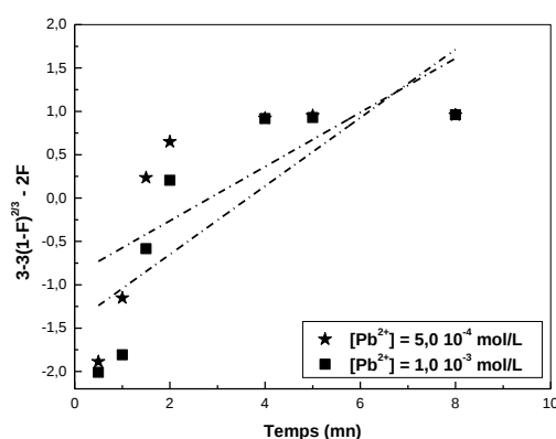
Figure 68: Modèle de diffusion par réaction chimique appliqué à la cinétique de sorption des ions Pb(II) sur la Lewatit TP 207, m = 0,0600 g, V = 5 ml, \text{pH} = 4.82 , \varnothing = 250 tpm
