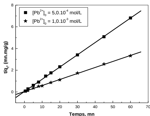
Figure 85: Application du modèle de pseudo-second ordre à la cinétique de sorption des ions Pb(II) par la résine Lewatit TP 260, m = 0,0600 g, V_{\text{sol}} = 5 mL, \text{pH}_{\text{initial}} \approx 5,0 , \emptyset = 250 tpm
