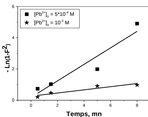
Figure 87: Modèle de diffusion intra-particulaire appliqué à la cinétique de sorption des ions Pb(II) sur la résine Lewatit TP 260, m = 0.0600 g, V = 5 ml, pH = 5 , \emptyset = 250 tpm
