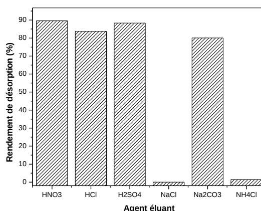
Figure 47: Effet de la nature de l'éluant sur le rendement d'élution des ions \text{La(III)} retenus par la résine Lewatit TP 260, V_{\text{Eluant}} = 5,0 mL, m_{\text{résine saturée en La(III)}} = 0,100 g, \varnothing = 250 tpm
