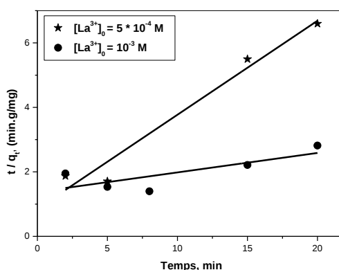
Figure 33: Application du modèle de pseudo-second ordre à la cinétique de sorption des ions \text{La}^{3+} par la résine Lewatit TP 260, m = 0,1000 g, V_{\text{sol}} = 5 mL, \text{pH}_i \approx 5.19 , \emptyset = 250 tpm
