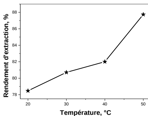
Figure 60 : Effet de la température sur le rendement de l'extraction de Pb(II) par la Lewatit TP 207, [Pb(II)]_i = 5.10^{-4} mol/L, m = 0,0600 g, V = 5 mL, pHi \approx 1,3 , \emptyset = 250 tpm
