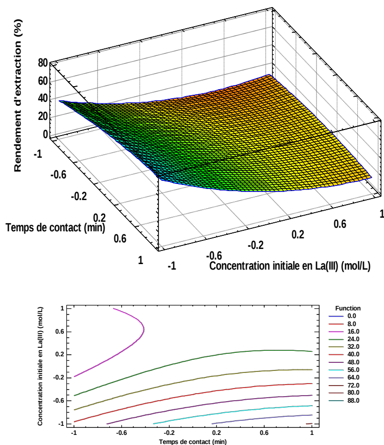
Figure 136 : La surface de réponse et la courbe iso-réponse montrant l'effet de temps de contact et de la concentration en métal et leur effet mutuel sur le rendement d'extraction avec X_2 = 0
