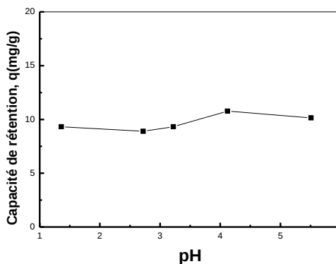
Figure 118 : Effet du pH de solution sur La capacité de rétention des ions de \text{Pb}^{2+} par la résine Lewatit TP 214, [\text{Pb}]_i = 1,0 \cdot 10^{-3} \text{ M} , m = 0,050 \text{ g} , V = 5 \text{ mL} , \varnothing = 250 \text{ tpm}
