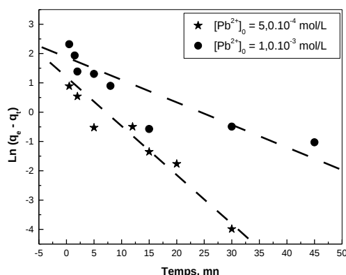
Figure 84: Application du modèle de pseudo-premier ordre à la cinétique de sorption des ions Pb(II) par la résine Lewatit TP 260, m = 0,0600 g, V_{sol} = 5 mL, pH_{initial} \approx 5,0 , \emptyset = 250 tpm
