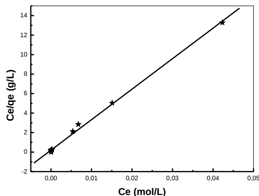
Figure 89: Modèle de Langmuir appliqué à l'extraction de Pb(II) par la résine Lewatit TP 260, m = 0.0600 \text{ g} , V_{\text{sol}} = 5 \text{ mL} , t = 15 \text{ mn} , \varnothing = 250 \text{ tpm}
