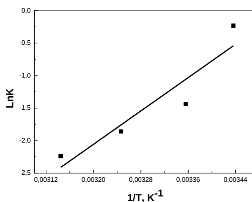
Figure 116 : Evolution de \ln K_d en fonction de 1/T pour l'extraction de Cd(II) par la Lewatit TP 214, [Cd(II)]_i = 1,0 \cdot 10^{-3} mol/L, pH_i = 5,0 , m_{résine} = 0,050 g, V_{aq} = 5,0 mL, t = 60 mn, \varnothing = 250 tpm
