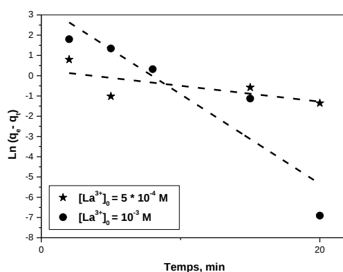
Figure 32: Application du modèle de pseudo-premier ordre à la cinétique de sorption des ions \text{La}^{3+} par la résine Lewatit TP 260, m = 0,1000 g, V_{\text{sol}} = 5 mL, \text{pH}_{\text{initial}} \approx 5.19 , \emptyset = 250 tpm
