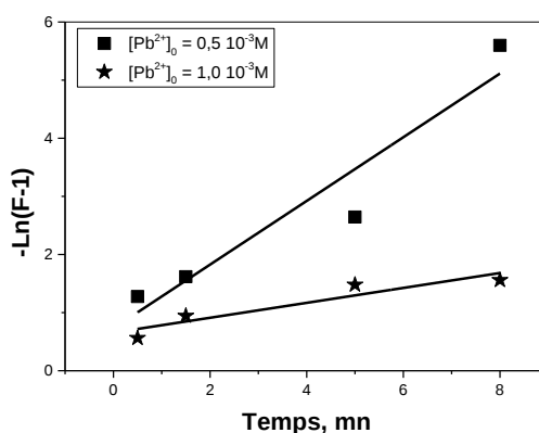
Figure 86: Modèle de diffusion externe appliqué à la cinétique de sorption des ions Pb(II) sur la résine Lewatit TP 260, m = 0,0600 g, V = 5 ml, pH_i = 5,0 , \emptyset = 250 tpm
