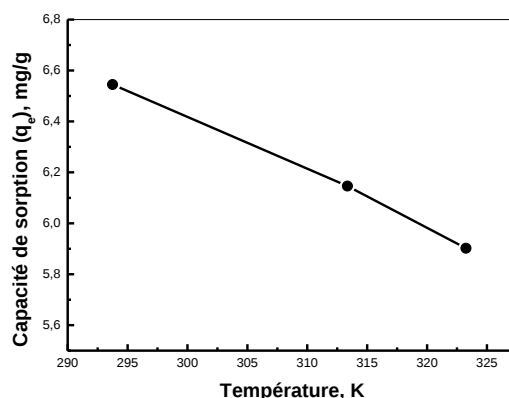
Figure 82 : Effet de la température sur la capacité de sorption de Pb(II) par la Lewatit TP 260, [\text{Pb(II)}]_i = 5.10^{-4} mol/L, m = 0,0600 g, V = 5 mL, \text{pHi} \approx 1,15 , \varnothing = 250 tpm
