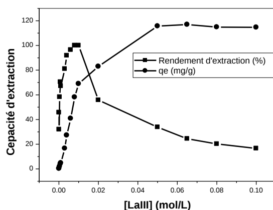
Figure 15 : Effet de la concentration initiale du La^{3+} sur la capacité d'extraction de la résine Lewatit TP 207, m = 0.1000 g, V_{sol} = 5 mL, t_{agitation} = 20 mn, \varnothing = 250 tpm
