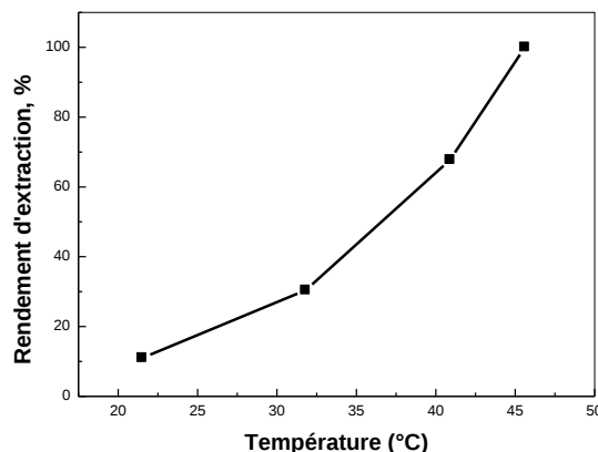
Figure 21 : Effet de la température sur le rendement d'extraction de \text{La}^{3+} par la Lewatit TP 207, [\text{La}^{3+}]_i = 5.10^{-4} mol/L, m = 0,100 g, V = 5 mL, \text{pHi} \approx 3,46 , \varnothing = 250 tpm
