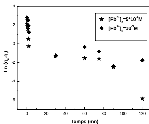
Figure 63: Application du modèle de pseudo-premier ordre à la cinétique de sorption des ions Pb(II) par la résine Lewatit TP 207, m = 0,0600 g, V_{\text{sol}} = 5\text{ml} , \varnothing = 250 tpm.
