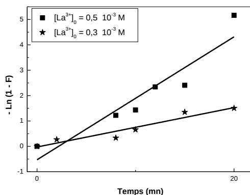
Figure 12: Application du modèle de diffusion externe à la cinétique de sorption des ions La^{3+} sur la résine Lewatit TP 207, m \approx 0,100 g, V = 5 ml, pH_i = 3,46 , \varnothing = 250 tpm
