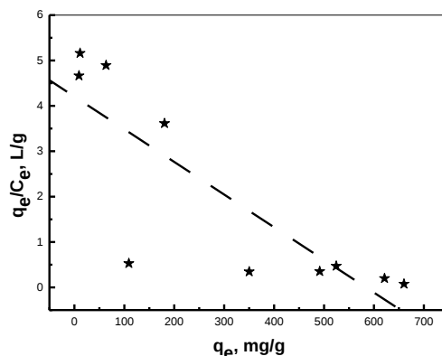
Figure 91: Modèle de Elovich appliqué à l'extraction de Pb(II) par la résine Lewatit TP 260, m = 0.0600 g, V_{sol} = 5 mL, t = 15 mn, \varnothing = 250 tpm
