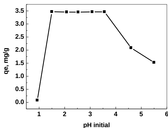
Figure 4 : Effet du pH de la phase aqueuse sur la capacité de sorption du La(III) par la Lewatit TP 207, C_0 = 5 \cdot 10^{-4} mol/L, m \approx 0.1000 g, t_{\text{agitation}} = 180 mn, \varnothing = 250 tpm
