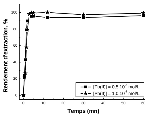
Figure 54 : Effet du temps de contact sur le rendement d'extraction de Pb(II) par la Lewatit TP 207, m \approx 0.0600 \text{ g} , pH_i = 4.82 , \varnothing = 250 \text{ tpm} .
