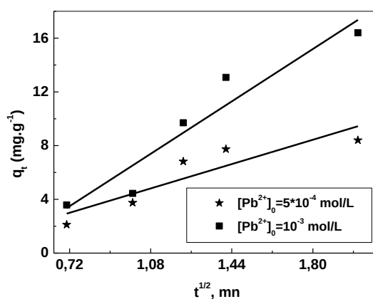
Figure 65 : Application du modèle de diffusion intra-particulaire à la cinétique de sorption des ions Pb(II) par la résine Lewatit TP 207, m = 0,0600 g, V_{sol} = 5 ml, \emptyset = 250 tpm
