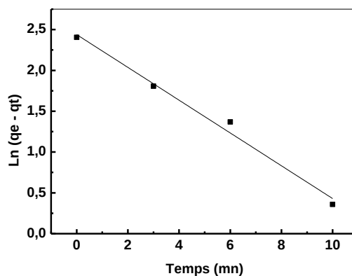
Figure 121 : Application du modèle de pseudo-premier ordre à la cinétique de sorption des ions Pb^{2+} par la Lewatit TP 214, [Pb(II)]_0 = 1,0 \cdot 10^{-3} M, m = 0.050 g, V = 5 mL, pH_i = 4,5 , \emptyset = 250 tpm
