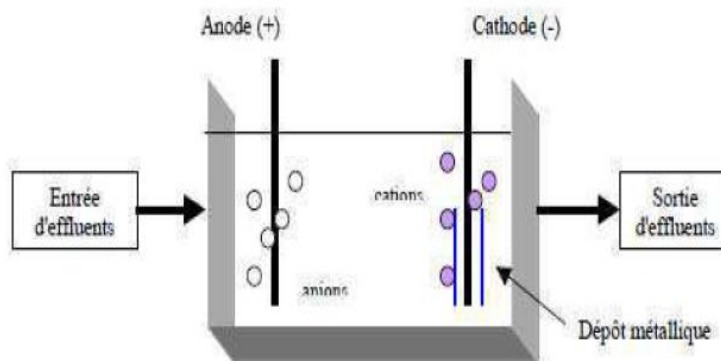
Figure 1 : Schéma d'une électrolyse simple [6].
