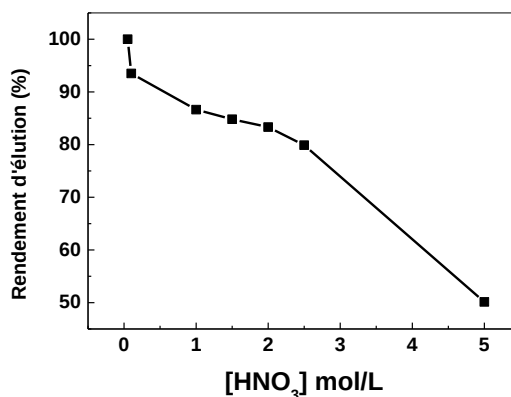
Figure 25: Effet de la concentration de l'éluant sur l'élution de La(III) à partir de la Lewatit TP 207 chargée en métal, V_{\text{acide nitrique}} = 5,0 \text{ mL} , m = 0,100 \text{ g} , \emptyset = 250 \text{ tpm}
