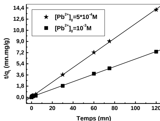
Figure 64: Application du modèle de pseudo-second ordre à la cinétique de sorption des ions Pb(II) par la résine Lewatit TP 207, m = 0,0600 g, V_{sol} = 5 ml, \emptyset = 250 tpm
