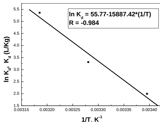
Figure 23: Evolution de \ln K_d en fonction de 1/T lors de l'extraction de \text{La}^{3+} par la Lewatit TP 207, [\text{La(III)}]_i = 5.10^{-4} mol/L, m = 0,1000 g, V = 5 mL, \text{pHi} \approx 3,46 , \varnothing = 250 tpm
