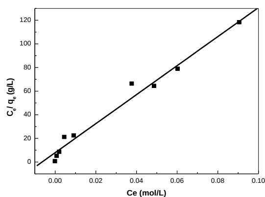
Figure 39 : Modèle de Langmuir appliqué à l'extraction de La(III) par la résine Lewatit TP 260, m = 0,1000 g, V_{sol} = 5 mL, t_{agitation} = 30 mn, \varnothing = 250 tpm
