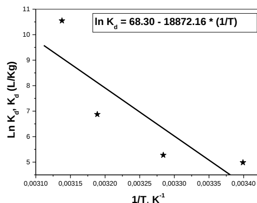
Figure 46: Evolution de \ln K_d en fonction de 1/T pour l'extraction de \text{La}^{3+} par la Lewatit TP 260, [\text{La(III)}]_i = 5.10^{-4} mol/L, m = 0,1000 g, V = 5 mL, \text{pHi} \approx 5,19 , \varnothing = 250 tpm
