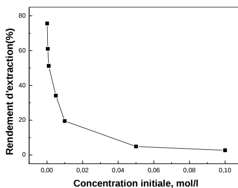
Figure 126: Influence de la concentration initiale en Pb(II) sur le rendement d'extraction des ions de Pb^{2+} par la résine Lewatit TP 214, pH_i = 4,5 , m = 0,050 g, V = 5 mL, t = 30 mn, \emptyset = 250 tpm.
