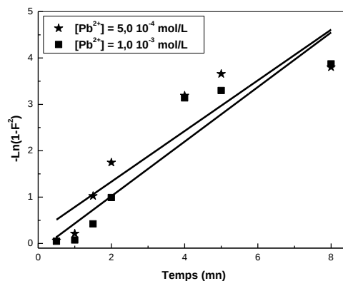
Figure 67: Modèle de diffusion intra-particulaire appliqué à la cinétique de sorption du Pb(II) sur la résine Lewatit TP 207, m = 0.0600 g, V = 5 ml, \text{pH} = 4.82 , \varnothing = 250 tpm
