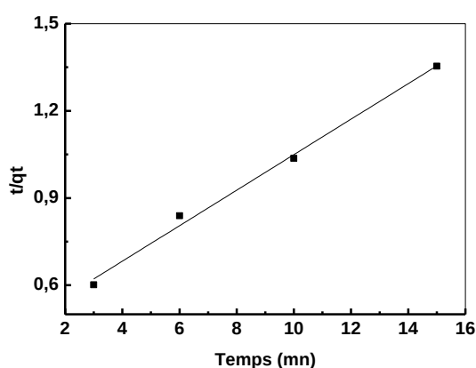
Figure 122: Application du modèle cinétique du pseudo-second ordre à la cinétique de sorption des ions Pb^{2+} par la Lewatit TP 214, [Pb(II)]_0 = 1,0 \cdot 10^{-3} M, m = 0.050 g, V = 5 mL, pH_i = 4,5 , \emptyset = 250 tpm
