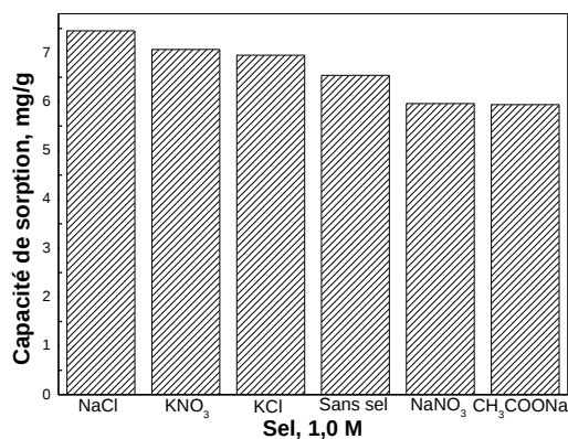
Figure 111 : Effet de la nature du sel ajouté sur la capacité d'extraction de Cd(II) par la Lewatit TP 214, m = 0,050 g, V = 5,0 mL, pH i = 5,0, [Cd 2+ ] = 1,0 10 -3 mol/L, t = 60 mn, Ø = 250 tpm
