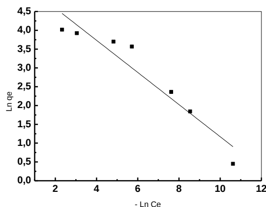
Figure 129: Modèle de Freundlich appliqué à l'extraction des ions Pb(II) par la Lewatit TP 214, \text{pH}_i = 4,5 , m = 0,0500 g, V = 5 mL, t = 30 mn, \varnothing = 250 tpm.
