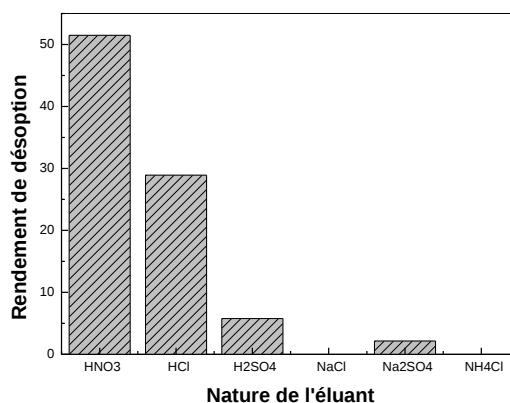
Figure 72: Effet de la nature de l'éluant sur le rendement de désorption des ions Pb 2+ à partir de la Lewatit TP 207 chargé en métal, V éluant = 5,0 mL, m chargée en plomb = 0,06 g, Ø = 250 tpm
