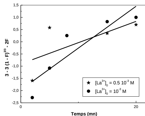
Figure 37: Modèle de diffusion par réaction chimique appliqué à la cinétique de sorption des ions \text{La}^{3+} sur la résine Lewatit TP 260, m = 0.1000 g, V = 5 ml, \text{pH} = 5,19 , \emptyset = 250 tpm.
