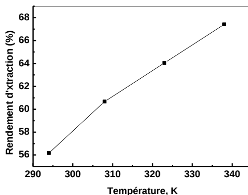
Figure 132: Effet de la température sur le rendement d'extraction de Pb(II) par la résine Lewatit TP 214, [\text{Pb(II)}]_i = 1,0 \cdot 10^{-3} \text{ mol/L} , m = 0,050 \text{ g} , V = 5 \text{ mL} , \text{pH}_i = 4,5 , \emptyset = 250 \text{ tpm} .
