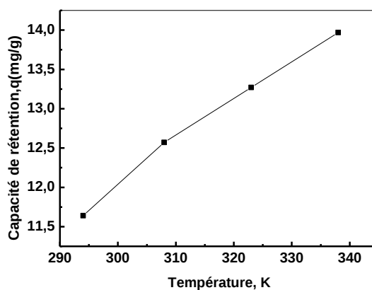
Figure 133: Effet de la température sur la capacité de rétention de Pb(II) par la résine Lewatit TP 214, [\text{Pb(II)}]_i = 1,0 \cdot 10^{-3} \text{ mol/L} , m = 0,050 \text{ g} , V = 5 \text{ mL} , \text{pH}_i = 4,5 , \emptyset = 250 \text{ tpm} .
