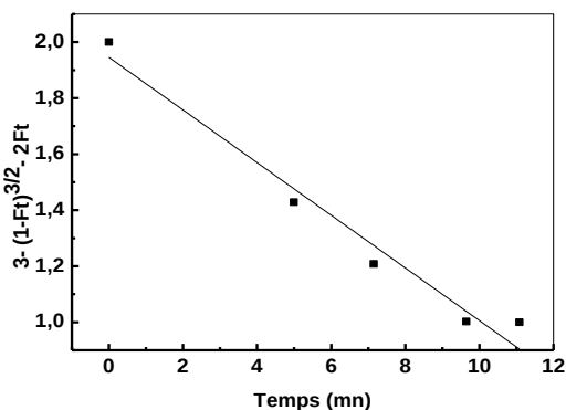
Figure 125: Modèle de diffusion par réaction chimique appliqué à la cinétique de sorption des ions Pb^{2+} sur la résine Lewatit TP214, [Pb(II)]_0 = 1,0 \cdot 10^{-3} M, m = 0,0500 g, V = 5 mL, pH_i = 4,5 , \emptyset = 250 tpm.
