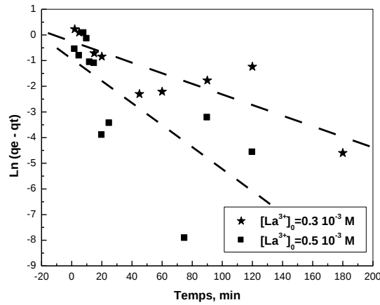
Figure 9: Application du modèle de pseudo-premier ordre à la cinétique de sorption des ions La(III) par la résine Lewatit TP207, m = 0,1000 g, V_{\text{sol}} = 5 mL, \text{pH}_{\text{initial}} \approx 3.49 , \varnothing = 250 tpm
