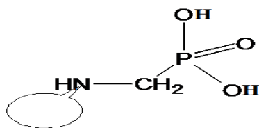
Styrène-divinylebenzène
