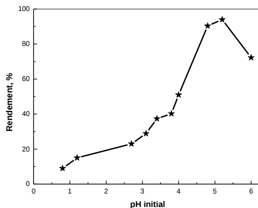
Figure 28 : Effet du pH initial de la phase aqueuse sur le rendement d'extraction de La(III) par la Lewatit TP 260, C_0 = 5 \cdot 10^{-4} mol/L, m \approx 0.1000 g, t_{\text{agitation}} = 180 mn, \varnothing = 250 tpm
