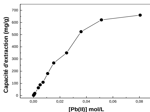
Figure 78 : Effet de la concentration initiale du Pb(II) sur la capacité de sa sorption par la résine Lewatit TP260, m = 0.0600 g, V_{\text{sol}} = 5 mL, t_{\text{agitation}} = 15 mn, \varnothing = 250 tpm
