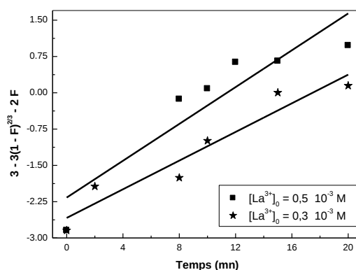
Figure 14: Application du modèle de diffusion par réaction chimique à la cinétique de sorption des ions La^{3+} par la Lewatit TP 207, m = 0.1000 g, V = 5 ml, pH = 3,46 , \varnothing = 250 tpm.
