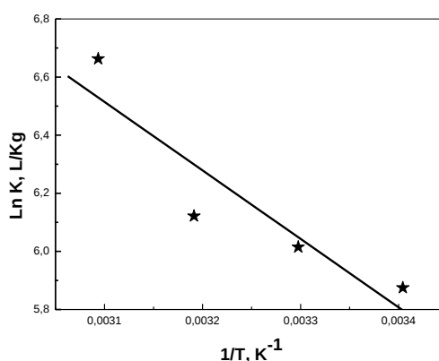
Figure 62: Evolution de \ln K_d en fonction de 1/T pour l'extraction de \text{Pb(II)} par la Lewatit TP 207, [\text{Pb(II)}]_i = 5.10^{-4} \text{ mol/L} , m = 0,0600 \text{ g} , V = 5 \text{ mL} , \text{pHi} \approx 1,3 , \emptyset = 250 \text{ tpm}
