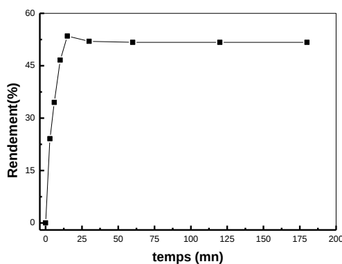
Figure 119: Effet du temps de contact sur le rendement d'extraction des ions \text{Pb}^{2+} par la résine Lewatit TP 214, [\text{Pb(II)}]_0 = 1,0 \cdot 10^{-3} \text{ M} , m = 0.050 \text{ g} , V = 5 \text{ mL} , \text{pHi} = 4,5 , \emptyset = 250 \text{ tpm} .
