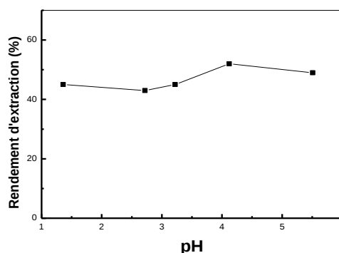
Figure 117: Effet du pH de la solution sur le rendement d'extraction des ions de \text{Pb}^{2+} par la résine Lewatit TP 214, [\text{Pb}]_i = 1,0 \cdot 10^{-3} \text{ M} , m = 0,050 \text{ g} , V = 5 \text{ mL} , \varnothing = 250 \text{ tpm}
