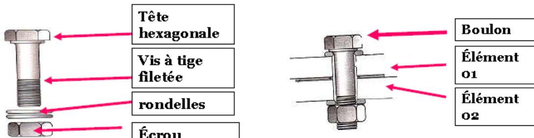
Figure 175: Assemblage par boulonnage Source : https://be-steel.eu/fr
