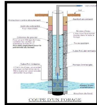
Figure 105 : Coupe d'un forage d'eau . Source : http://www.geotechsol.com/forages.php
