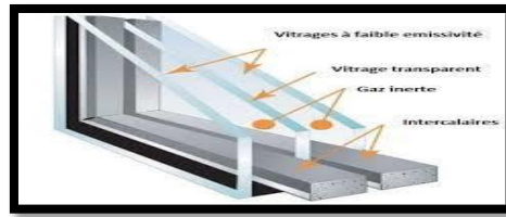
Figure191 : le triple vitrage
