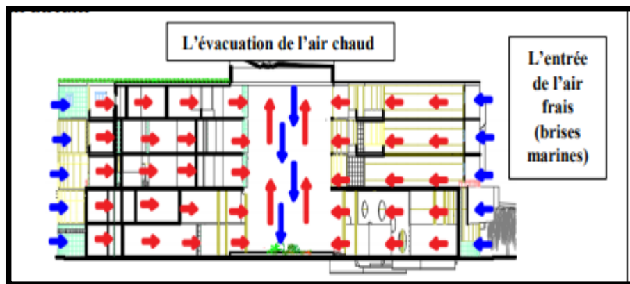
Figure 122 : figure 101 ventilation naturelle à travers le patio
