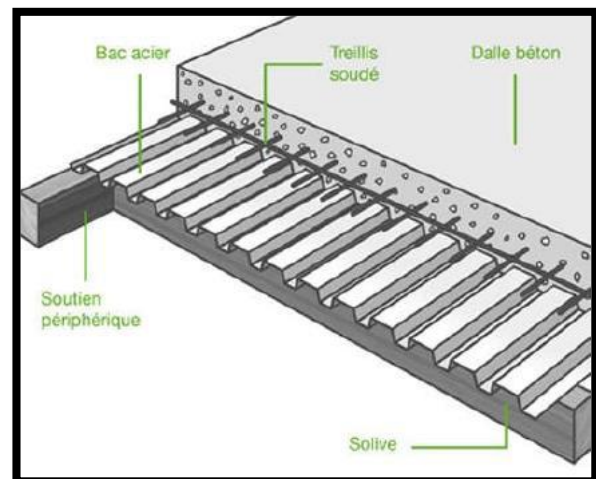
Figure 176: détail plancher collaborant.
