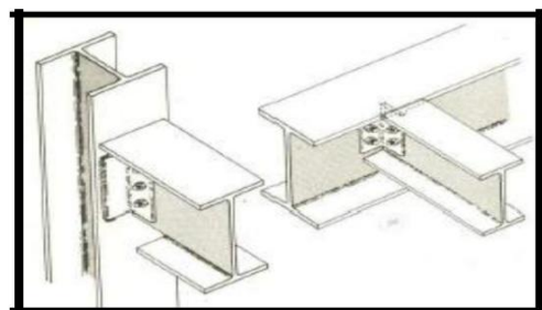
Figure 171: assemblage poteau-poutre métallique
