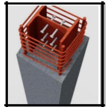
Figure 169: Exemple de poteau
