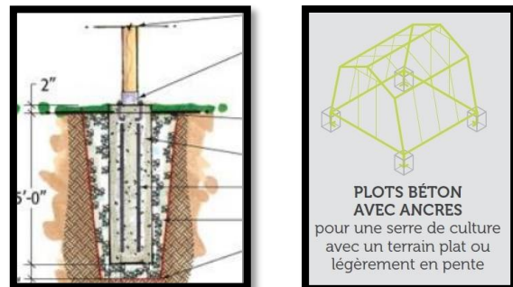
Figure 187: la fondation des serres, Source : https://www.invernaderosima.com/
