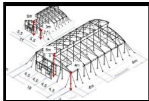
Figure 185: Structure des serres, Source : Auteur
