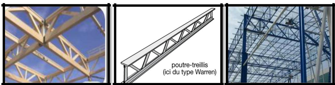
Figure 178: Poutre en treillis.
