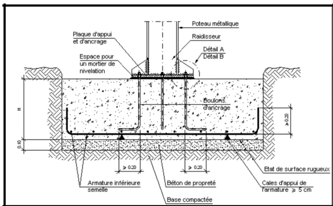
Figure 170 : Structure métallique. Profondeur de pénétration dans Fondation.
