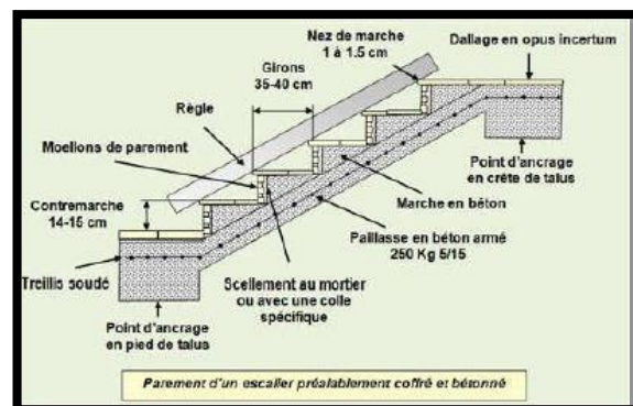
Figure 181 : Détail escalier en béton. Source : https://www.jardiniers
