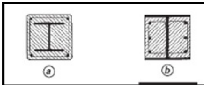
Figure 173 : types de poteau mixte
