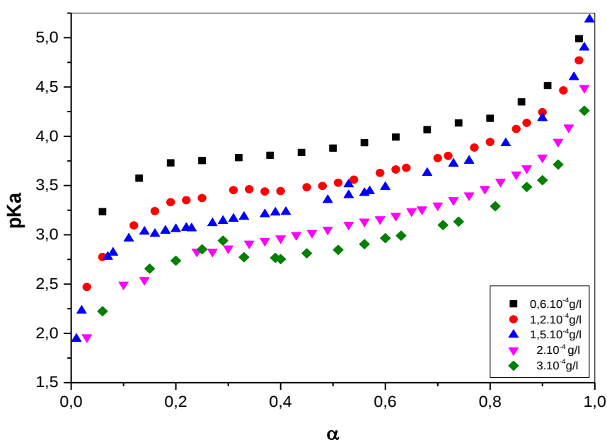
Figure IV.19: Variation du pKa en fonction de \alpha pour différentes concentrations du copolymère P4VPC 8 Br48.8% dans l'eau à 25°C
