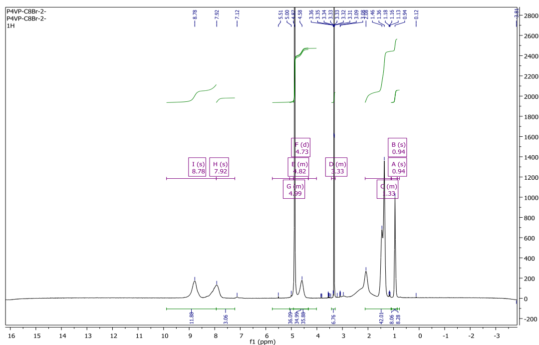
Figure III.11 : Spectre \text{RMN}^1\text{H} de copolymère \text{P4VPC}_8\text{Br}72\% dans le méthanol deutéré
