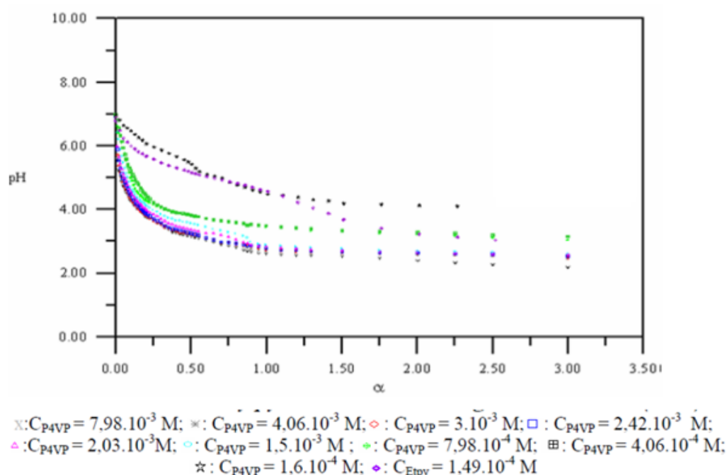
Figure IV.16: Variation du pH en fonction de \alpha pour différentes concentrations en P4VP et en 4-éthylpyridine dans le mélange eau-méthanol (50%) [37]
