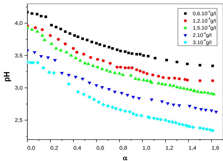
Figure IV.18: Titration potiométrique du P4VPC 8 Br 72% en fonction de \alpha dans l'eau à 25°C
