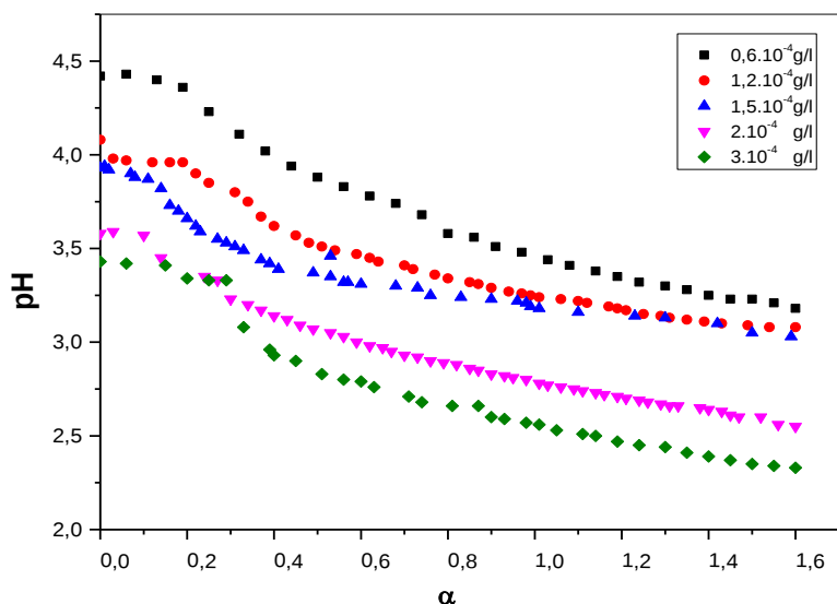
Figure IV.17: Titration potiométrique du P4VPC 8 Br 48.8% en fonction de \alpha dans l'eau à 25°C
