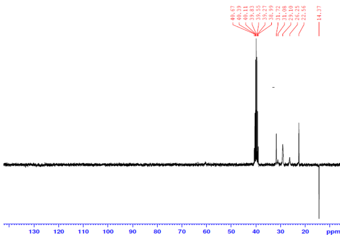
Figure III.14: Spectre \text{RMN}^{13}\text{C} de copolymère \text{P4VPC}_8\text{Br}_{20\%} dans le méthanol deutéré
