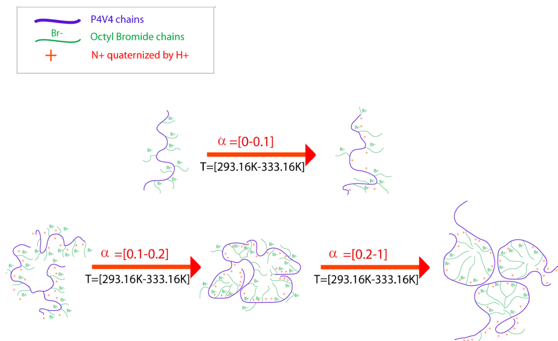
Figure IV.25 : Conformation de transition du Poly( N -octyl-4-vinylpyridinium bromide) en solution aqueuse avec HCl et l'effet thermodynamique [47]
