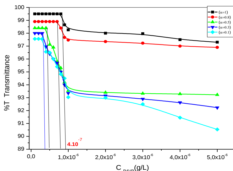
Figure IV.10: Variation% de la transmittance du P4VP en fonction de sa faible concentration C_{P4VP} à \alpha=1 ; \alpha=0.8 ; \alpha=0.5 ; \alpha=0.3 et \alpha=0.1
