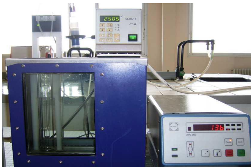
Figure II.3: Viscosimètre à capillaire type Ubbelhode
