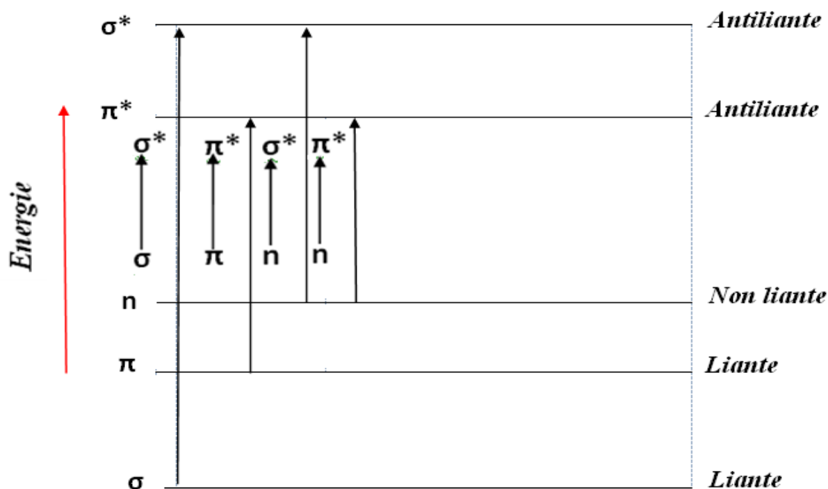
Figure II.1: Graphique comparatif rassemblant les transitions les plus souvent rencontrées dans les composés oxygénés ou azotés
