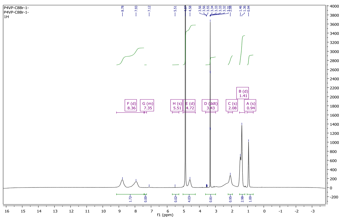
Figure III.12: Spectre \text{RMN}^1\text{H} de copolymère \text{P4VPC}_8\text{Br} 48.8\% dans le méthanol deutéré
