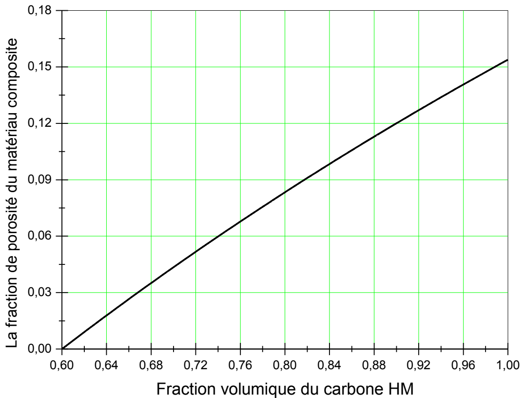
Figure 17 : variation de la porosité du composite l'époxyde/carbone HM en fonction de la fraction volumique du carbone HM
