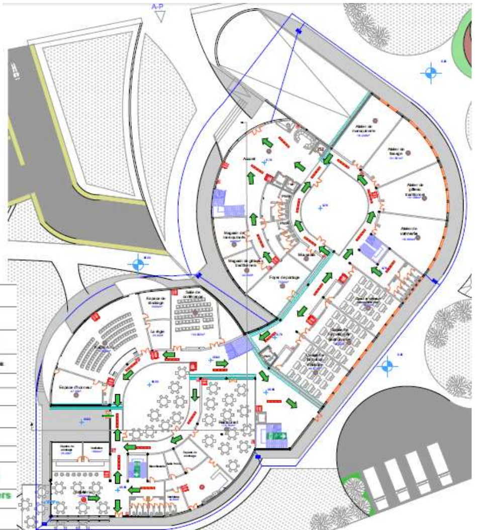
Figure 167: Plan d'incendie de RDC.
