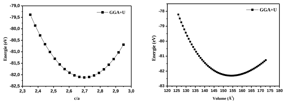
Figure III.14 : La variation de l'énergie totale en fonction du rapport c/a et le volume pour \text{TiO}_2 pur par l'approximation GGA+U.
