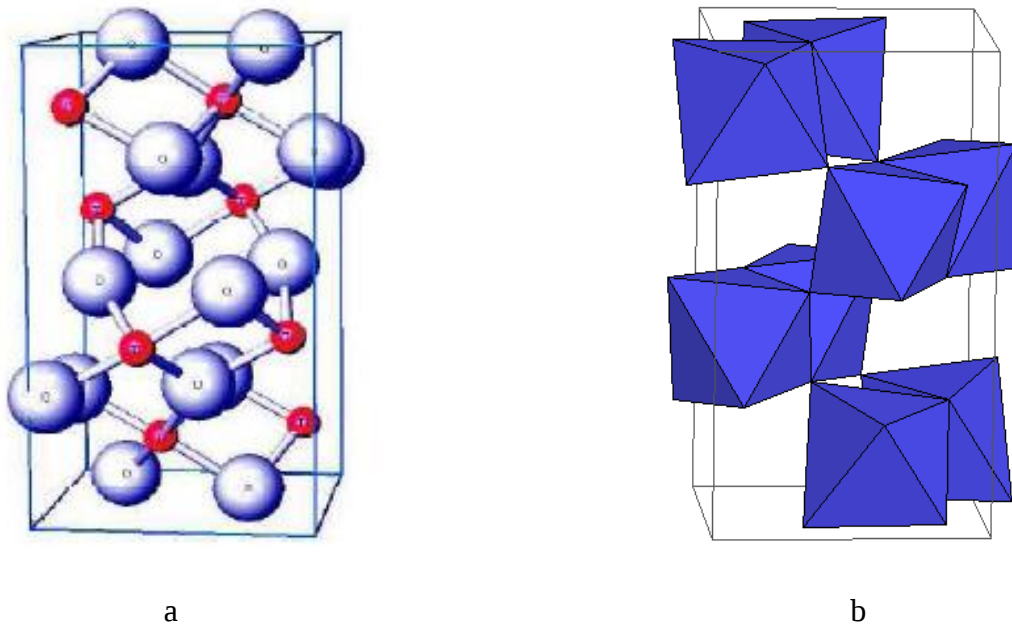
Figure I. 6 : (a) La structure cristalline de brookite, (b) : L'octaèdre de brookite [15].
