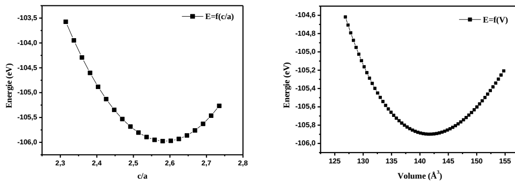
Figure III.5 : La variation de l'énergie totale en fonction du rapport ( c/a ) et le volume pour la phase anatase du \text{TiO}_2 .
