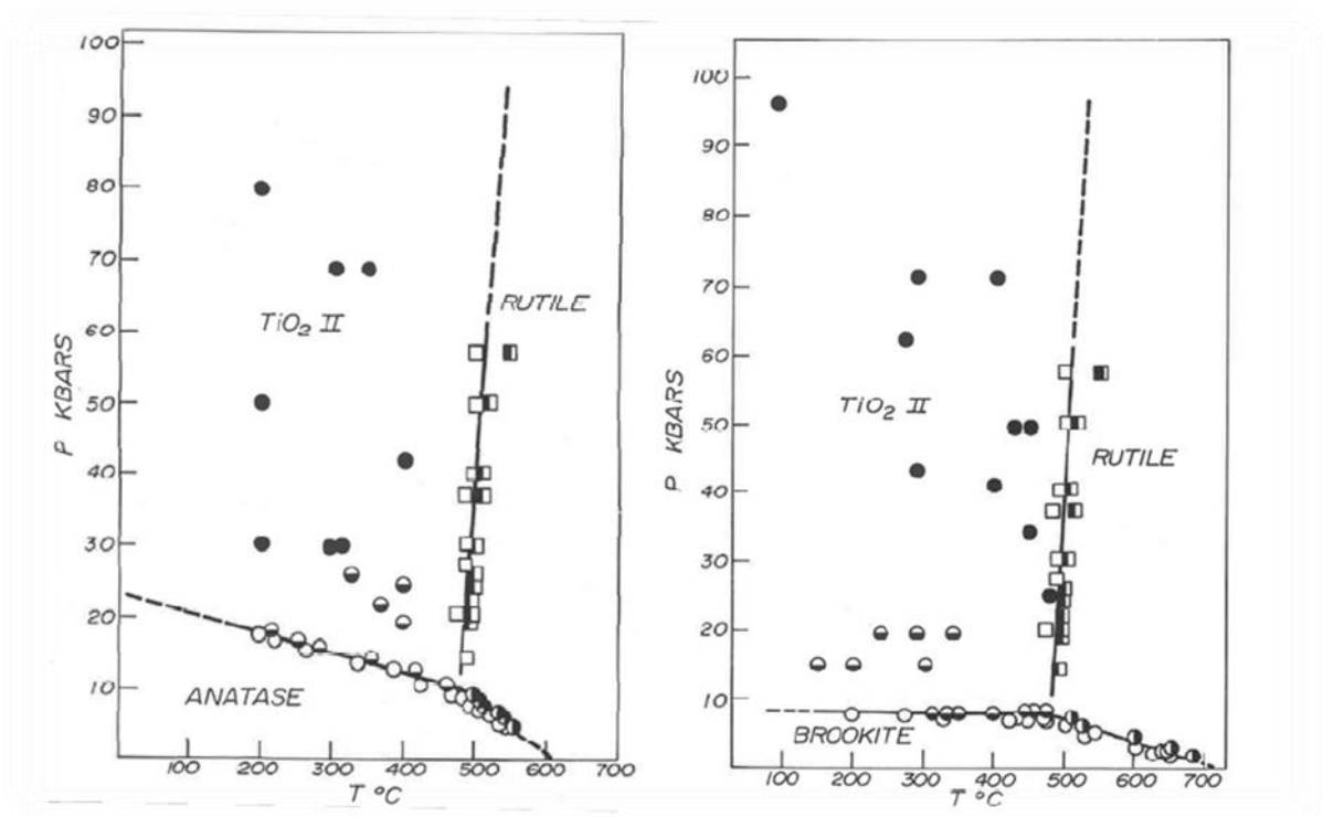
Figure I. 7 : Diagramme pression-température illustrant les conditions de transformations de (a) L'anatase et (b) de la brookite en rutile ou en \text{TiO}_2 de type II (type \alpha\text{-PbO}_2 ) [12].
