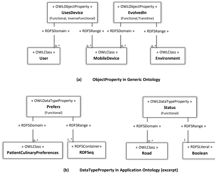
FIGURE 5.5 – Modélisation des propriétés des ontologies de contexte par ODM
