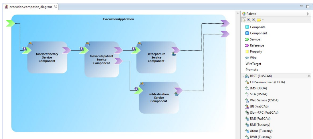
Figure 6.10: Architecture à base de composants de l'application SCA «Evacuation»
