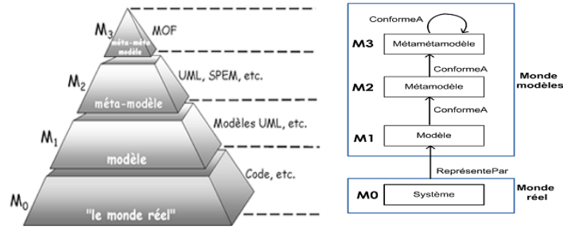
FIGURE 3.3 – Pyramide de modélisation à quatre niveaux
