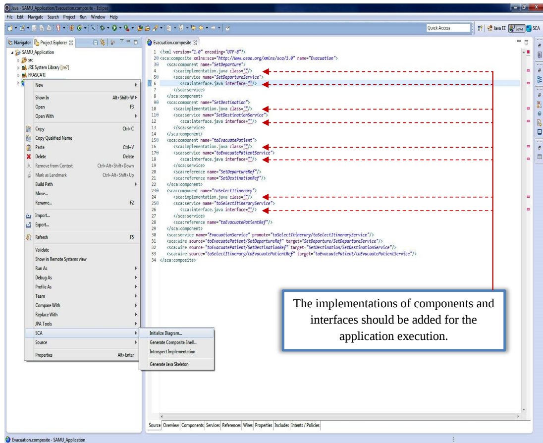
Figure 6.9: Le Langage de Description de l'Assemblage généré de Evacuation.composite dans Eclipse
