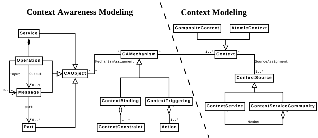
FIGURE 4.1 – Le métamodèle ContextUML
