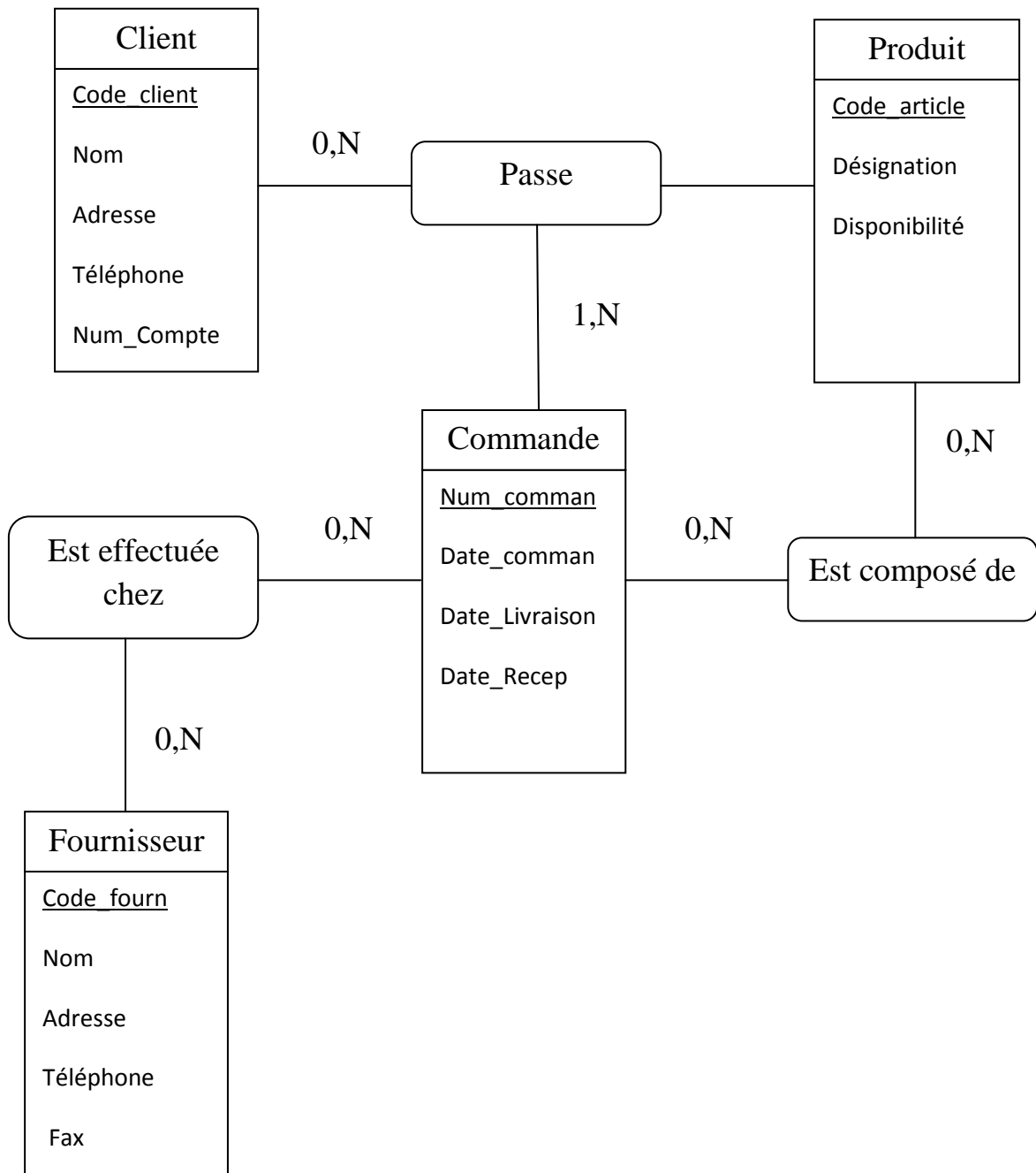
Figure 3-2 : MCD Général de la Gestion de Production
