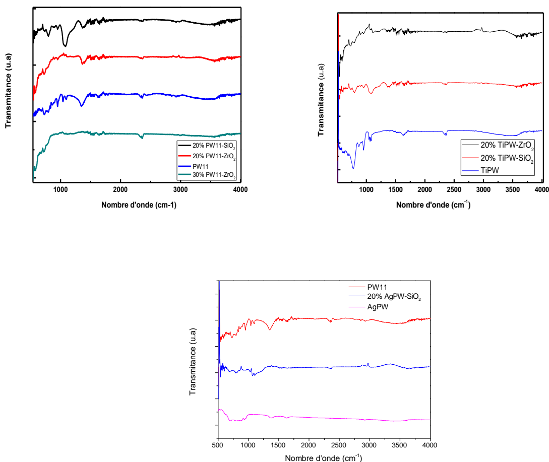
Figure III.4 : Spectres IRTF des matériaux préparés
