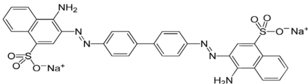
Figure I.4 : Structure du Rouge Congo.
