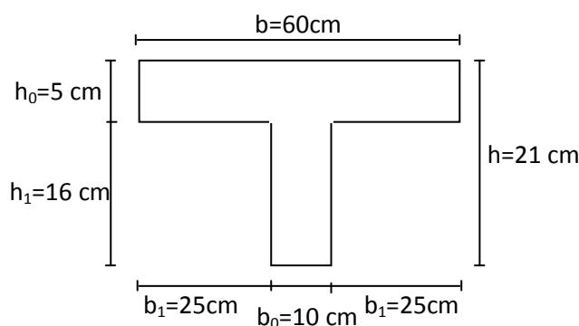
Figure 2.8 Dimensions des Poutrelles
