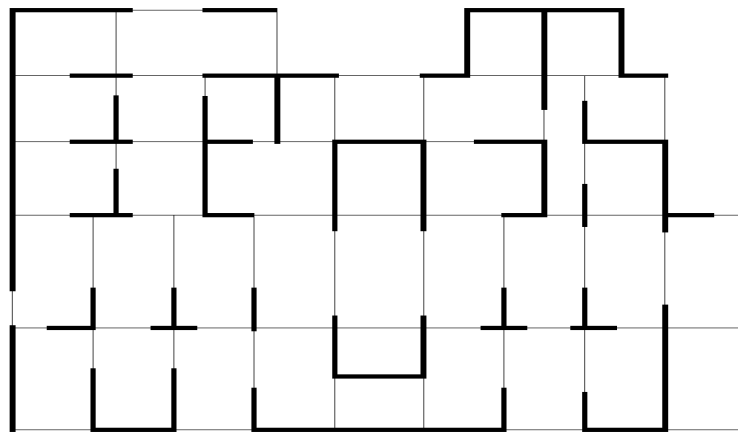
Figure 4.7 Deuxième disposition des voiles
