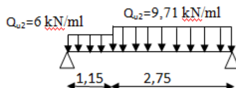
Figure 3.11 Chargement du premier type d'escalier à l'ELS
