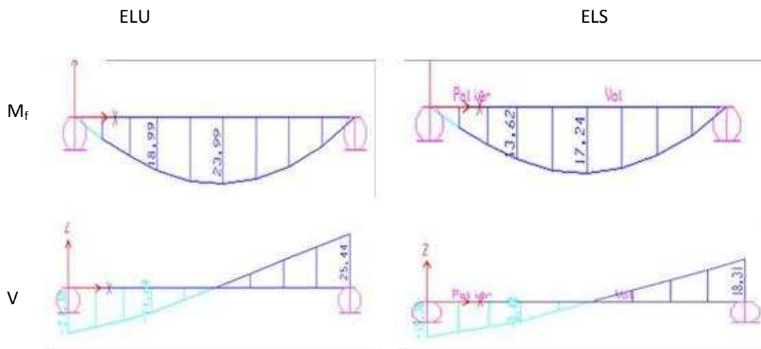
Figure 3.12 Diagramme des sollicitations pour l’escalier Type 1
