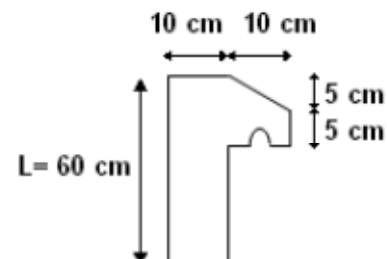
Figure 3.4 Coupe transversale de l'acrotère de l'acrotère
