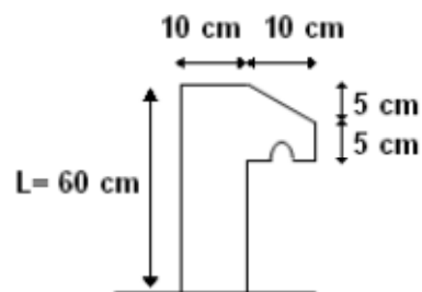
Figure 2.15 Coupe transversale de l'acrotère
