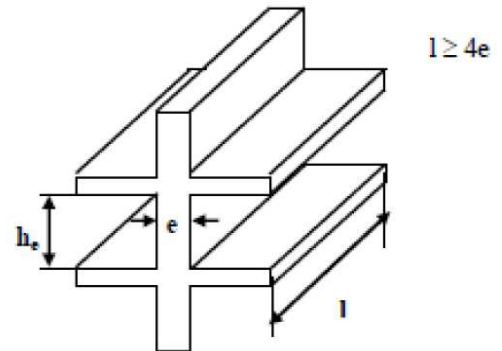
Figure 2.9 Coupe de voile 2 e solution
