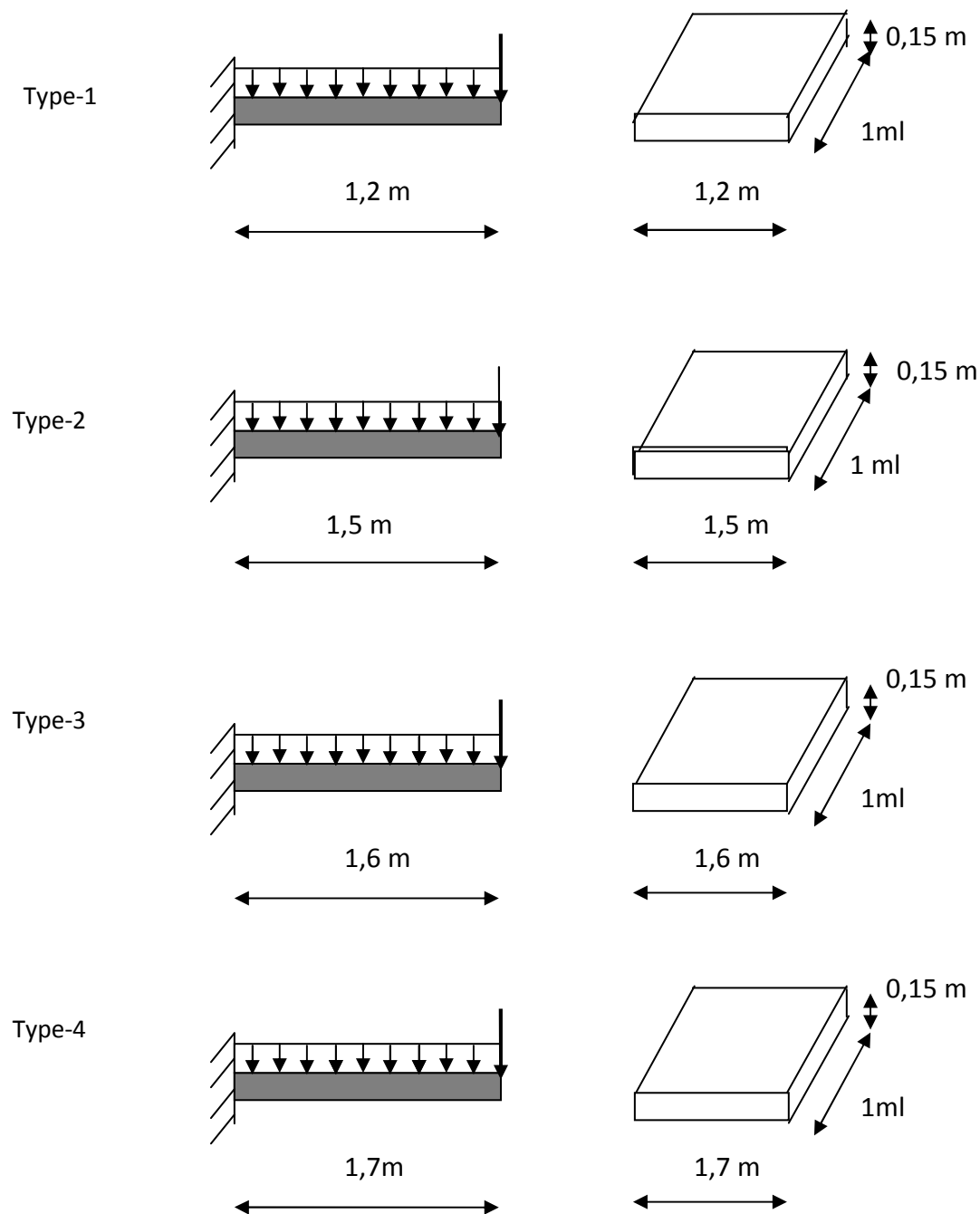
Figure 3.15 Schéma statique
