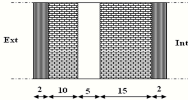
Figure 1.4 Coupe d'un mur extérieur
