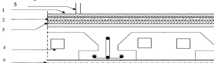
Figure 2.12 Elément constituant le plancher étage courant,
