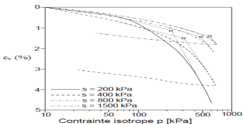
Figure 1.7 : Effets de la succion sur la compressibilité d'un limon de Jossigny compacté, (CUI et al, 1996)
