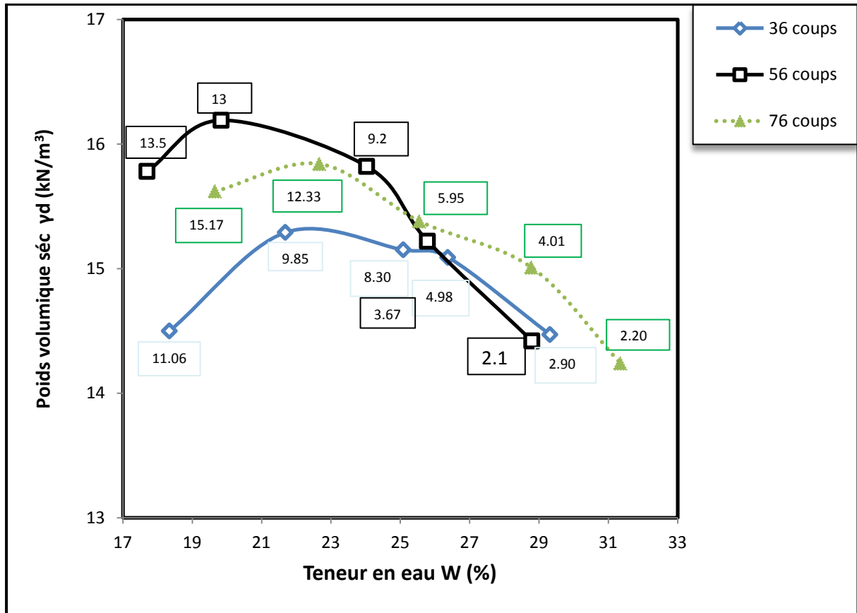
Figure 3.9 : Les Valeurs de l'essai Indice Portant Immédiate (IPI) mesurées présentées suivant les courbes de l'essai de compactage Proctor.
