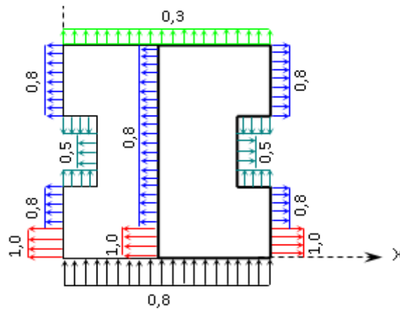
Figure II.9 : Coefficient de pression extérieure C_{pe}
