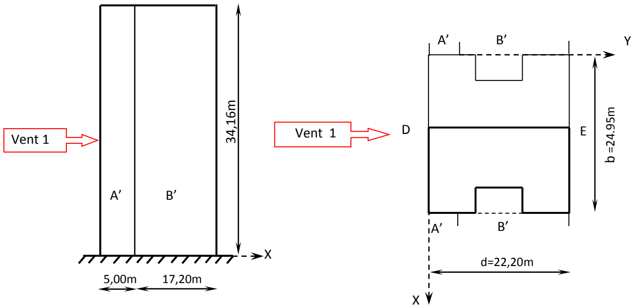
Figure II.8 : Découpage de zone de pression
