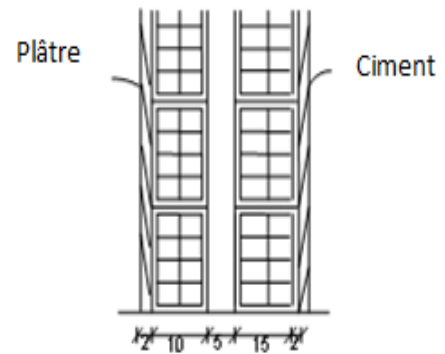
Figure II.2 : mur extérieure
