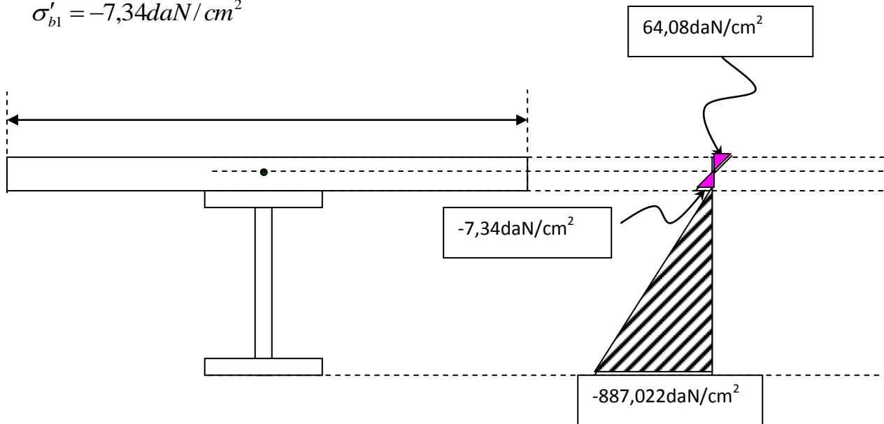
Figure V.2 : présentation des contraintes dans la section du plancher
