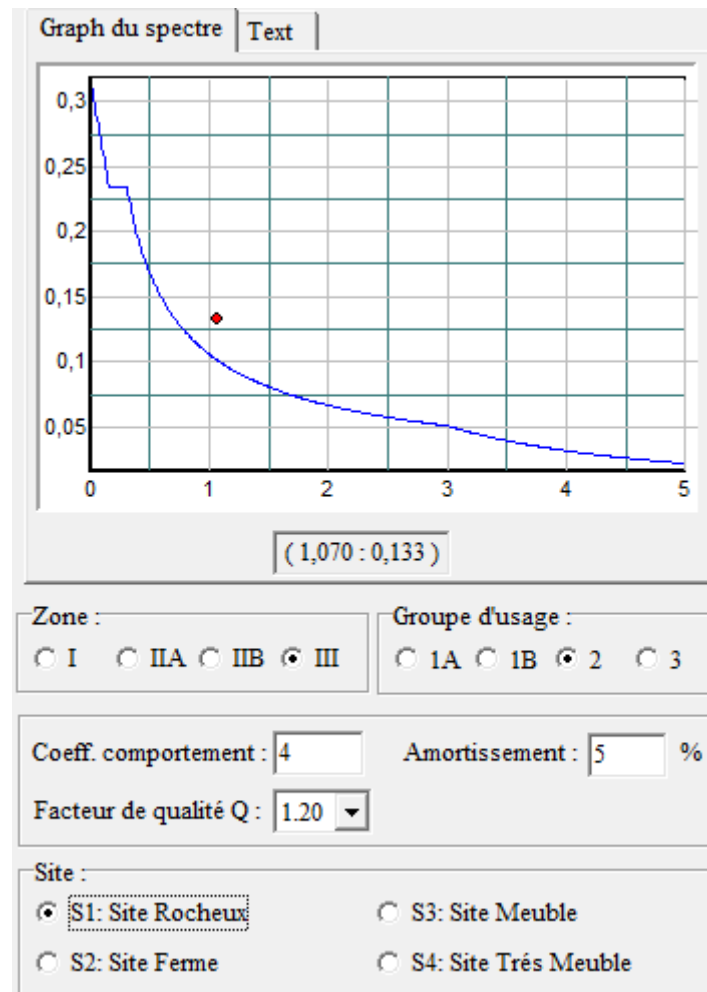
Figure IV.1 réponse spectral selon RPA
