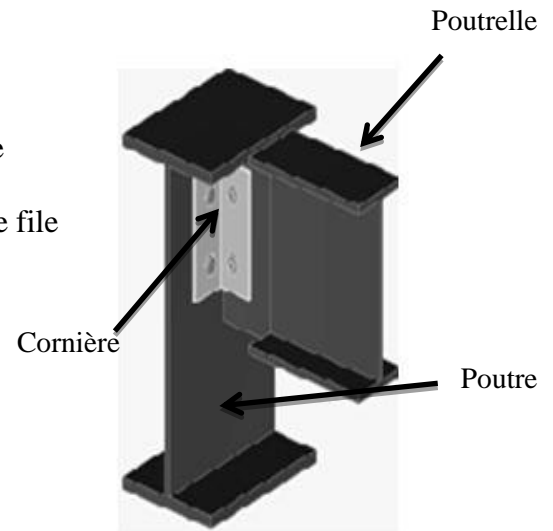
Figure VII.1. Assemblage poutrelle-poutre.
