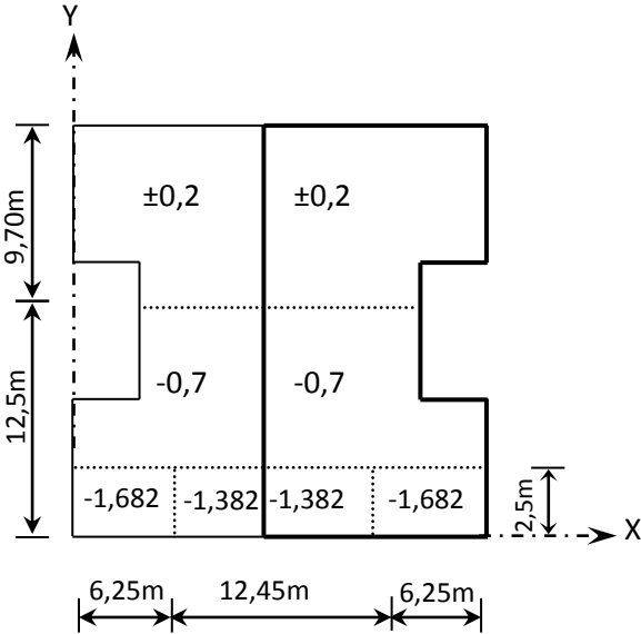
Figure II.10 : Coefficient « C pe » pour la toiture.
