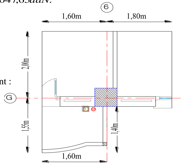
Figure III.4 : surface porté par poteau de rive
