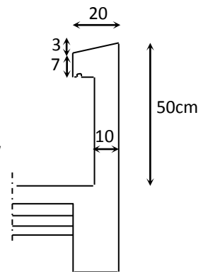
Figure II.3 : Acrotère
