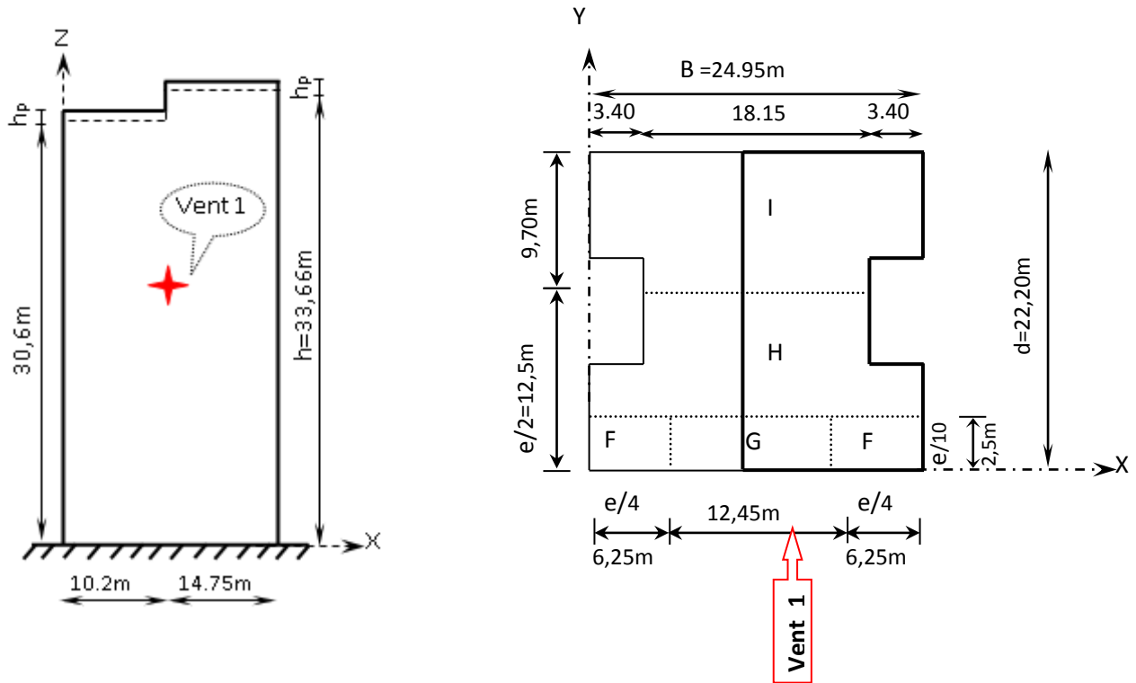
Figure II.9 : Découpage de zone de pression « toiture »
