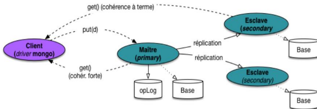
Figure III.10 : Un replica set dans MongoDB [28]
