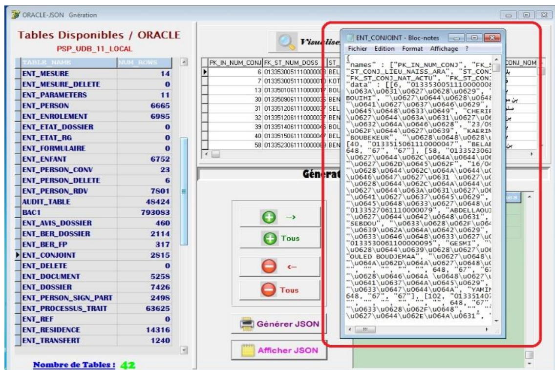
Figure III.37 : Un extrait d'un fichier JSON généré par oracle-json
