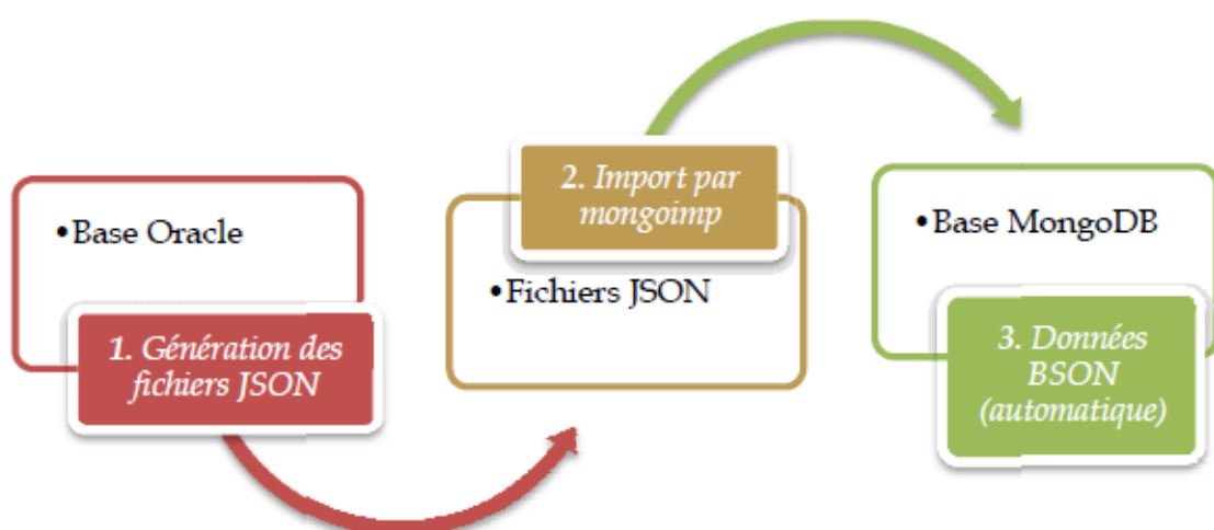
Figure III.32 : Schéma de l'approche de migration d'Oracle vers MongoDB
