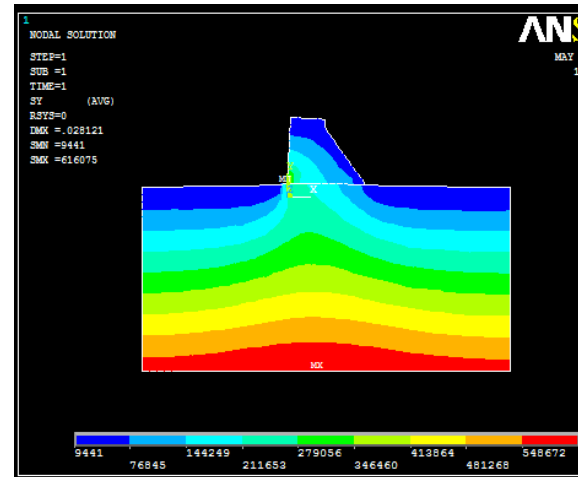
Fig. 3.83 : Champs des contraintes Barrage submersible BCR E_{\text{Fondation}} = 500.10^3 \text{ KPa}
