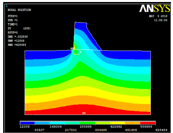
Fig. 3.61 : Champs des contraintes Barrage déversant BCR -E Fondation= 500.10^3 KPa
