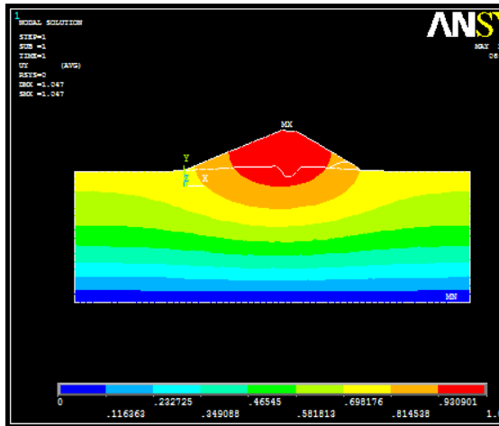
Fig. 3.30 : Champs des déformations Barrage en terre- E_{Fondation}=30.103 \text{ KPa}
