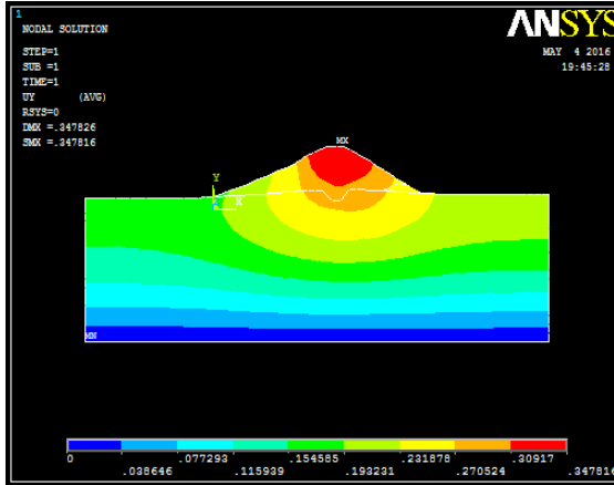
Fig. 3.44 : Champs des déformations Barrage en terre – Remplissage du lac E_{Fondation} = 100.10^3 \text{ KPa}
