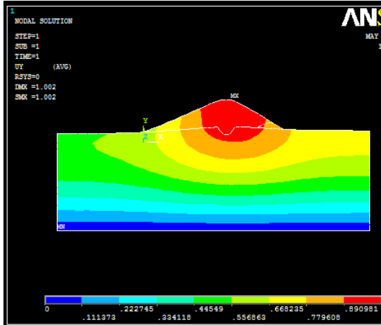
Fig. 3.40 : Champs des déformations Barrage en terre – Remplissage du lac E_{Fondation} = 30.10^3 \text{ KPa}
