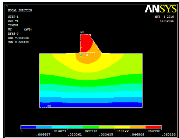
Fig. 3.80 : Champs des déformations Barrage submersible BCR E_{Fondation} = 200.10^3 \text{ KPa}
