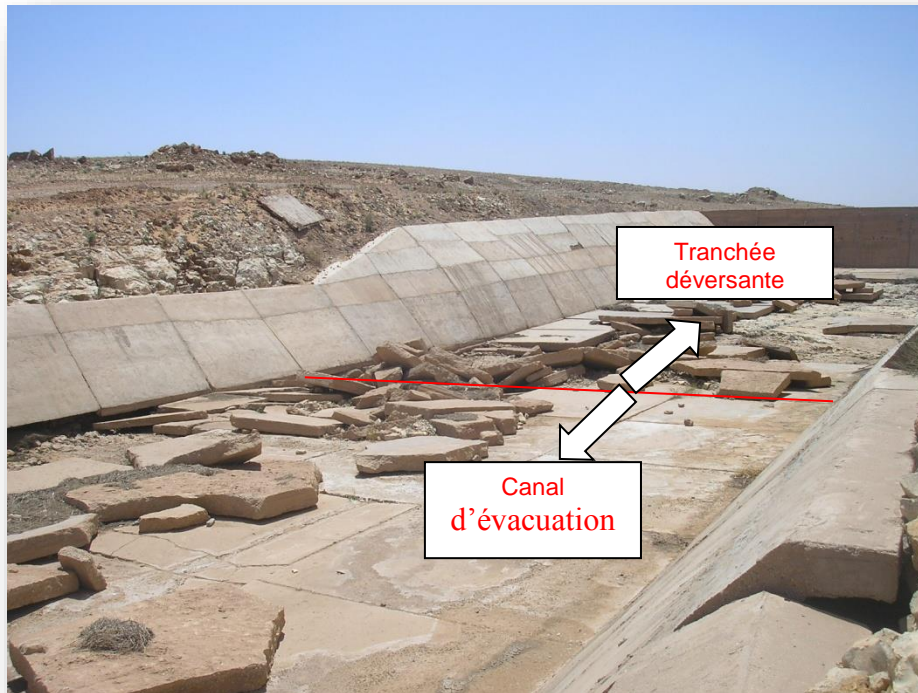
Photo 3.8 : dégradations du radier généralisée sur l'évacuateur des crues (CTH, 2006)
