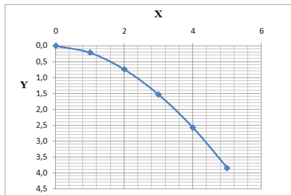
Fig. 3.20 : Profil Creager du déversoir latéral pour l'estimation du volume du béton
