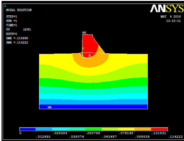
Fig. 3.78 : Champs des déformations Barrage submersible BCR E_{Fondation} = 100.10^3 \text{ KPa}
