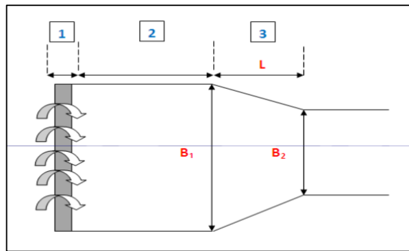
Fig. 3.11 : Configuration spatiale de l'entonnement frontal
