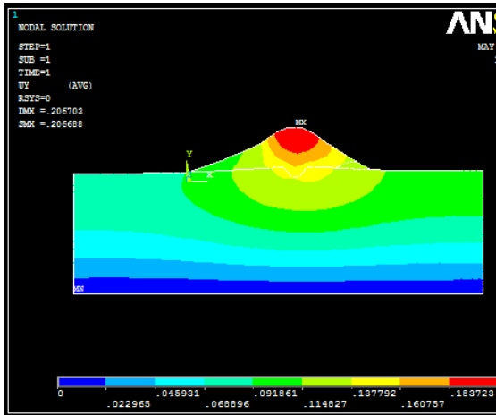
Fig. 3.46 : Champs des déformations Barrage en terre – Remplissage du lac E_{Fondation} = 250.10^3 \text{ KPa}
