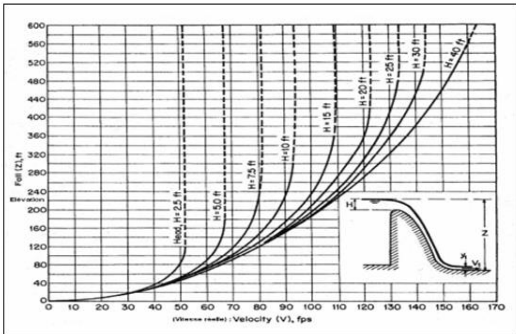
Fig. 2.15 : Variation des vitesses réelles au pied aval d'un déversoir à forte pente aval en fonction de la côte de la retenue et de la charge sur le déversoir
