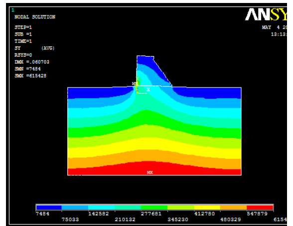
Fig. 3.81 : Champs des contraintes Barrage submersible BCR E_{Fondation} = 200.10^3 \text{ KPa}
