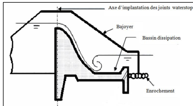
Fig. 2.13: Schéma d'un déversoir poids en béton à profil Creager
