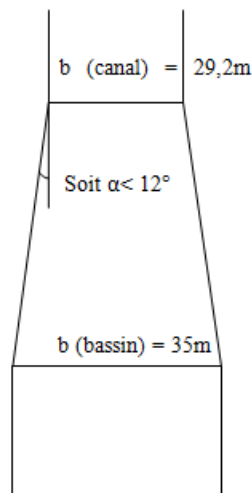
Fig. 3.15 : Configuration planimétrique du bassin de dissipation
