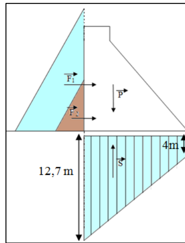
Fig. 3.19 : Force agissants sur le barrage BCR
