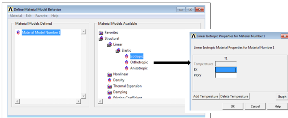
Fig. 3.27 : Choix des propriétés des éléments- code de calcul ANSYS.
