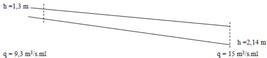
Fig. 3.2 : Profil en long de la tranchée déversante
