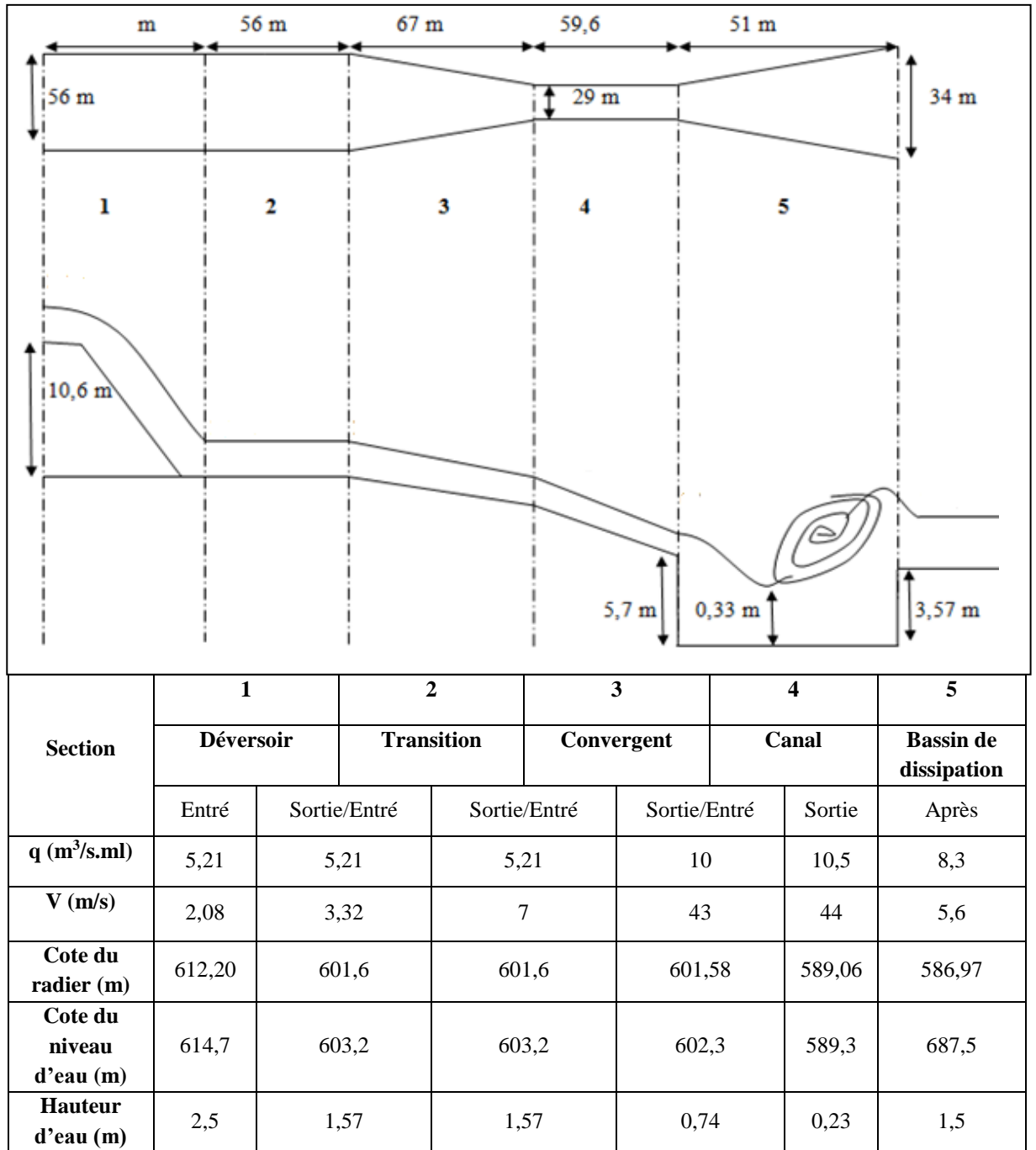
Fig. 3.16 : Paramètres de conception de l'évacuateur à entonnement frontal
