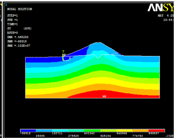
Fig. 3.43 : Champs des déformations Barrage en terre – Remplissage du lac E_{Fondation} = 70.10^3 \text{ KPa}
