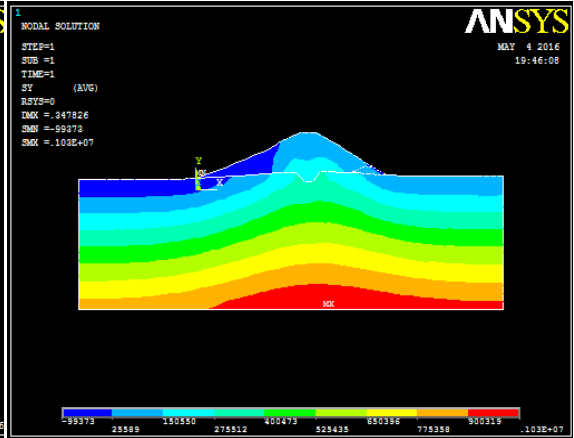
Fig. 3.45 : Champs des déformations Barrage en terre – Remplissage du lac E_{Fondation} = 100.10^3 \text{ KPa}
