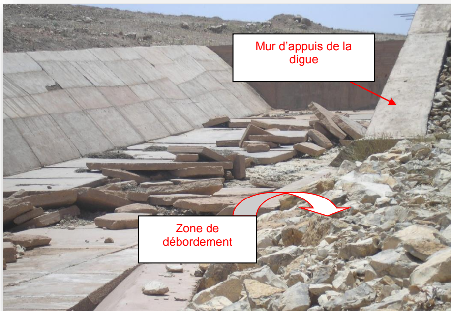
Photo 3.6 : Tranchée déversante : détérioration complète du radier et entraînement des dalles (CTH, 2006)
