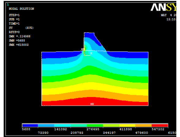
Fig. 3.79 : Champs des contraintes Barrage submersible BCR E_{Fondation} = 100.10^3 \text{ KPa}
