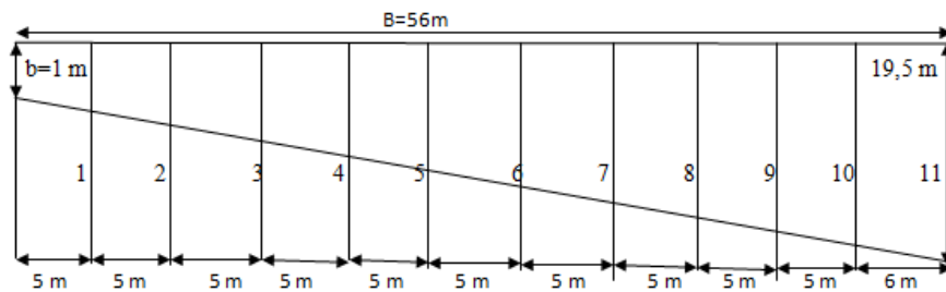
Fig. 3.1 : Vue en plan de la tranchée déversante
