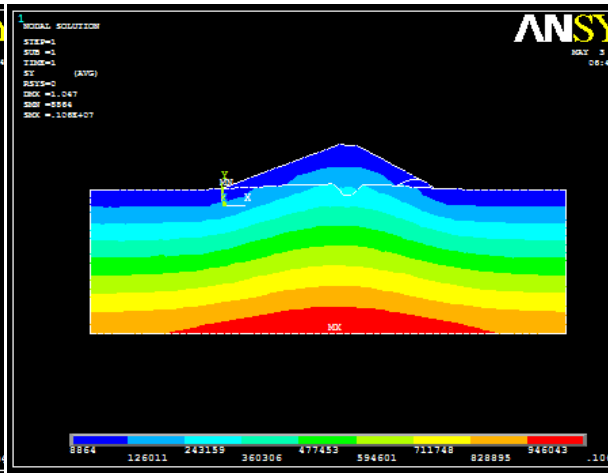
Fig. 3.31 : Champs des contraintes Barrage en terre- E_{Fondation}=30.103 \text{ KPa}
