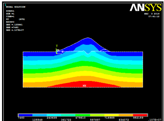
Fig. 3.39 : Champs des contraintes Barrage en terre - E_{\text{Fondation}}=500.10^3 \text{ KPa}
