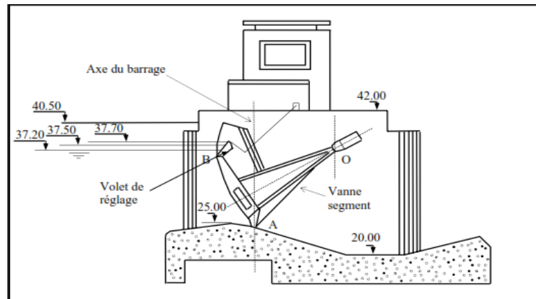
Fig. 2.21: Vanne segment avec clapet déversoir-Barrage Laroussia (M. BOUVARD, 1984)
