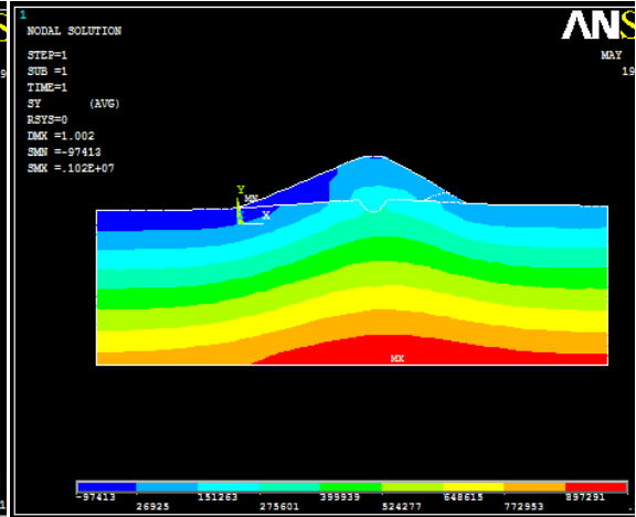
Fig. 3.41 : Champs des déformations Barrage en terre – Remplissage du lac E_{Fondation} = 30.10^3 \text{ KPa}
