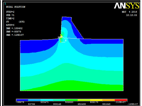
Fig. 3.65 : Champs des contraintes Barrage déversant BCR–Remplissage du lac E_{Fondation} = 70.10^3 \text{ KPa}
