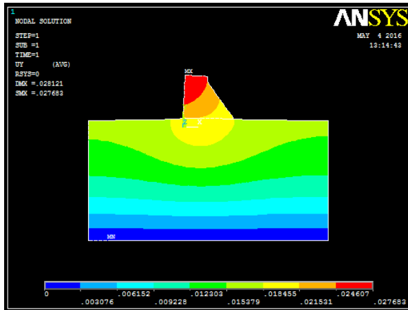
Fig. 3.82 : Champs des déformations Barrage submersible BCR E_{\text{Fondation}} = 500.10^3 \text{ KPa}
