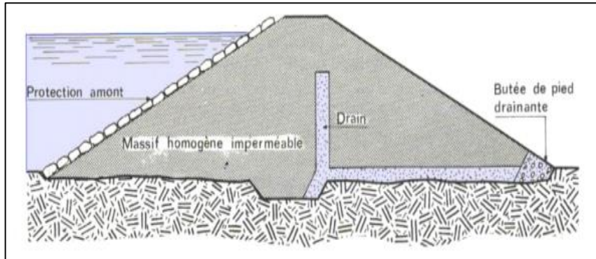
Fig. 2.2 : Profil d'un barrage en terre homogène (L. DJEMILI, 2006)
