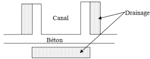
Fig. 3.21 : coupe transversal d'un canal avec drainage
