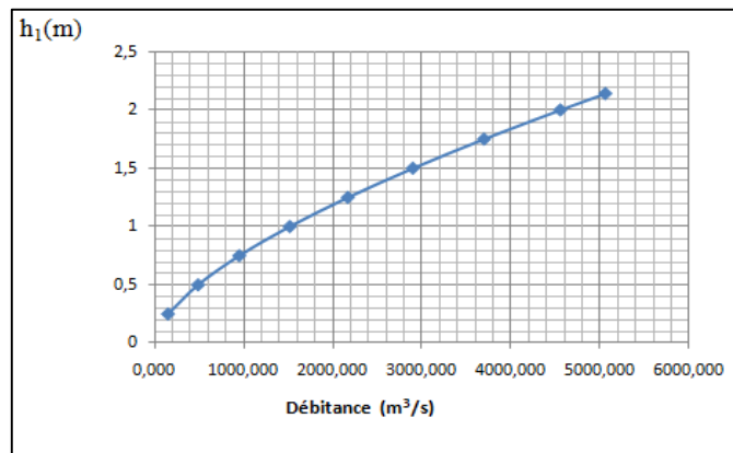
Fig. 3.4 : Courbe de la débitance pour le canal d'évacuation
