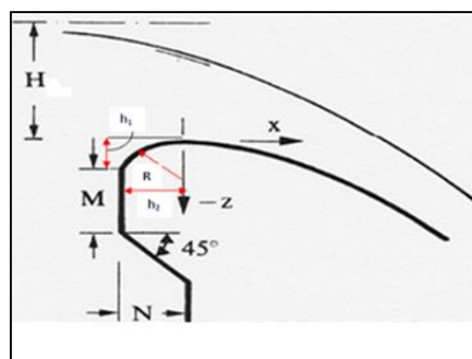
Fig. 2.14 : Dispositions sur les évacuateurs portés par les barrages
