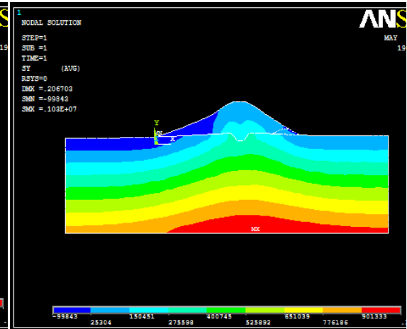
Fig. 3.47 : Champs des déformations Barrage en terre – Remplissage du lac E_{Fondation} = 250.10^3 \text{ KPa}
