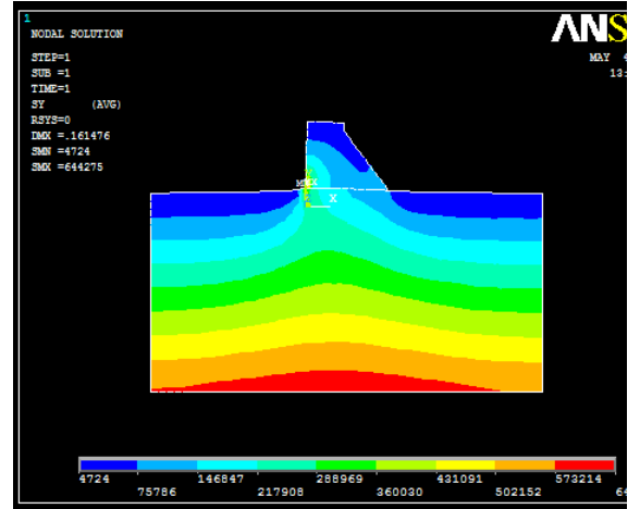
Fig. 3.77 : Champs des contraintes Barrage submersible BCR E_{Fondation} = 70.10^3 \text{ KPa}
