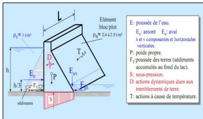
Fig. 2.10 : Actions agissantes sur un barrage poids
