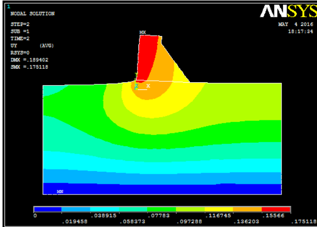
Fig. 3.64 : Champs des déformations Barrage déversant BCR–Remplissage du lac E_{Fondation} = 70.10^3 \text{ KPa}
