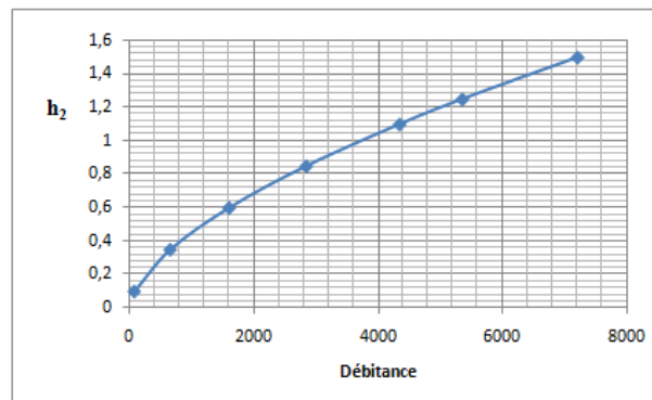
Fig. 3.12 : Courbe de débitance pour la transition
