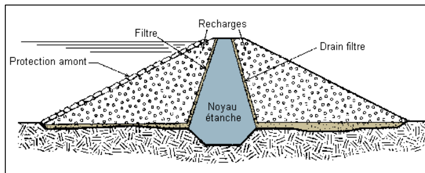
Fig. 2.1 : Profil d'un barrage en enrochement (S6, 01/02/2016)
