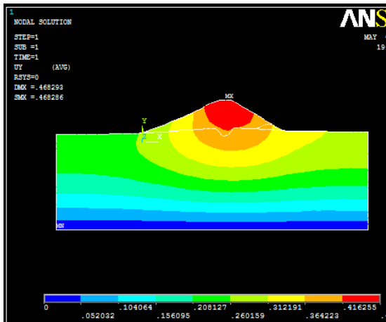
Fig. 3.42 : Champs des déformations Barrage en terre – Remplissage du lac E_{Fondation} = 70.10^3 \text{ KPa}
