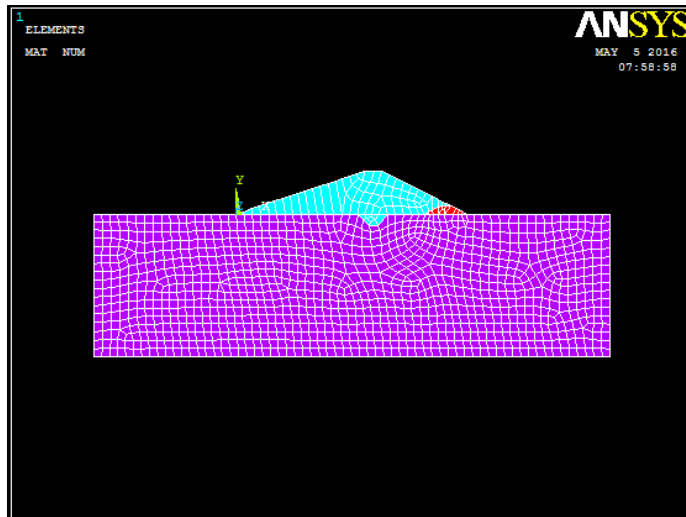
Fig. 3.29 : Discrétisation du barrage
