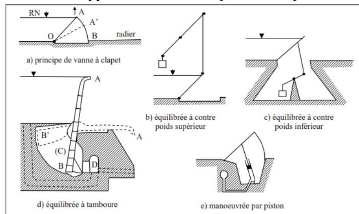
Fig. 2.22: Vanne à clapets (V. MAGLAKELIDZE, 1984)
