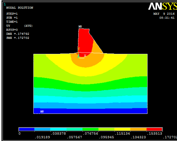
Fig. 3.76 : Champs des déformations Barrage submersible BCR E_{Fondation} = 70.10^3 \text{ KPa}
