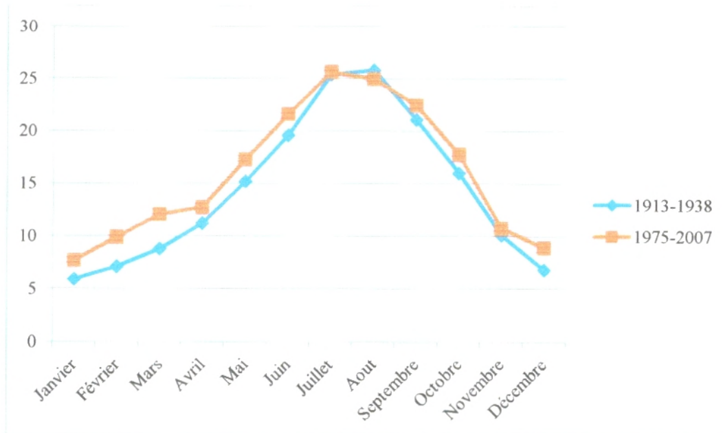
Figure 3. Températures moyennes enregistrées en deux périodes 1913-1938 et 1975-2007
