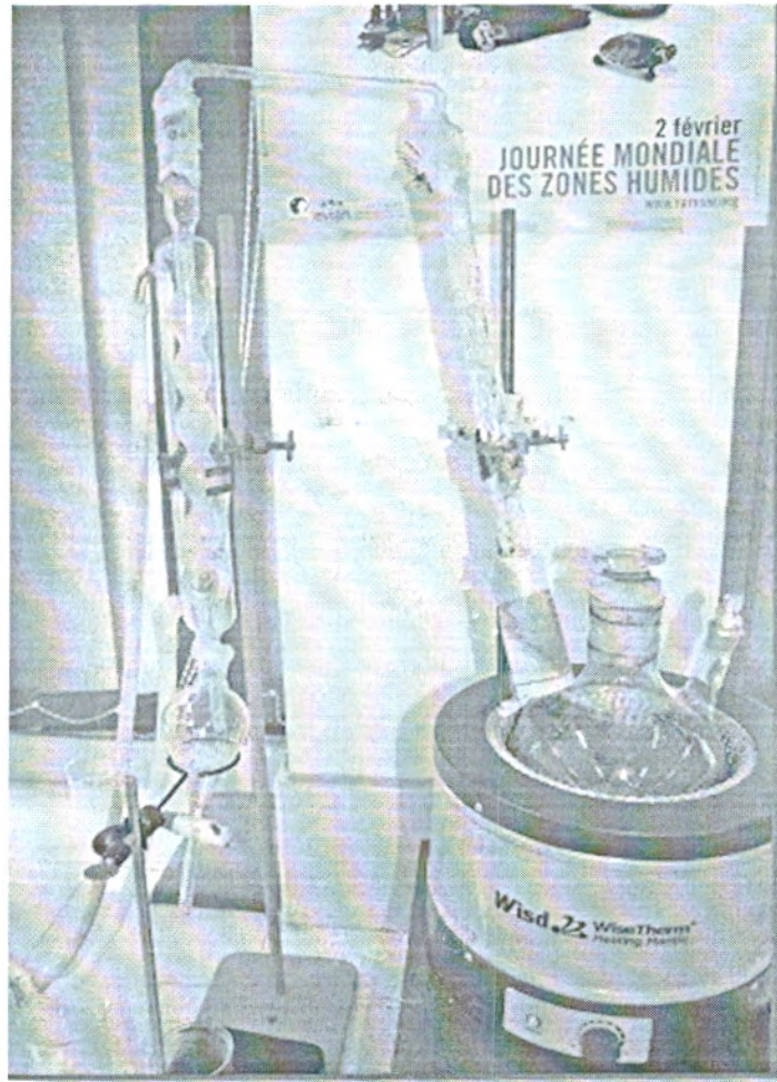
Figure 08 : Montage d'hydrodistillation
