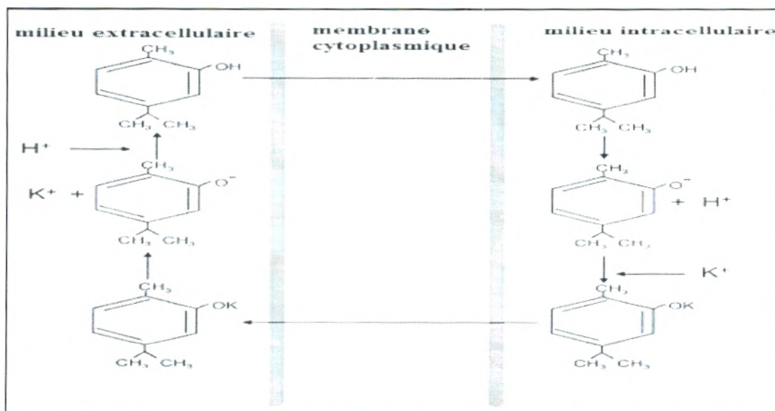
Figure 06 : Mécanisme d'action du carvacrol sur la membrane cellulaire (Ultee et al., 2002).
