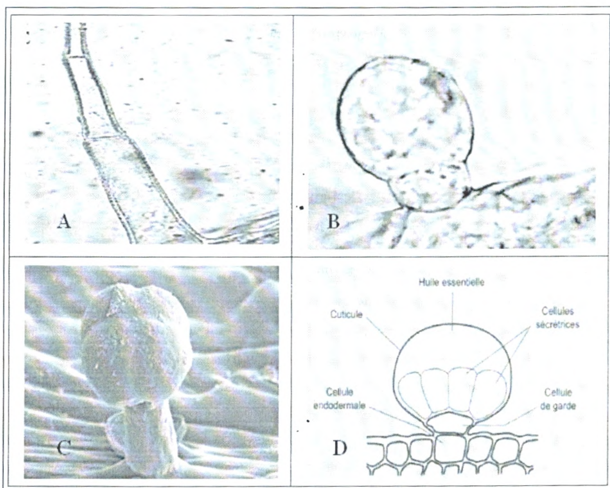
Figure 04: Diversité des structures de sécrétion des huiles essentielles. (A) : poil sécréteur de Mentha pulegium , (B) : trichome glandulaire de Mentha pulegium , (C) : trichome glandulaire de Lippia scaberrima et (D) : structure de trichome glandulaire de Thymus vulgaris (Combrinck et al. , 2007 ; Karray-Bouraoui et al. , 2009).
