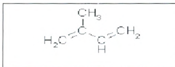
Figure 03: Structure de la molécule d'isoprène (Calsamiglia et al. , 2007).
