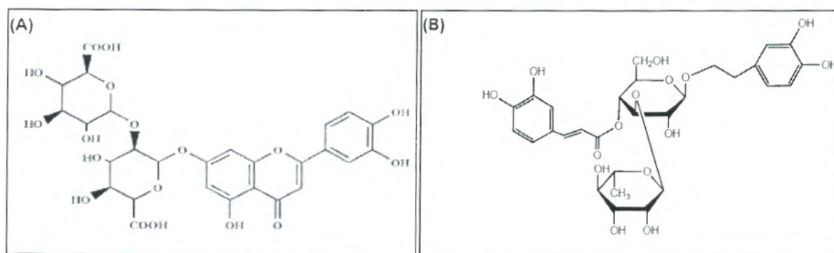
Figure 02 : Structure des principaux polyphénols présents dans l'infusé de verveine odorante.
