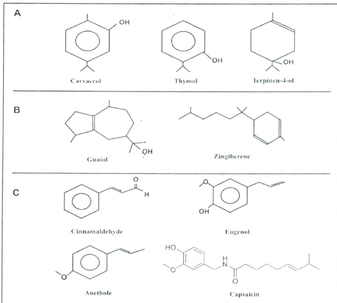
Figure 05 : Structure de quelques composés des huiles essentielles (A) : monoterpénoïdes, (B) : sesquiterpénoïdes et (C) : phénylpropanoïdes (Calsamiglia et al., 2007 ; Khenaka, 2011).
