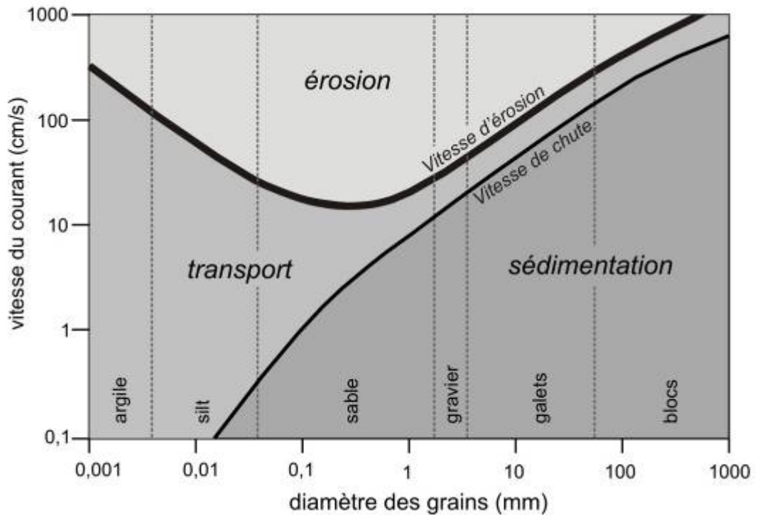
Figure I-1 : Diagramme de Hjulstrom
