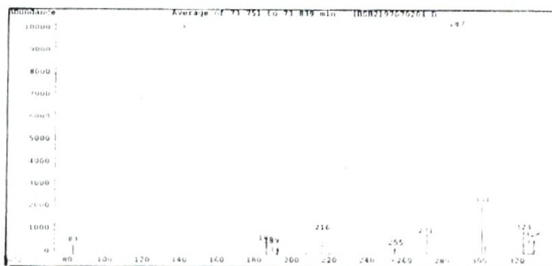
Figure 28. Spectre de masse LC/SM du composé RH7 (ériodictyol)
