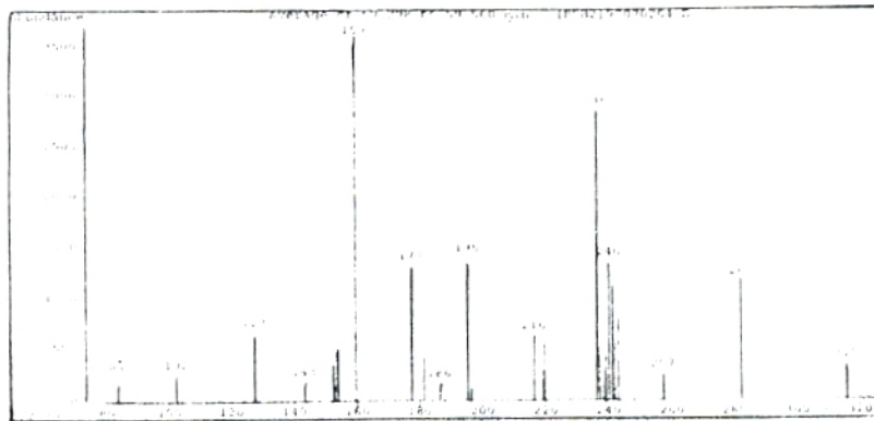
Figure 34. Spectre de masse LC/SM du composé RH3 (acide férulique)
