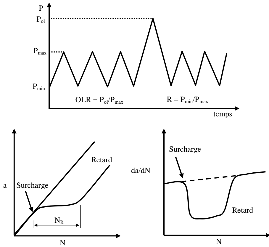
Figure .3 Longueur de la fissure en fonction du nombre de cycle
