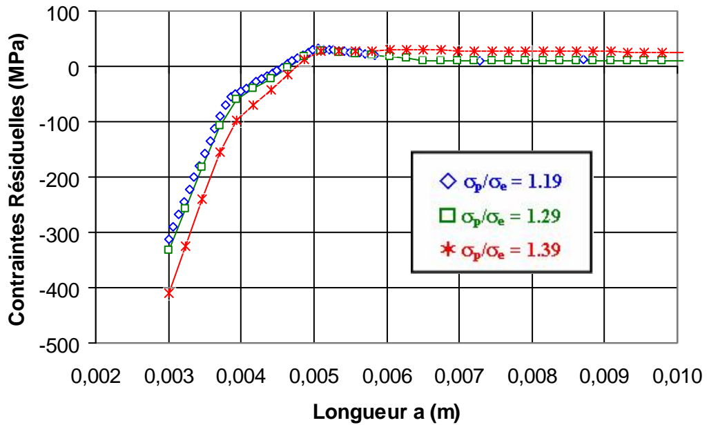
Figure 19. Effect du niveau de préchargement sur la distribution de la contrainte \sigma_{yy} pour l'éprouvette en alliage d'aluminium 6061 T6
