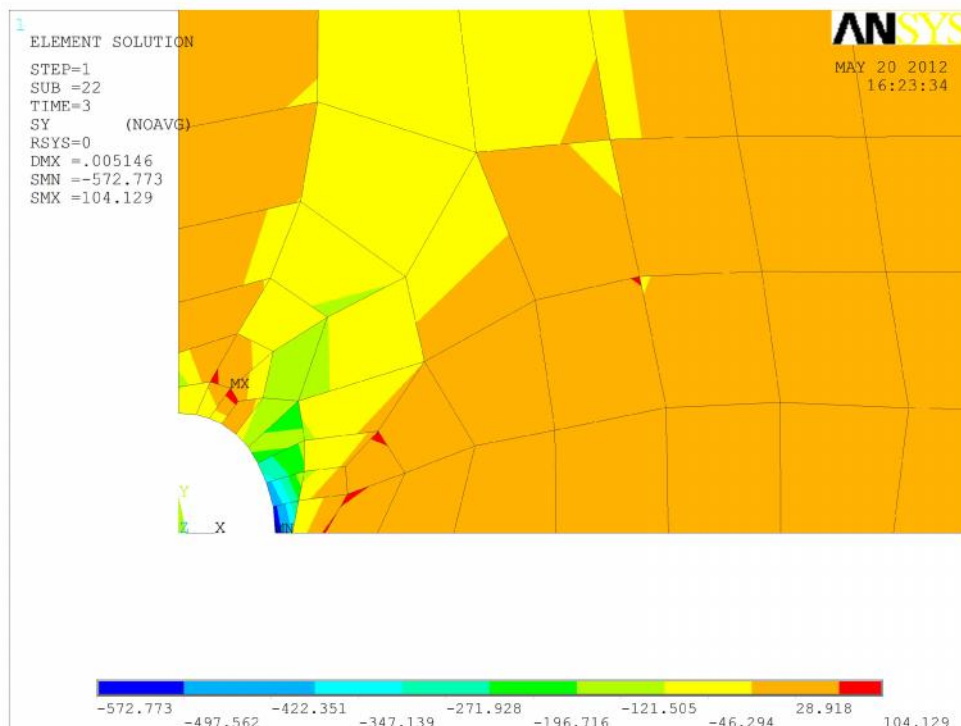
Figure 14 Distribution de la contrainte \sigma_{yy} pour \sigma_p/\sigma_e = 1.350 de l'éprouvette en alliage d'aluminium 2024 T351
