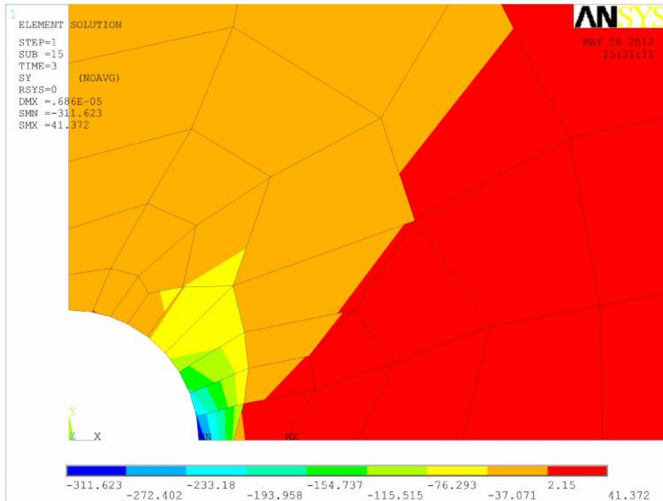
Figure 16. Distribution de la contrainte \sigma_{yy} pour \sigma_p/\sigma_e = 1.19 de l'éprouvette en alliage d'aluminium 6061 T6
