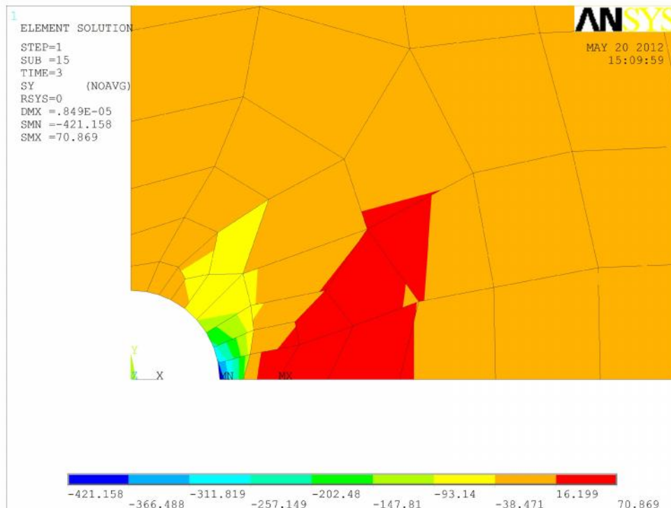
Figure 12. Distribution de la contrainte \sigma_{yy} pour \sigma_p/\sigma_e = 1.102 de l'éprouvette en alliage d'aluminium 2024 T351
