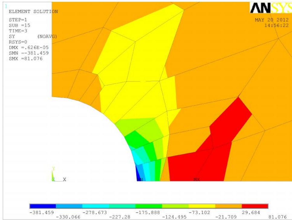
Figure 11 Distribution de la contrainte \sigma_y pour \sigma_p/\sigma_e = 1.047 de l'éprouvette en alliage d'aluminium 2024 T351
