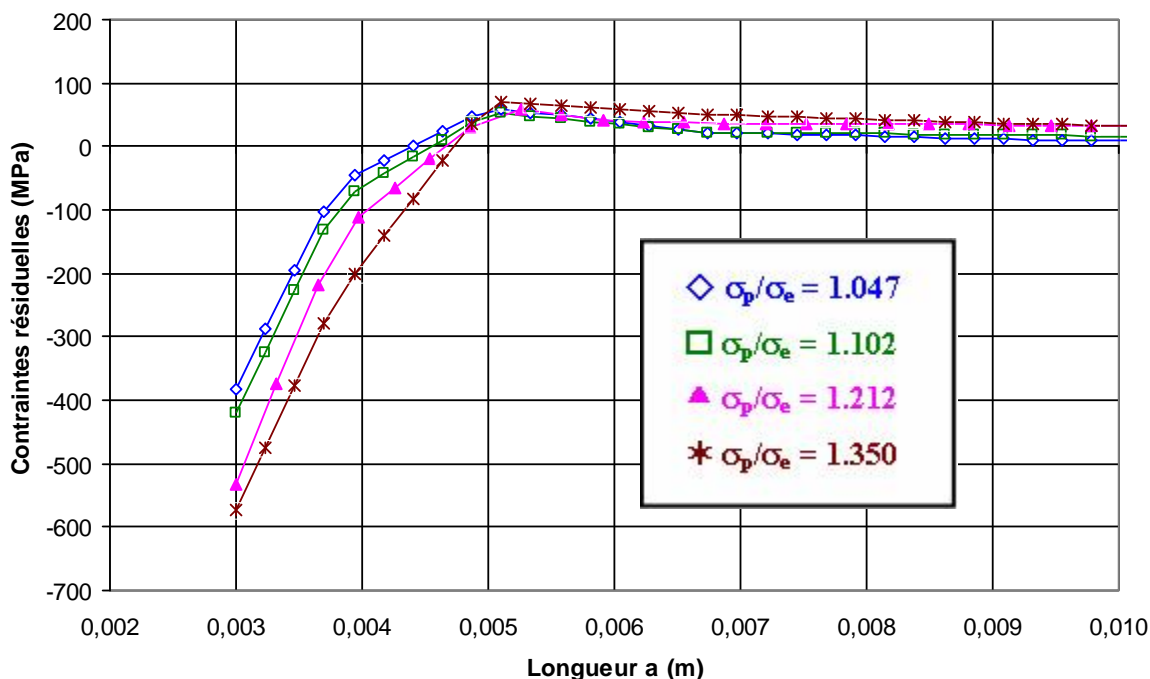
Figure 15. Distribution de la contrainte \sigma_y pour différent niveaux de préchargement suivant l'axe X de l'alliage d'aluminium 2024 T351
