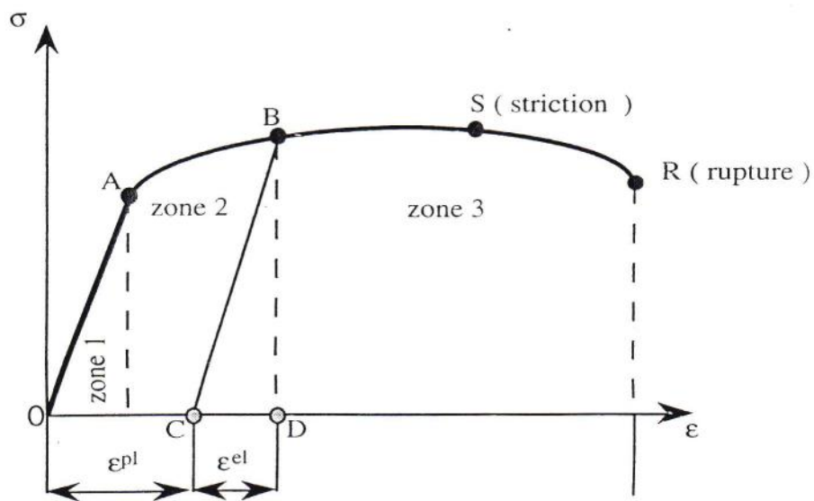
Figure 2. Courbe contrainte - déformation
