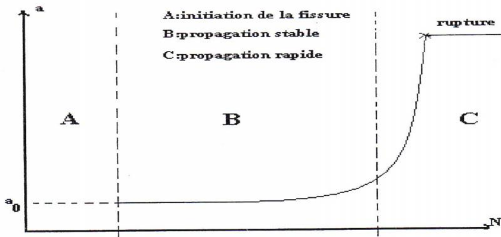
Figure 9. Evolution de la longueur de fissure en fonction du nombre de Cycle
