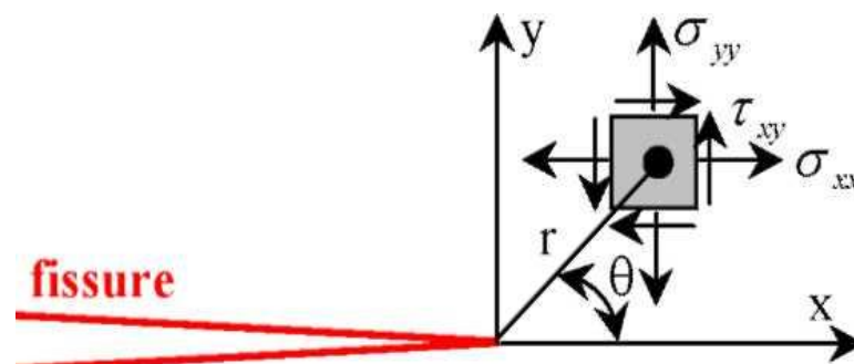
Figure 4. Définition des axes (x, y) et des coordonnées (r, \theta ) au voisinage de l'extrémité d'une fissure
