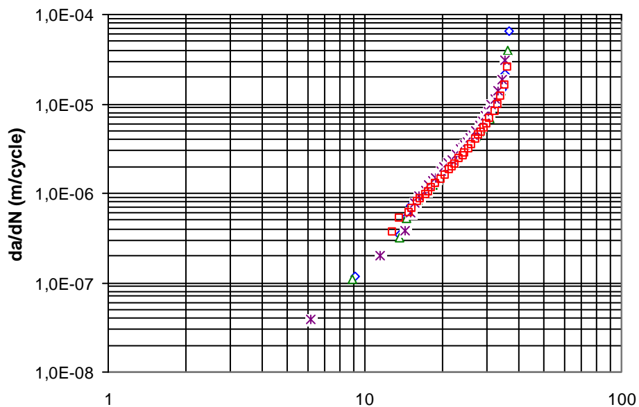
Figure 8. Effet du niveau de prédéformation plastique sur la vitesse de fissuration de l'alliage d'aluminium 6061 T6 à R = 0.25
