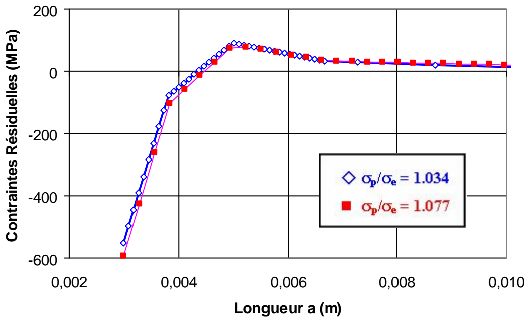
Figure 22. Effect du niveau de préchargement sur la distribution de la contrainte \sigma_{yy} pour l'éprouvette en alliage d'aluminium 7075 T6
