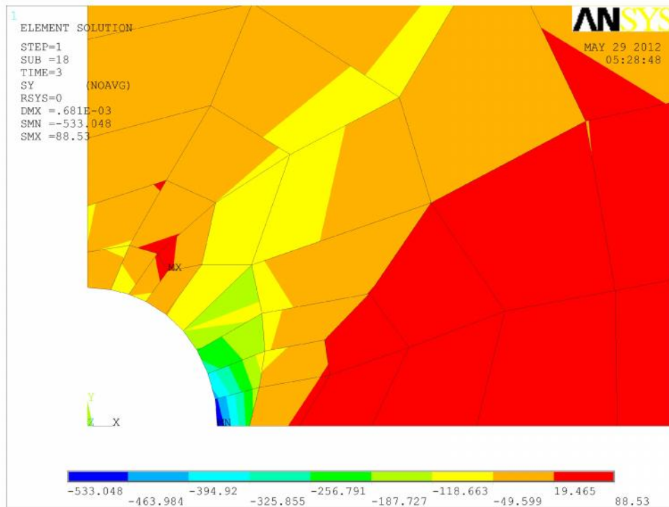
Figure 13 Distribution de la contrainte \sigma_{yy} pour \sigma_p/\sigma_e = 1.212 de l'éprouvette en alliage d'aluminium 2024 T351
