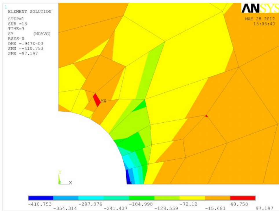
Figure 18. Distribution de la contrainte \sigma_{yy} pour \sigma_p/\sigma_e = 1.39 de l'éprouvette en alliage d'aluminium 6061 T6
