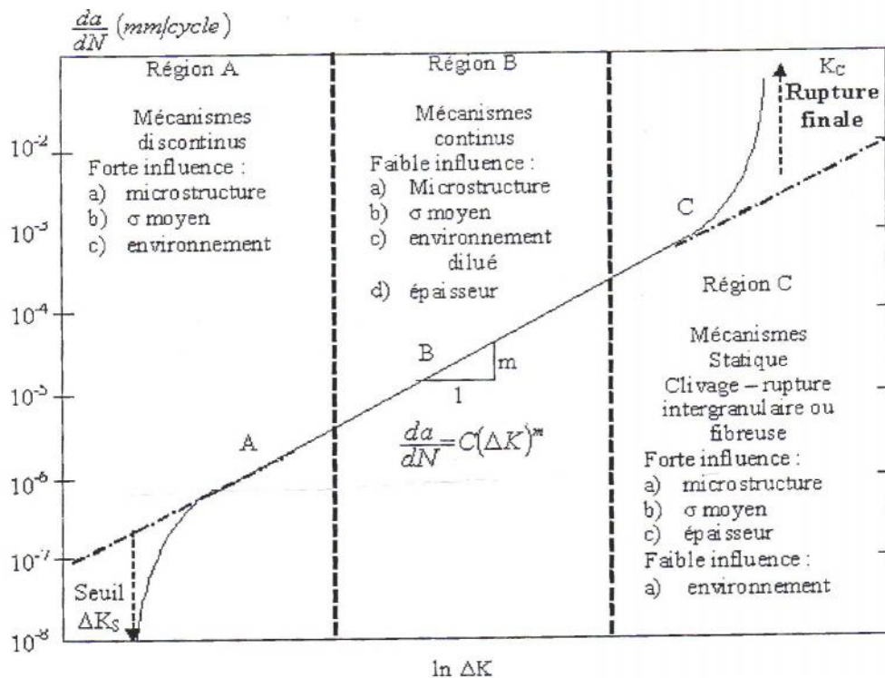
Figure 10. Représentation schématique des différents régimes de propagation
