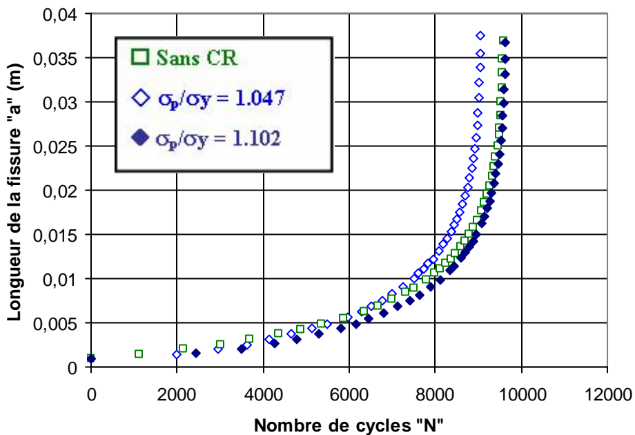
Figure 3. Comparaison de la durée de vie en fatigue en absence et en présence des contraintes résiduelles pour l'alliage d'aluminium 2024 T351 à R = 0.25
