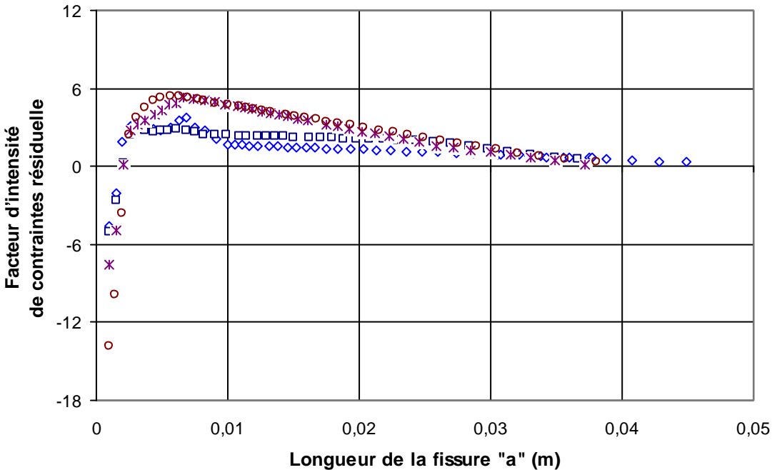
Figure 5. Variation du facteur d'intensité de contraintes résiduelles Kr pour différents niveaux de prédéformation de l'alliage d'aluminium 2024 T351
