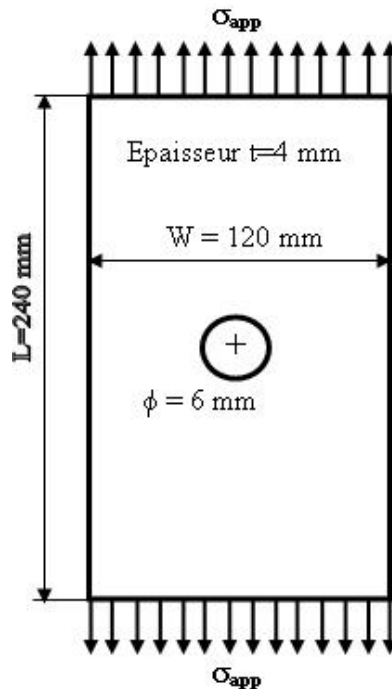
Figure 1. Géométrie de la plaque
