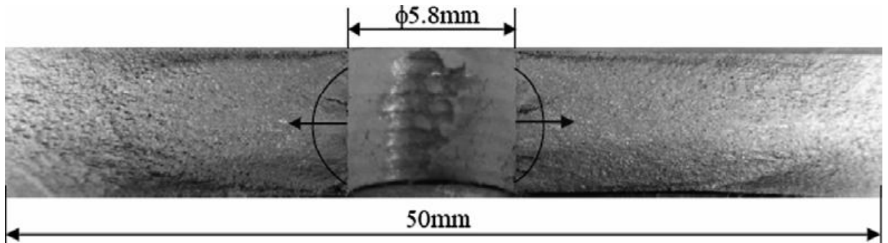
Figure 1. Exemple de fissure sur une plaque trouée [2]
