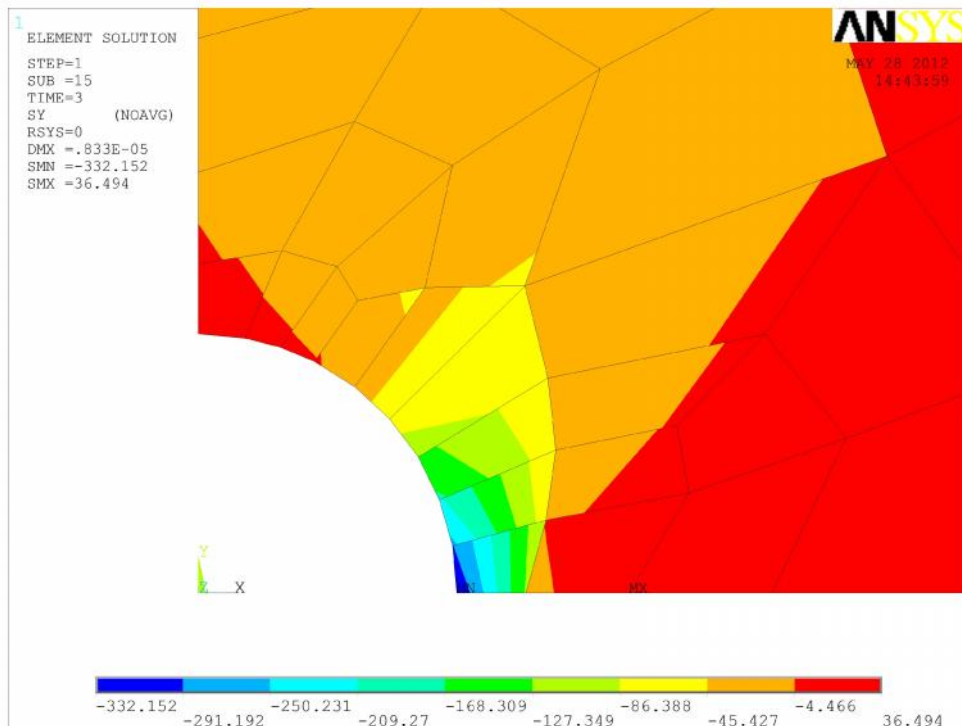
Figure 17. Distribution de la contrainte \sigma_{yy} pour \sigma_p/\sigma_e = 1.23 de l'éprouvette en alliage d'aluminium 6061 T6
