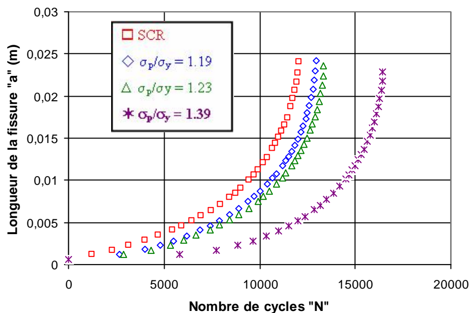
Figure 7. Comparaison de la durée de vie en fatigue en absence et en présence des contraintes résiduelles pour l'alliage d'aluminium 6061 T6 à R = 0.25
