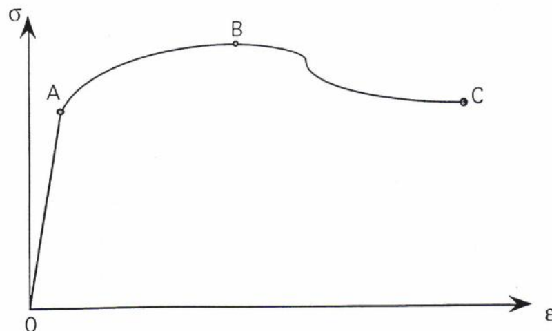
Figure 4 : Phénomène d'écrouissage et d'adoucissement en traction simple
