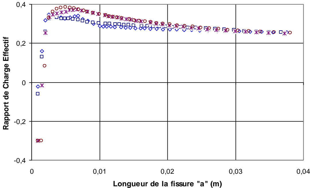
Figure 6. Variation du rapport de charge effectif pour différents niveaux de prédéformation de l'alliage d'aluminium 2024 T351
