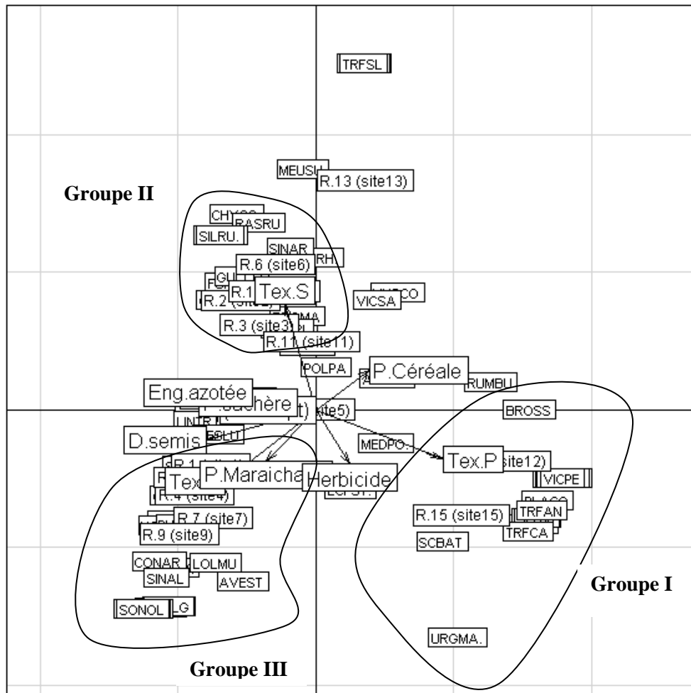
Fig.4.18 : Projection des espèces végétale et des facteurs sur le plan factoriel.
