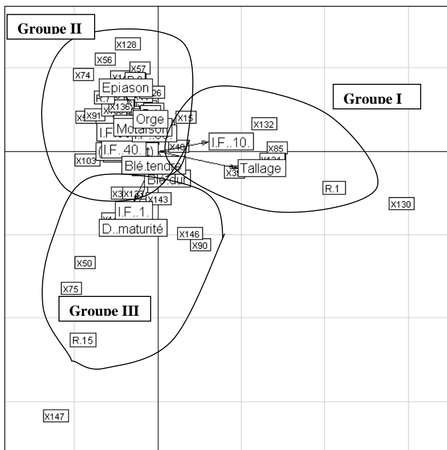
Fig. 4.21 : Projection des espèces entomologique et des facteurs sur le plan factoriel
