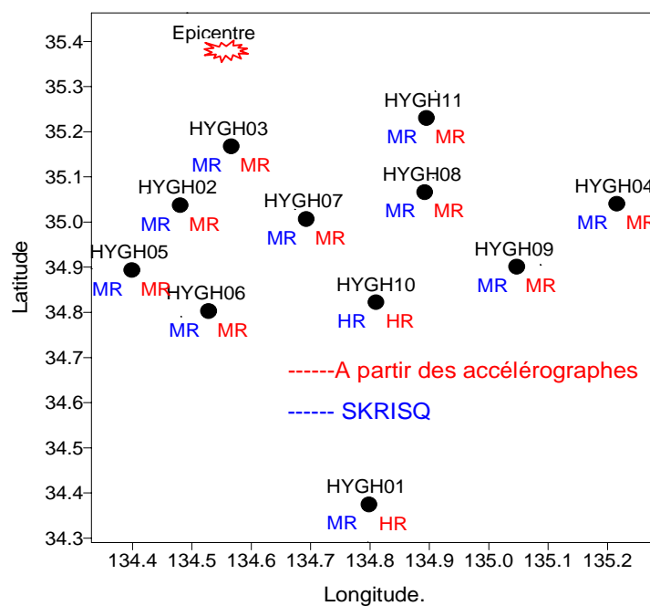
Figure.VI. 4. Niveaux de risques obtenus par SKRISQ, et calculés à partir des enregistrements réels
