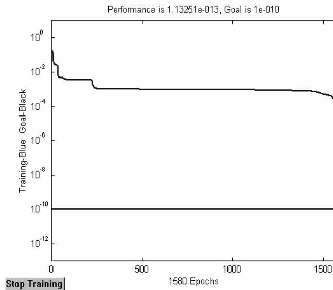
Figure.V. 14.Processus d'apprentissage
