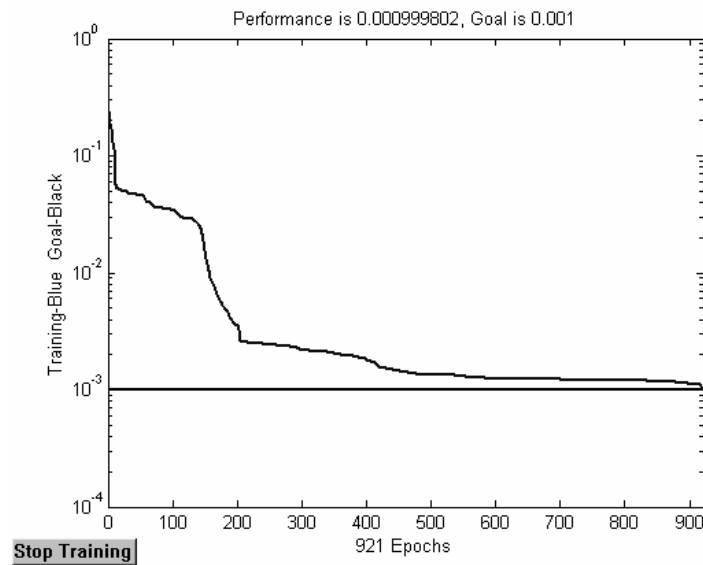
Figure.V.22..Processus d'apprentissage
