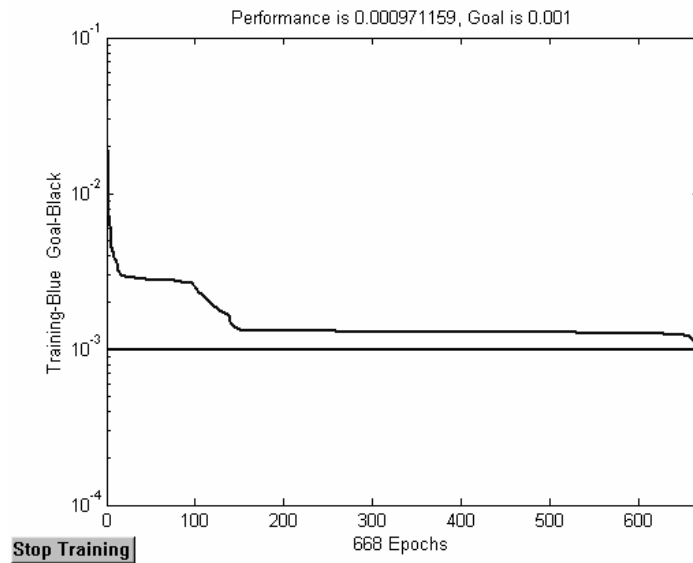
Figure.V. 19.Processus d'apprentissage
