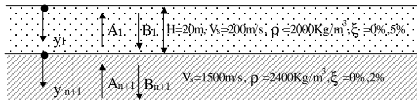
Figure.III. 3. Profil du sol monocouche
