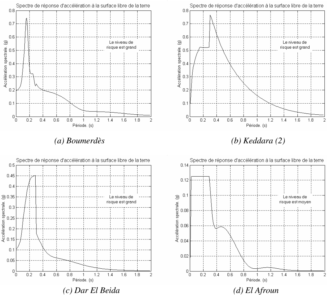
Figure.VI. 20.Spectres de réponse d'accélération estimés par SKRISQ
