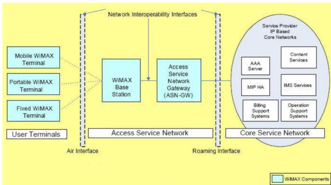
Figure I.3 : Architecture du réseau Wimax [4].
