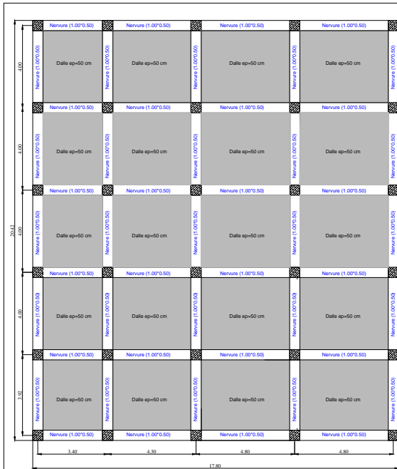
Plan de coffrage et ferrailage du radier général ECHELLE : 1/100
