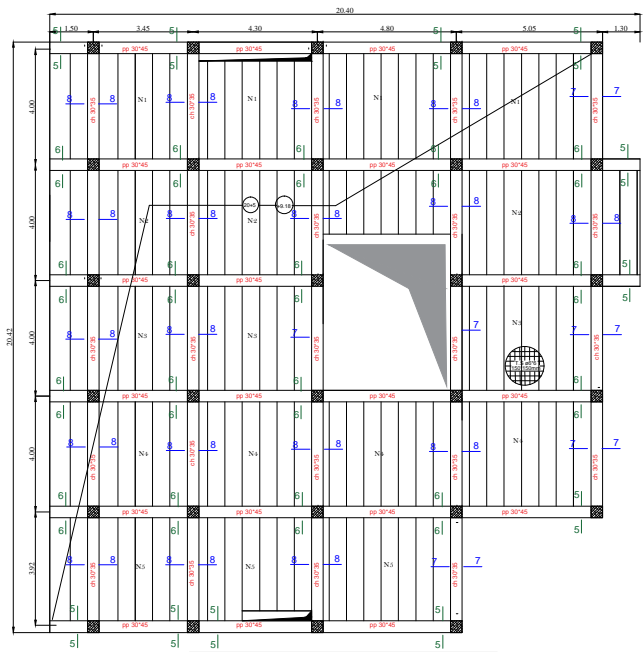
Plan coffrage Etage courant & Terrasse. Echelle : 1/100
