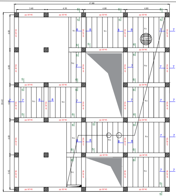
Plan coffrage MEZZANINE Echelle : 1/100
