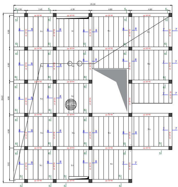
Plan coffrage 1er ETAGE Echelle : 1/100
