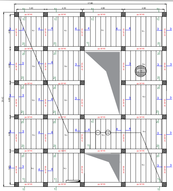
Plan coffrage Sous Sol 1 & RDC Echelle : 1/100
