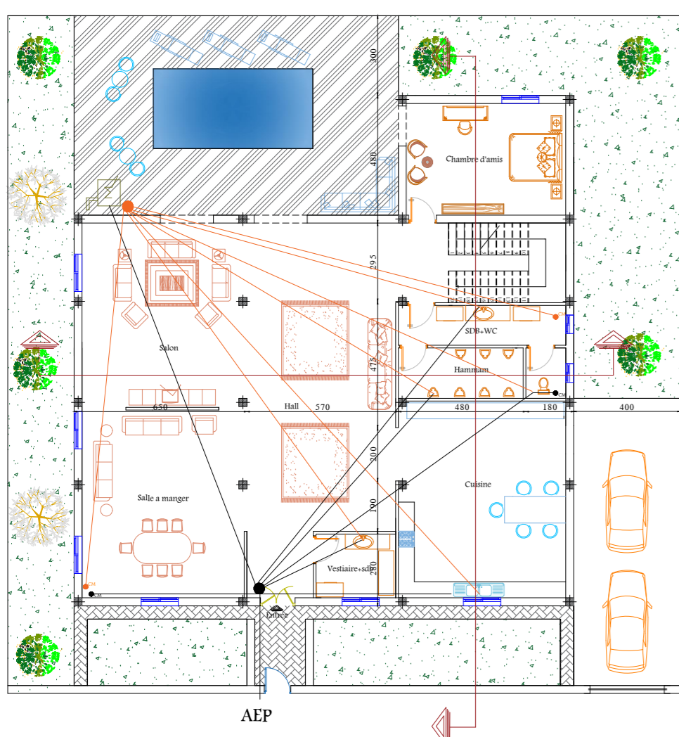
Plan CES plomberie ( rdc 1+ er étage )
