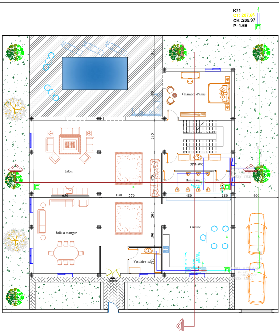
Plan d'assainissement + PVC ( rdc 1+ er
