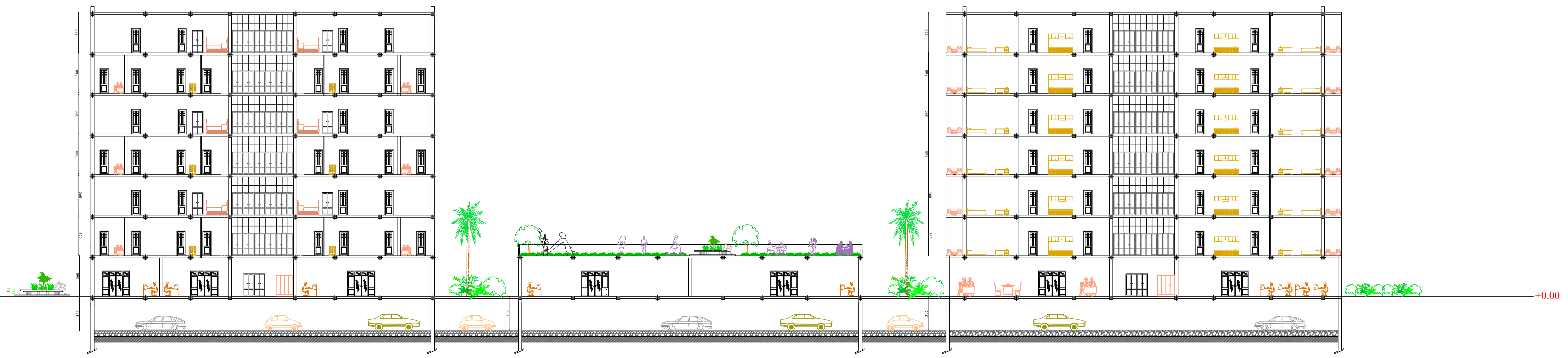
Coupe transversale A-A 1/200
