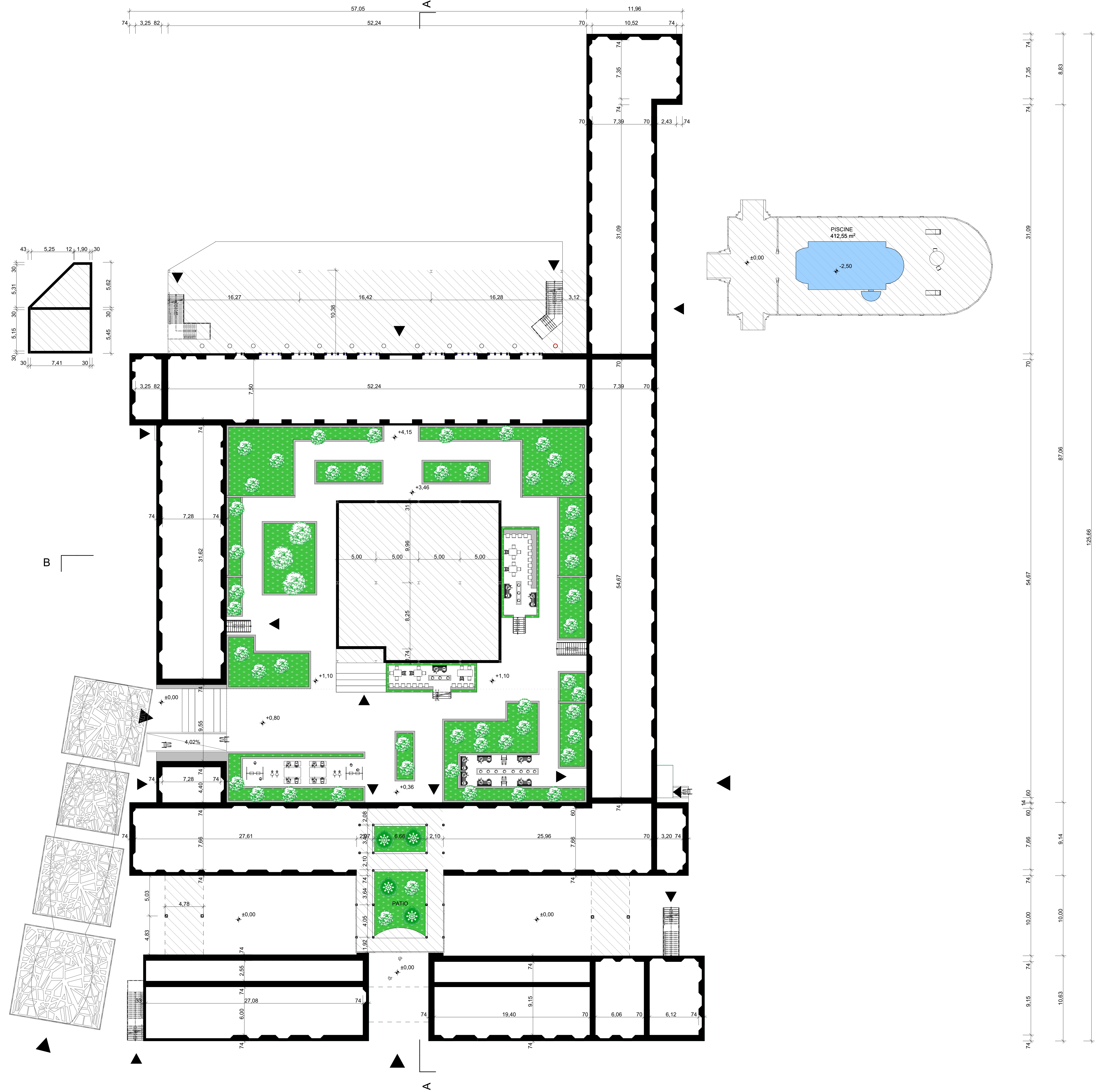
PLAN DE STRUCTURE NIVEAU 0 (1/200)
