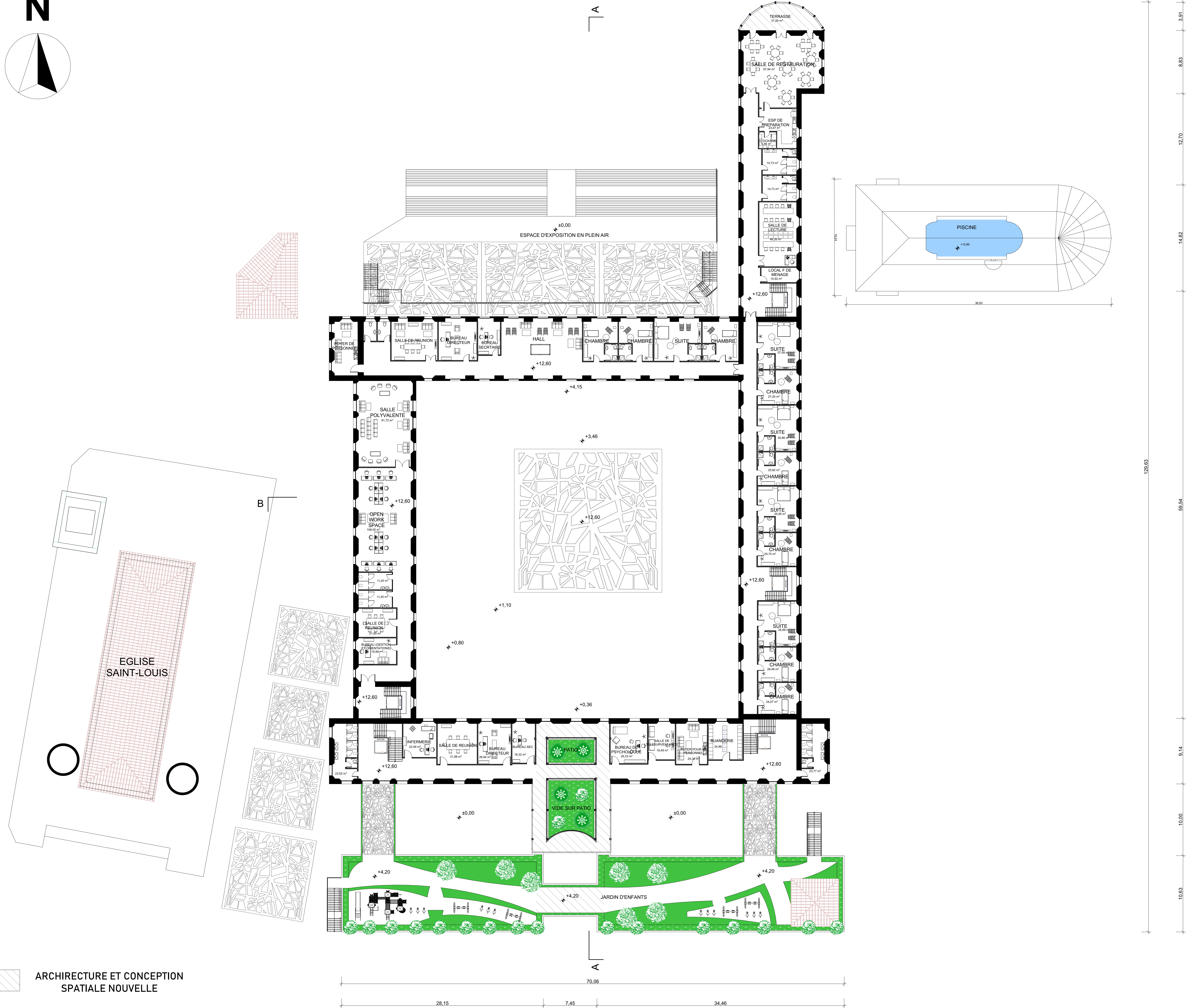
PLAN DE 3EME NIVEAU 1/200
