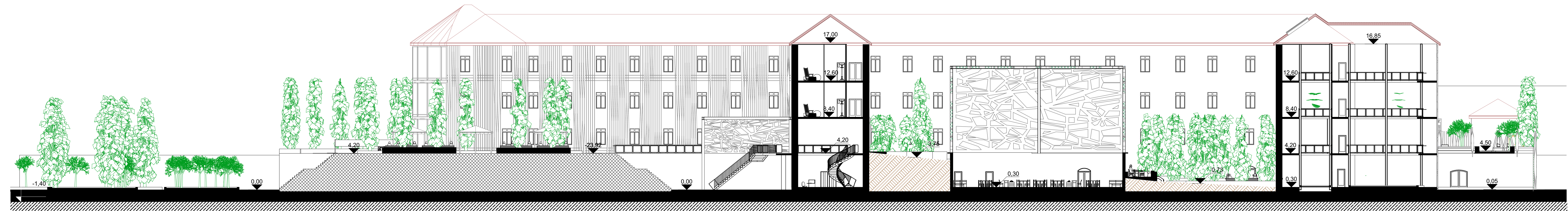
COUPE AA 1/200
