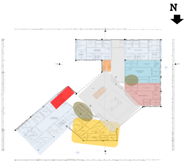
PLAN 1 er ETAGE
