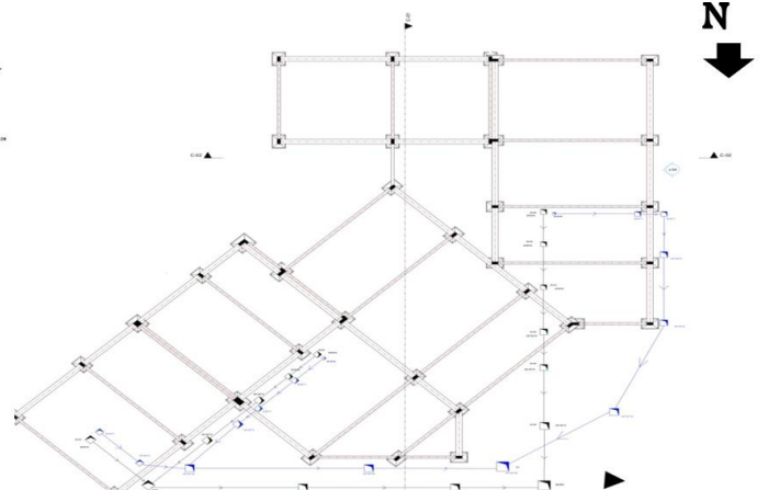
PLAN FONDATION
