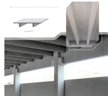
Figure 94: dalle nervurée préfabriquée
