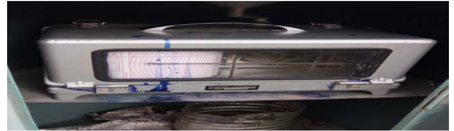
Photos 07 : le pluviographe
