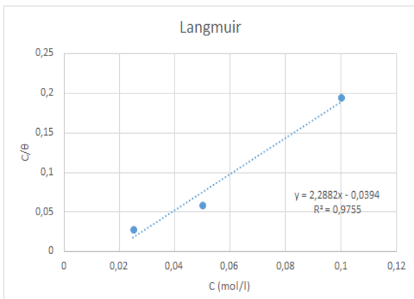
Figure 3.4: Courbe de l'adsorption de l'inhibiteur (AA) selon modèle de Langmuir
