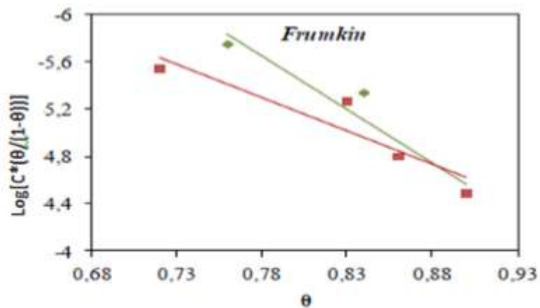
Figure 2.5 : Courbe de l'adsorption de l'inhibiteur selon le modèle de Frumkin (Faustin, 2013)
