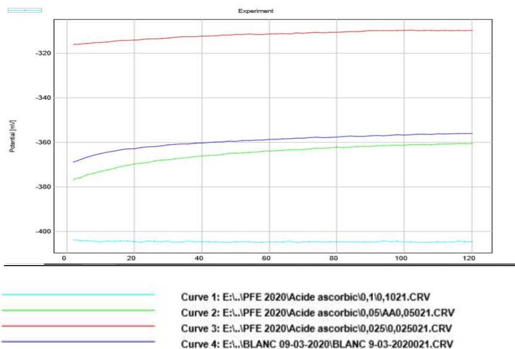
Figure 3.1: Diagrammes PCO de l'acier immergé dans le milieu d'étude en absence et en présence de différentes concentrations de l'acide ascorbique.
