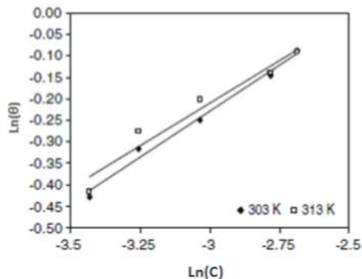
Figure 2.3 : La courbe de l'adsorption de l'inhibiteur selon l'isotherme de Freundlich (Badiea, et al., 2008)
