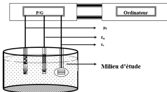
Figure 2.1: Montage électrochimique (Dob, 2018)
