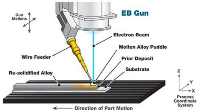
Figure 1.8 : Le processus d'impression 3D par fusion directe de matière [10]
