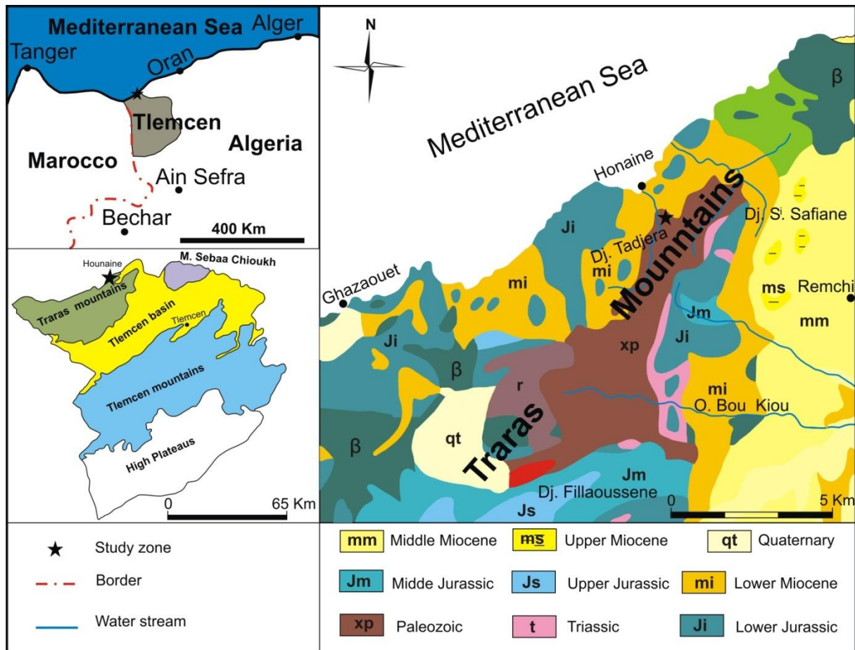
Fig. 2. - Localisation des Monts de Traras.
