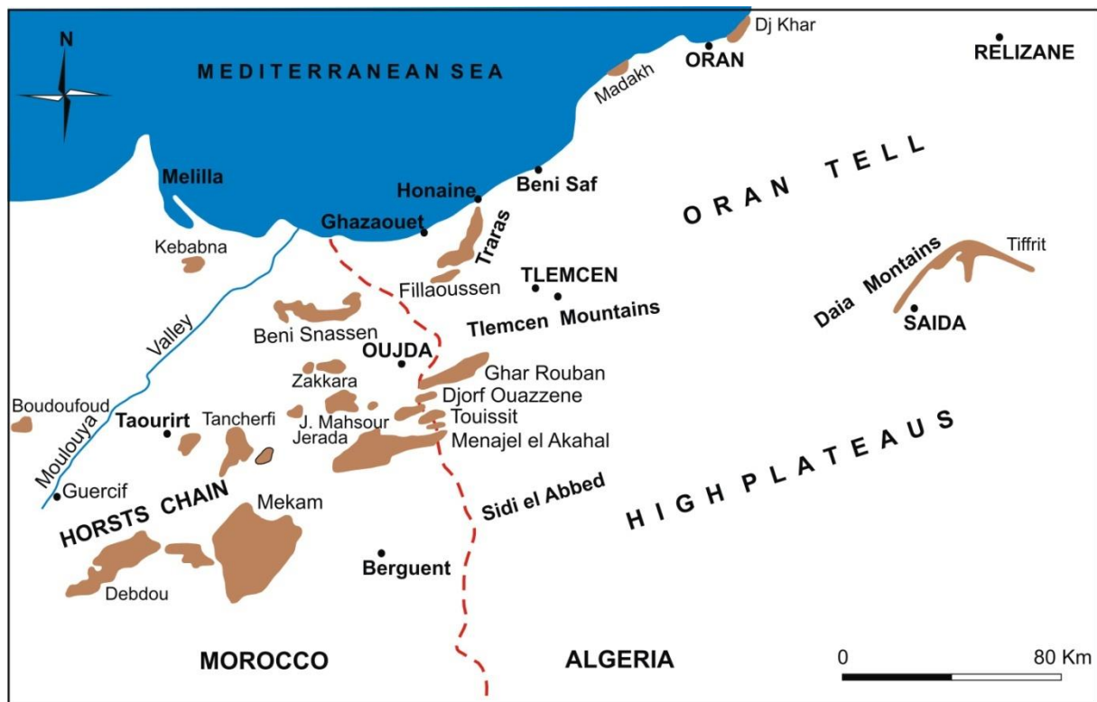
Fig. 1. - Carte de la situation des principaux massifs paléozoïques de part et d'autre de la frontière algéro-marocaine (d'après Ciszak 1993)
