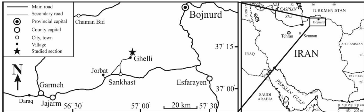
Fig. 3. Situation géographique de la région de Ghelli
