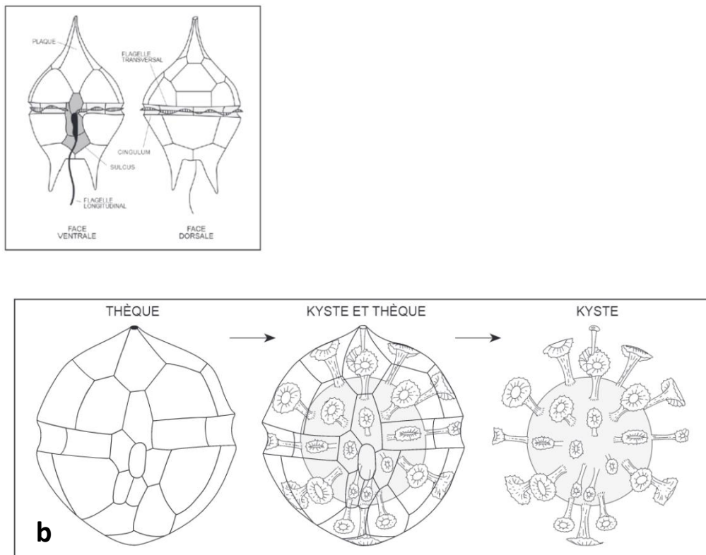
Fig. 1 : a. principaux caractères morphologiques du stade mobile d'un dinoflagellé moderne typique. b. relation entre thèque et kyste d'un même dinoflagellé (Fensome et al. 1998)
