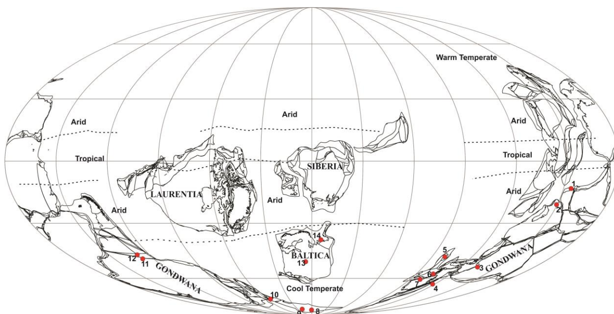
Fig. 6. Répartition paléogéographique de Saharidia fragilis durant le Furongien.
