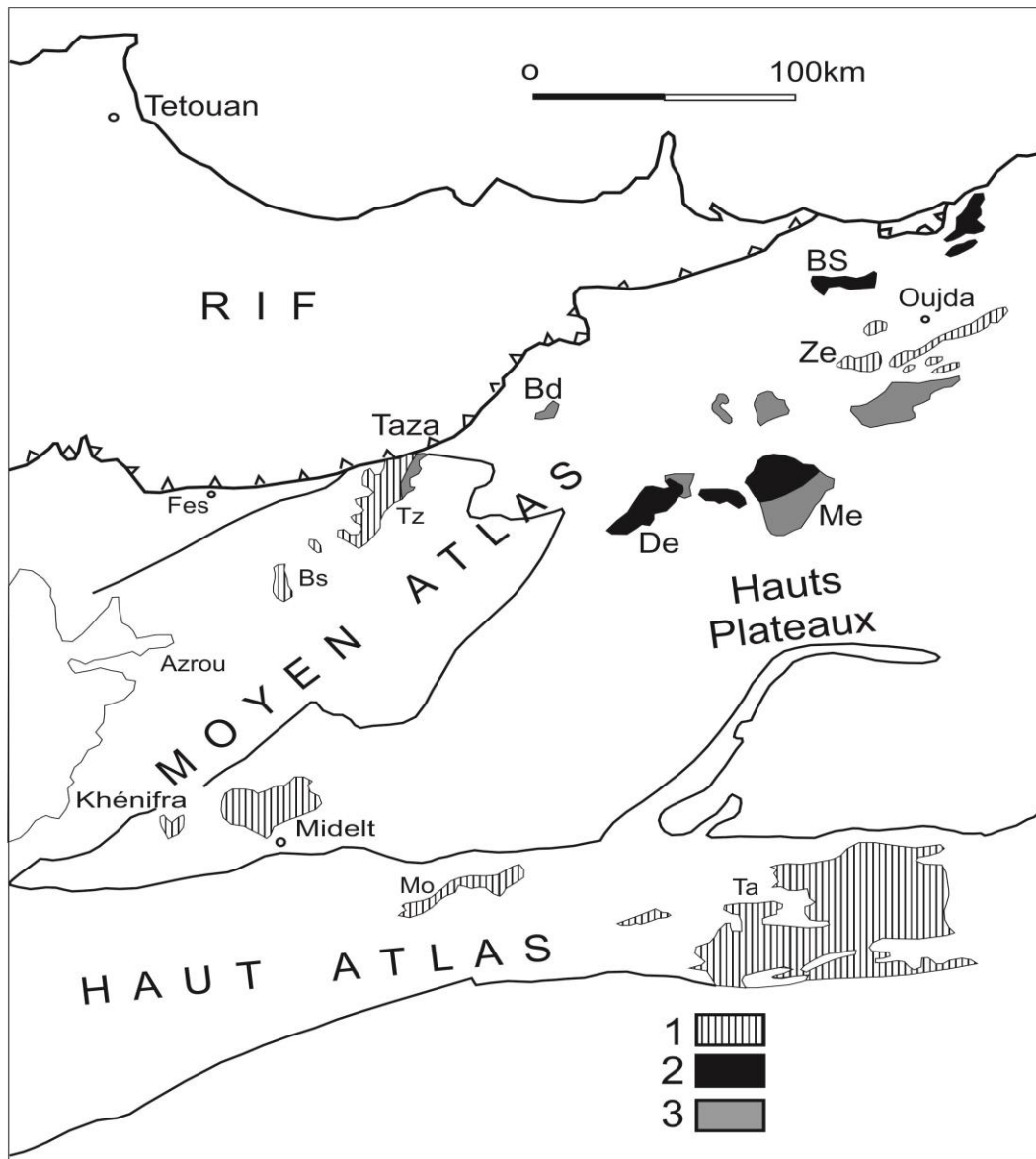
Fig. 1- Localisation des boutonnières paléozoïques au Maroc (Rauscher et al. 1982). 1. Paléozoïque inférieur ; 2. Carbonifère Inférieur ; 3. Viséen supérieur à Westphalien ; Bs. Bsabis; Tz. Tazekka ; Bd. Boudoufoud ; De. Debbou; Me. Mekam ; BS. Beni Snassène ; Mo. Mougueur; Ta. Tamelelt
