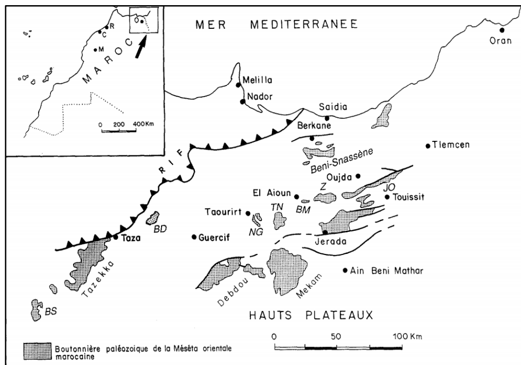
Fig. 4- Les affleurements paléozoïques de la région d'étude (Berkhli et al. 1993)
