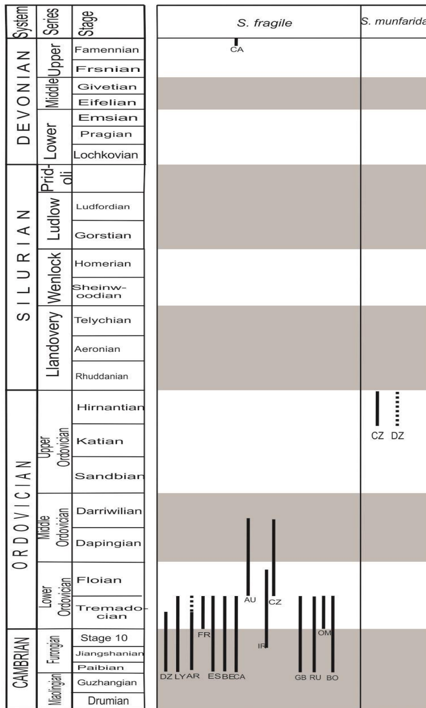
Fig. 5. Répartition stratigraphique des différentes espèces de Saharidia
