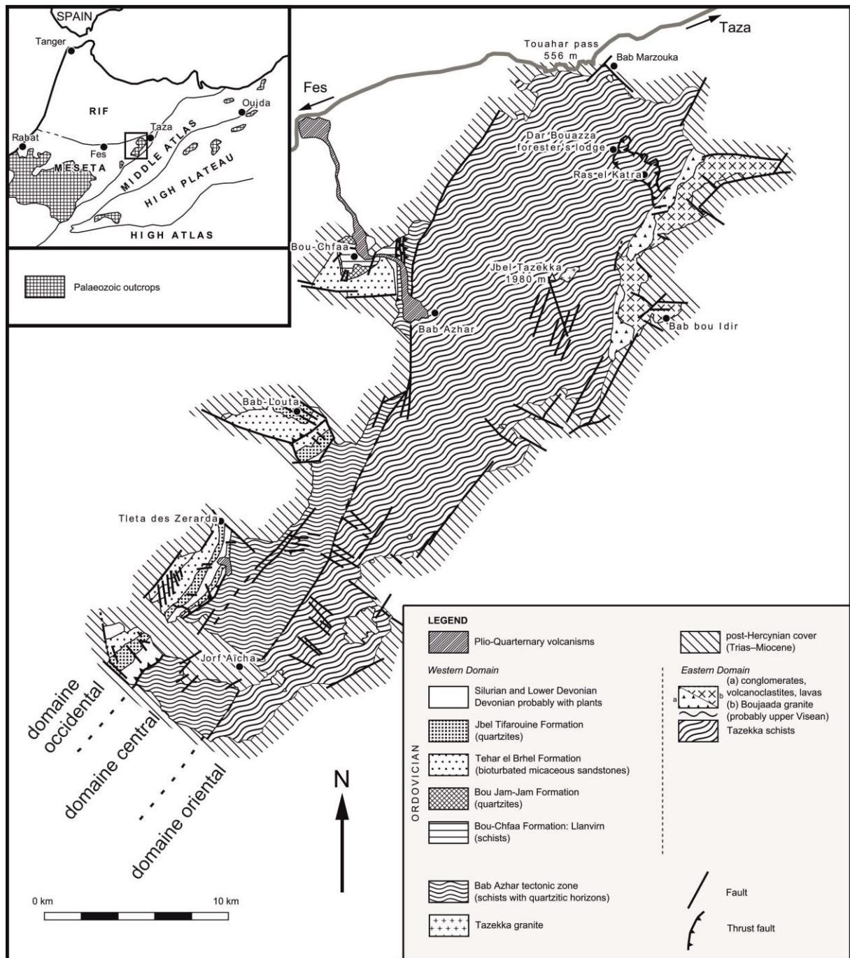
Fig. 3- Carte géologique du massif de Tazekka (Hoepffner 1987)
