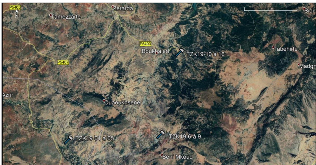
Fig. 5- Positions des coupes et échantillons analysés
