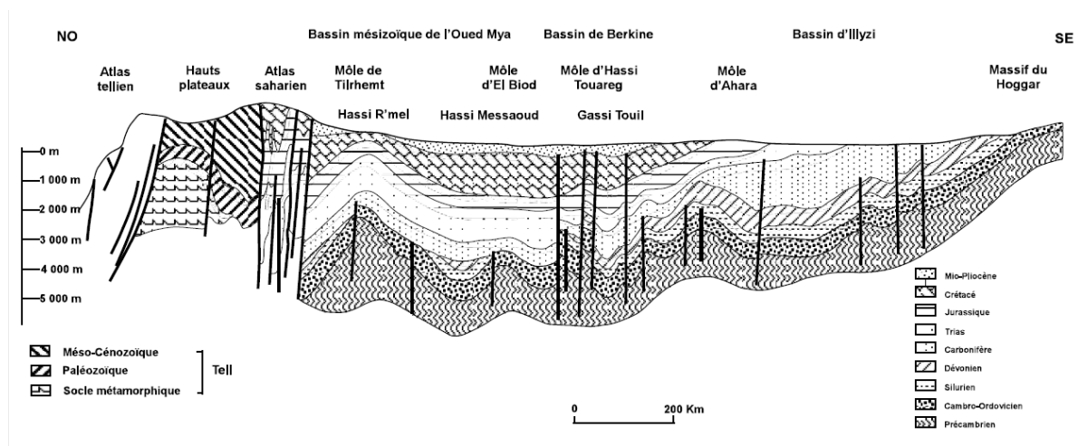
Fig. 1. Corrélation entre les différents bassins du Sahara ; position du matériel étudié (Hassi R'mel) par rapport au matériel type (Hassi Messaoud) (Peterson 1985)
