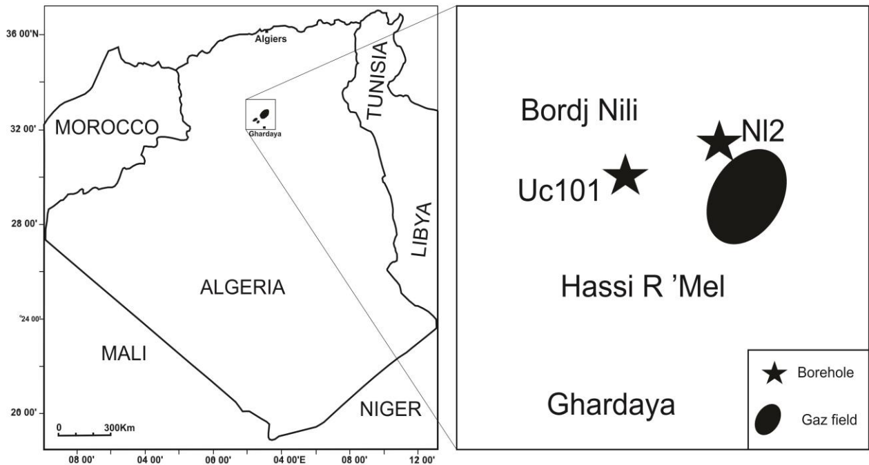
Fig. 2. Localisation des sondages NL2 et UC101
