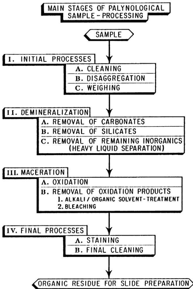
Fig. 3 Etapes de traitement palynologique d'une roche sédimentaire Ediger (1986)
