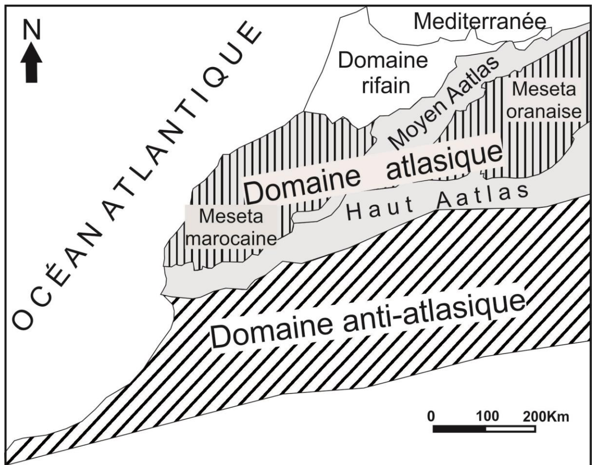
Fig. 2- Les domaines structuraux du Maroc (Michard 1976)
