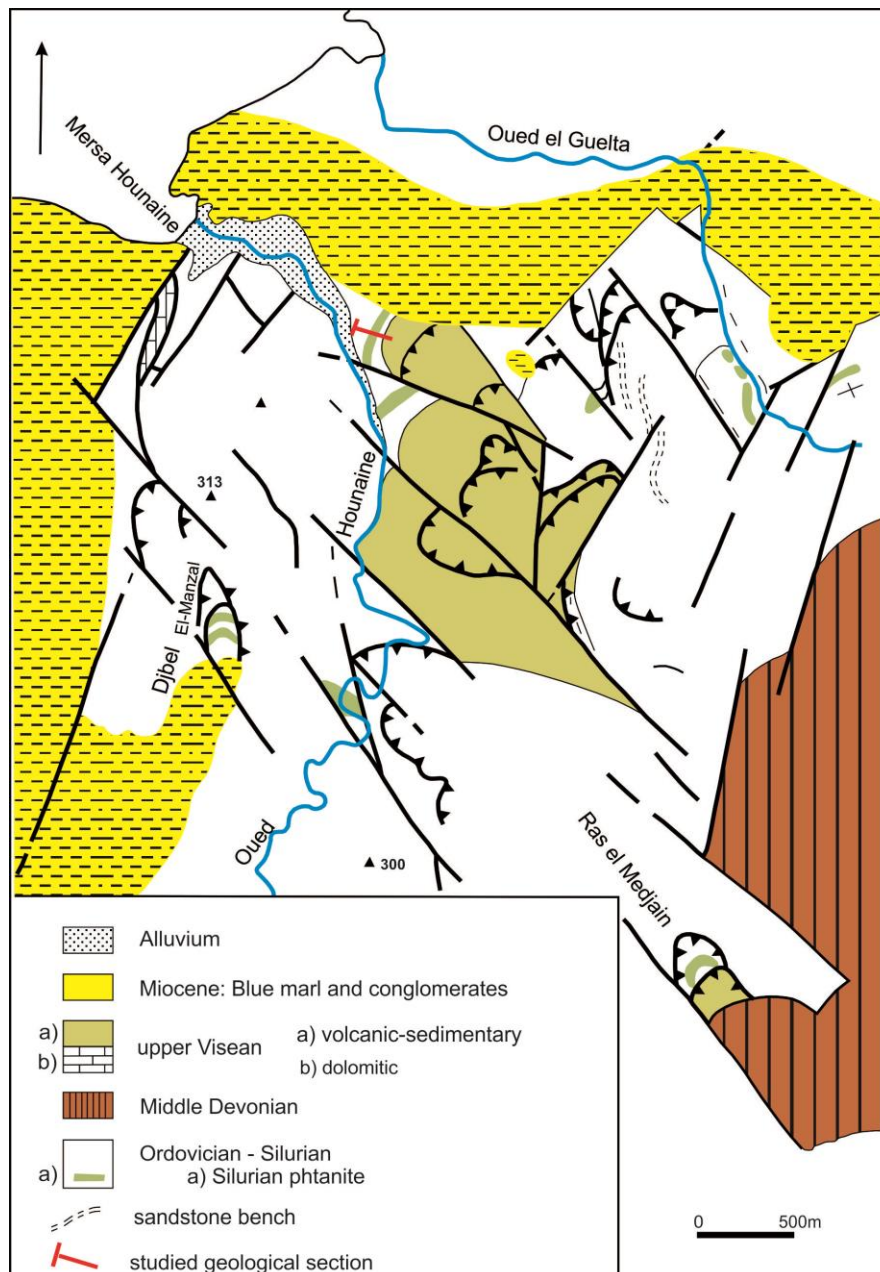
Fig. 3 - Carte géologique simplifiée de la région d'étude (d'après Ciszak 1993)
