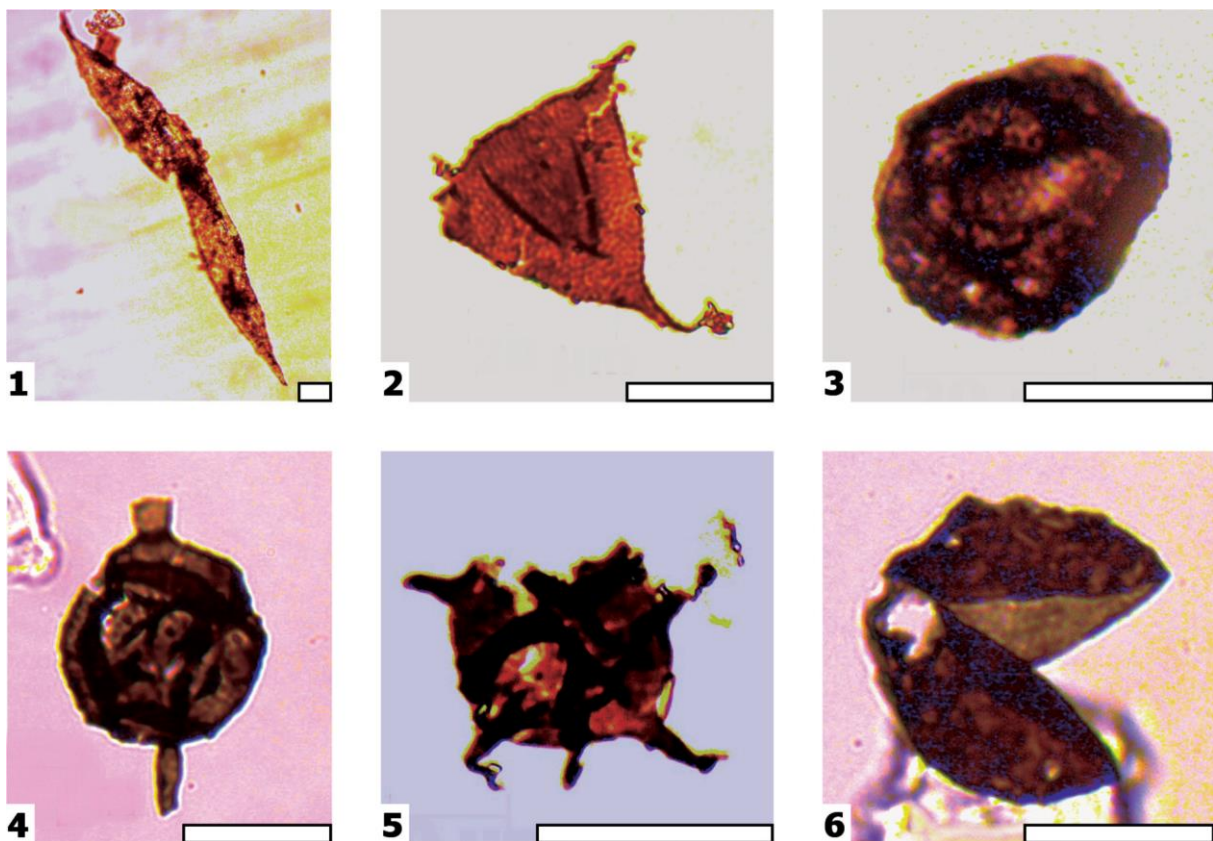
Fig. 6. Microphotographies d'une sélection des acritarches observés
