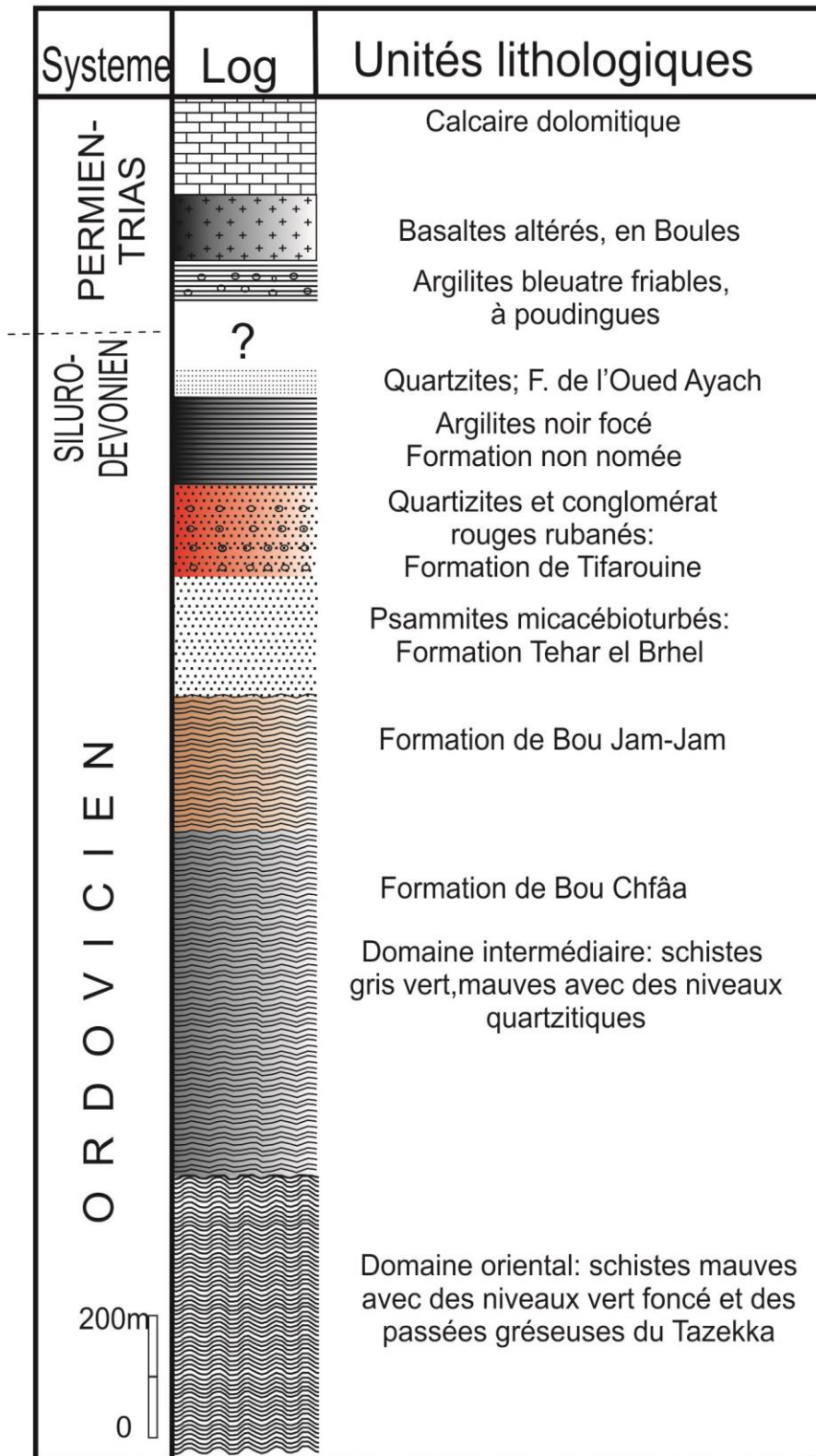
Fig. 4- Coupe lithostratigraphique synthétique des formations paléozoïques constituant le massif de Tazekka (in Chakir 1983)
