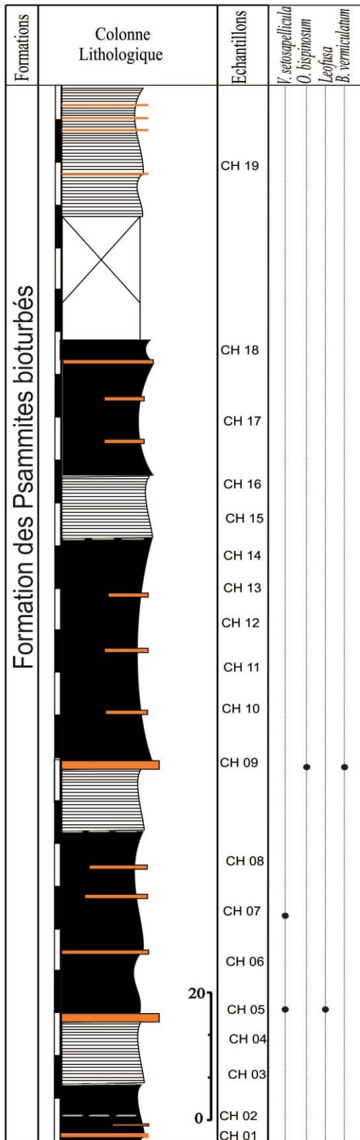
Fig. 4 -Log stratigraphique de la formation des psammites bioturbés, avec la position des échantillons palynologiques et la distribution des taxons d'acritarches identifiés.
