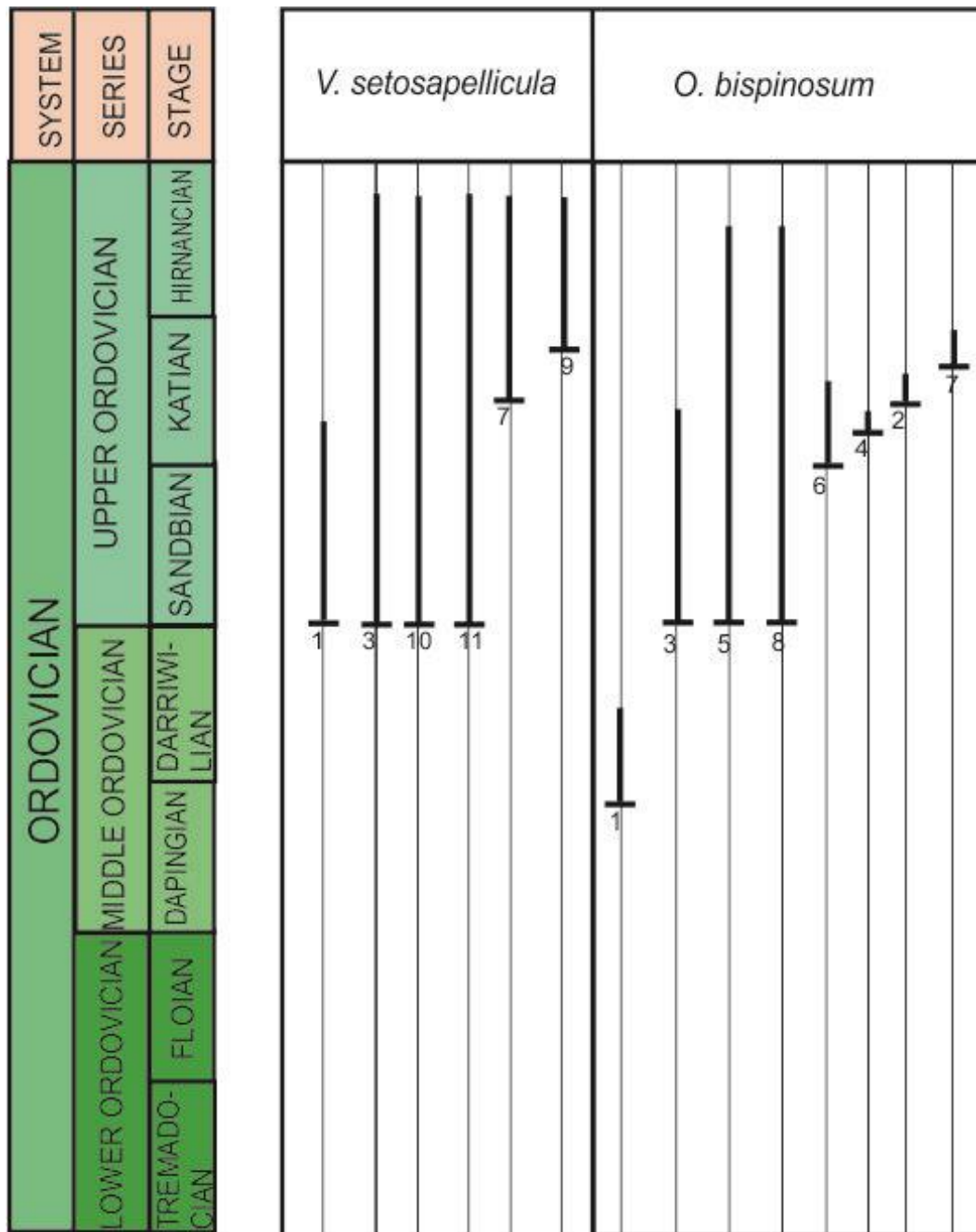
Fig. 5- Répartition stratigraphique globale des espèces V. setosapellicula et O. bispinosum
