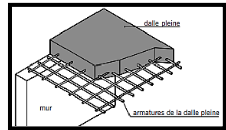
Figure 94. Dalle pleine
