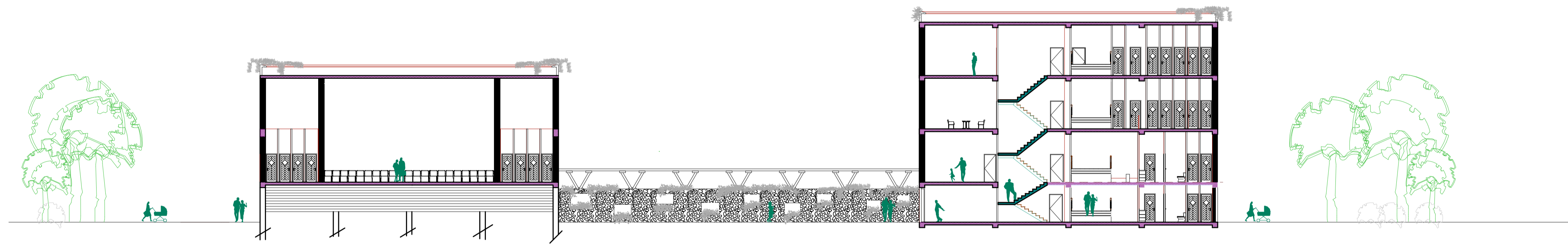
Coupe AA 1/200
