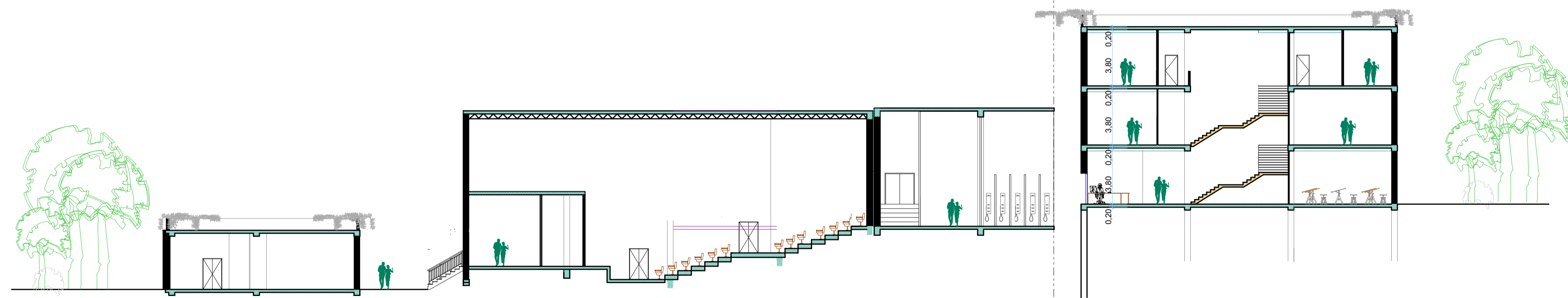
Coupe BB 1/200
